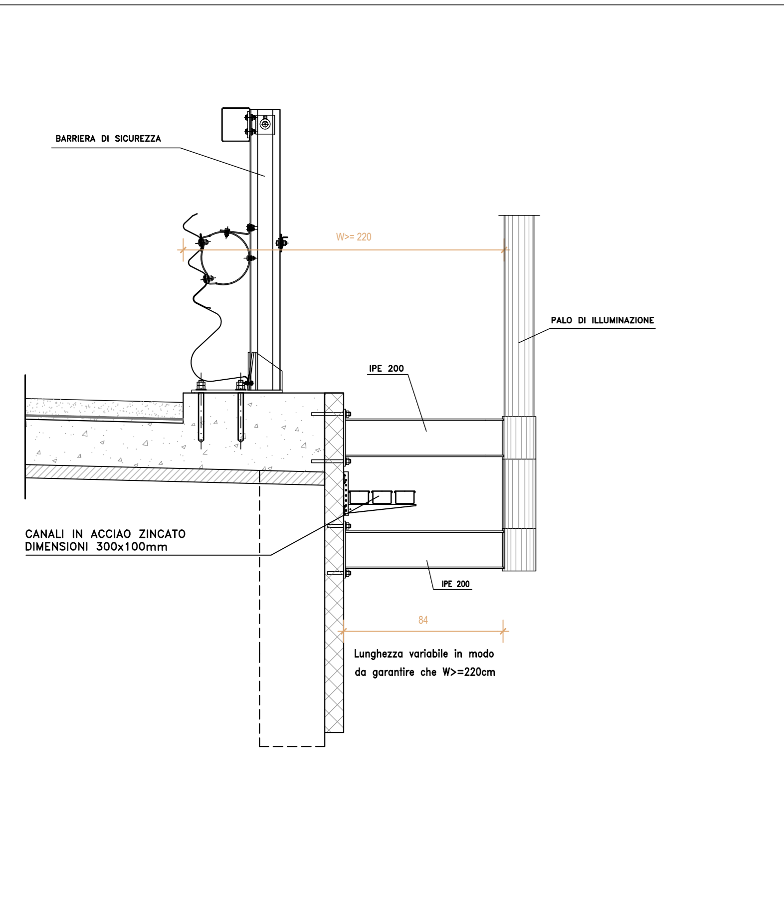
TIPOICO CAVIDOTTI IN CORRISPONDENZA DEI MURI
