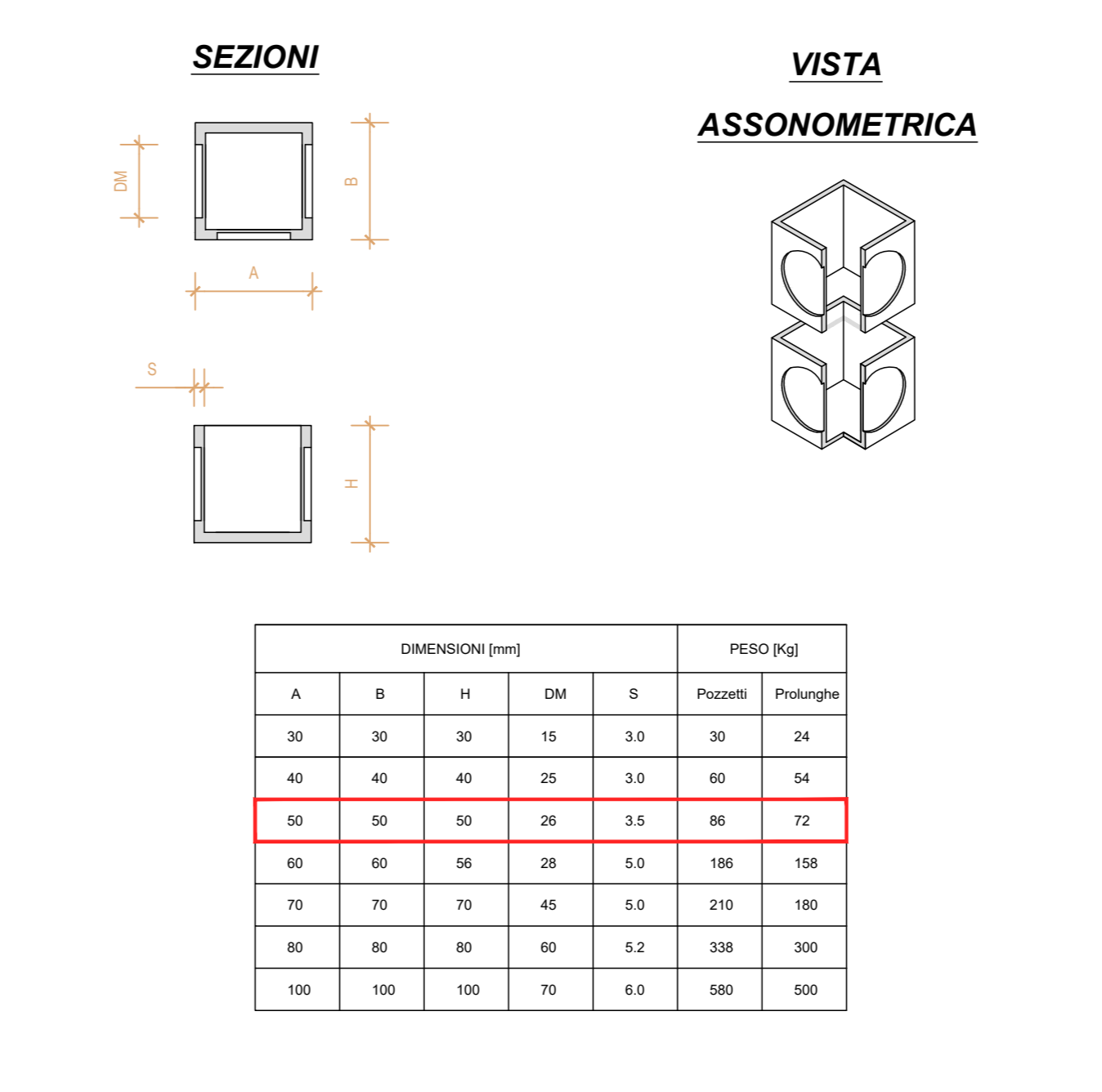
TIPOICO POZZETTO/PROLUNGHE
