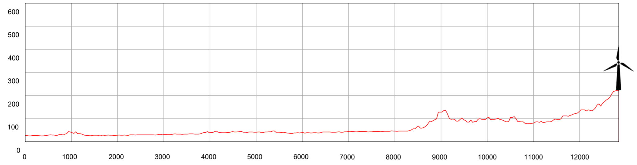
SEZIONE 7A_WTG04
