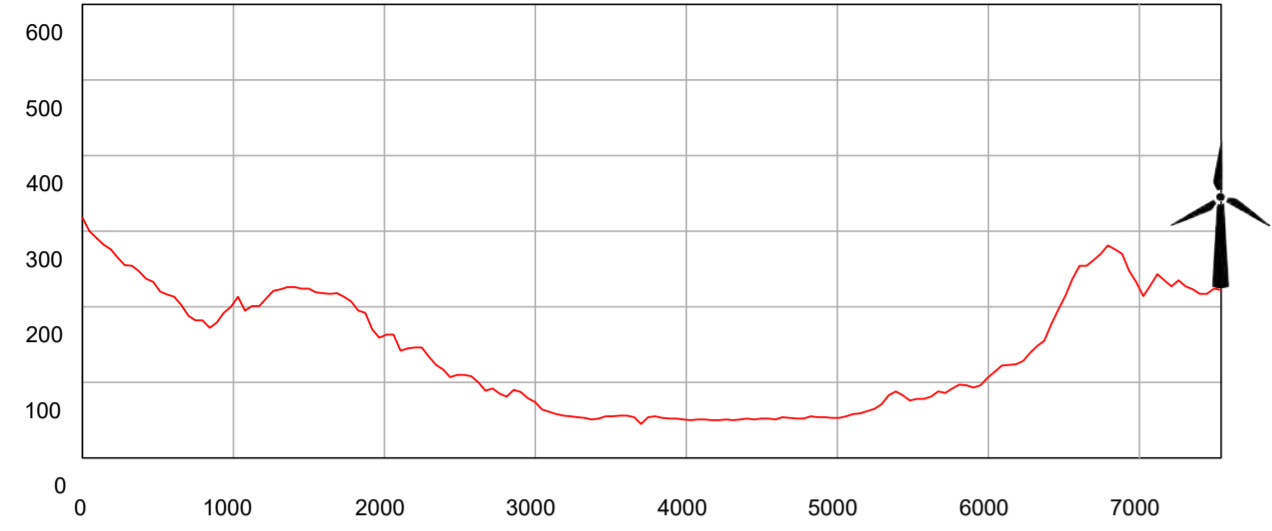
SEZIONE 1_WTG04
