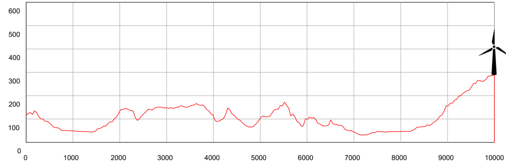
SEZIONE 4B_WTG08
