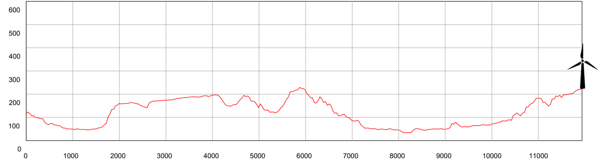
SEZIONE 4B_WTG04
