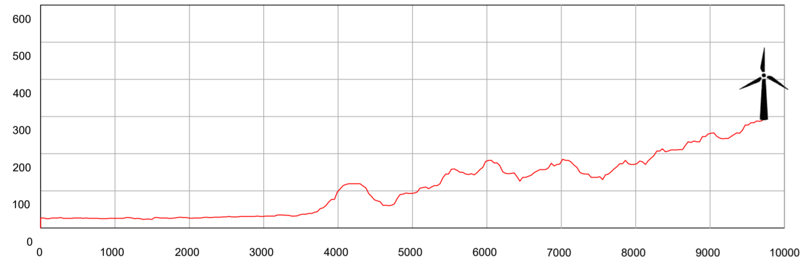
SEZIONE 7A_WTG08
