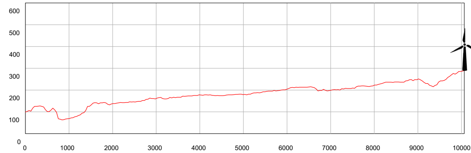
SEZIONE 22_WTG08
