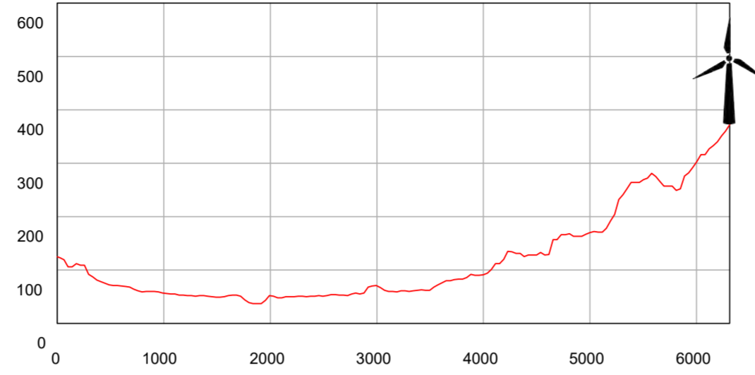
SEZIONE 4B_WTG01
