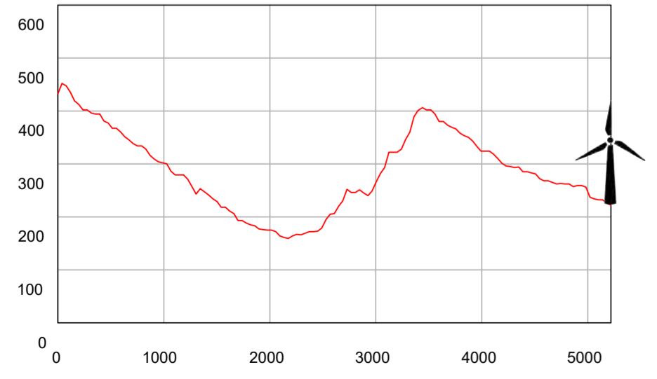
SEZIONE 17_WTG04
