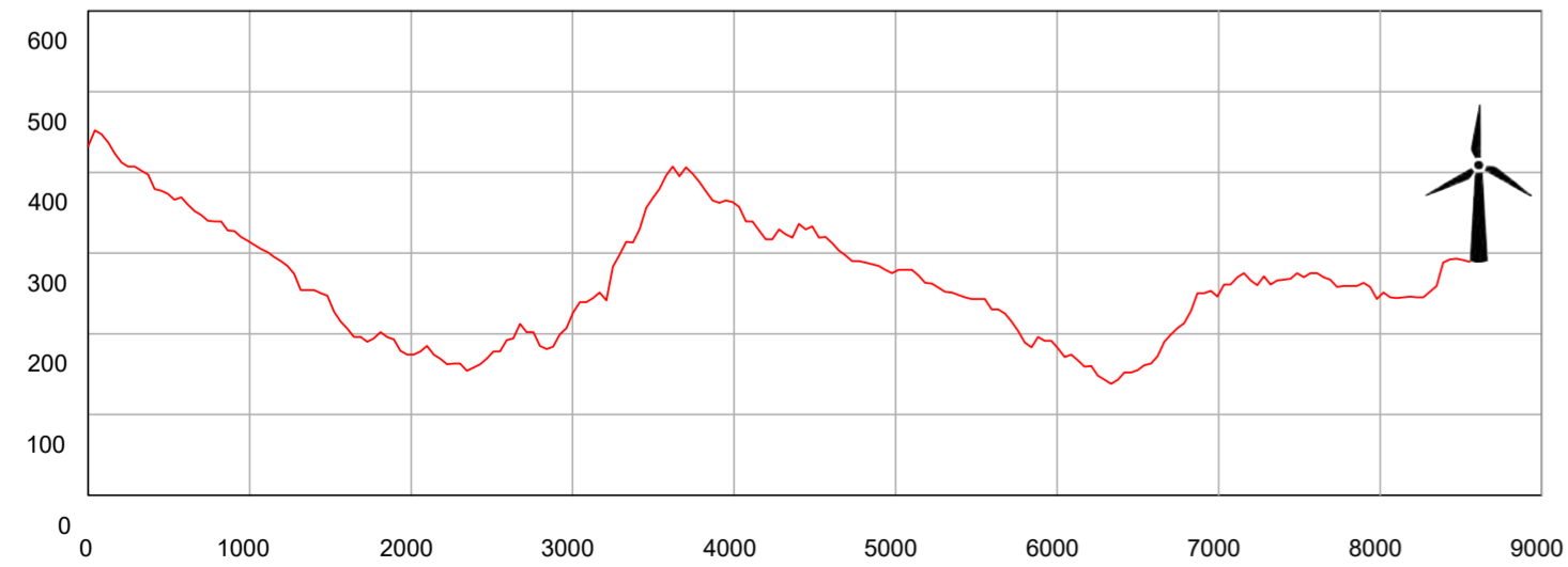
SEZIONE 17_WTG08
