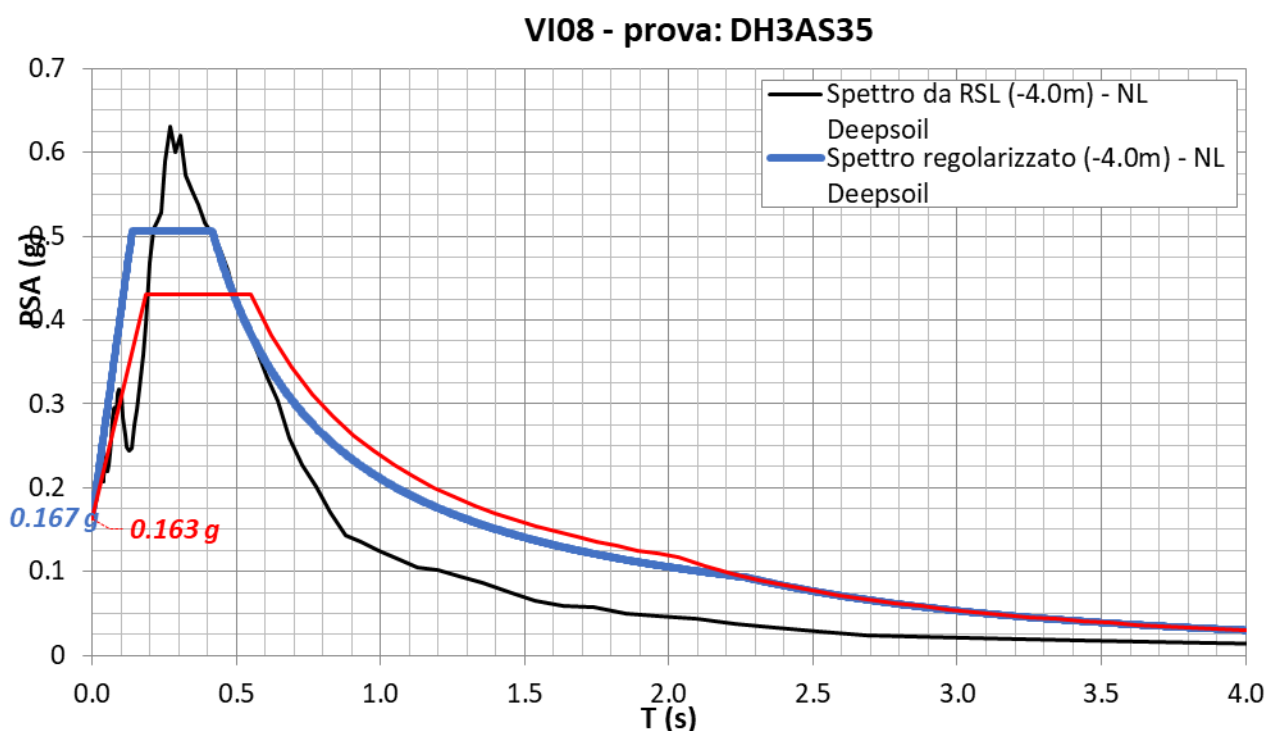
Figura 4-20 - Confronto spettro NTC (rosso) con spettro RSL (blu)
