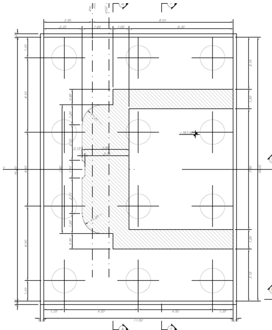
Figura 1-5 - elaborati grafici spalla B (mobile)
