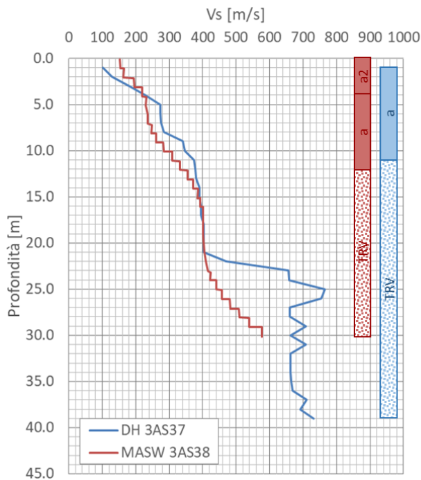
Figura 2 – Indagine sismica eseguita per il viadotto VI09 con relativa stratigrafia: Down Hole 3AS37 ( V_{s,q} = 335 m/s - Suolo tipo C) e la Masw 3AS38 ( V_{s,q} = 314 m/s - Suolo tipo C)
