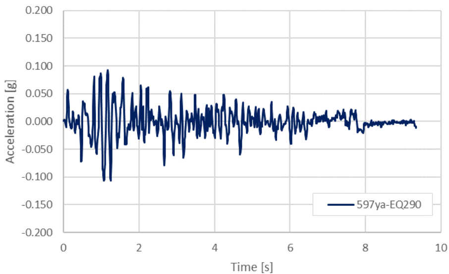
Figura 9 – Accelerogramma naturale: Waveform 597ya – Eartquake 290
