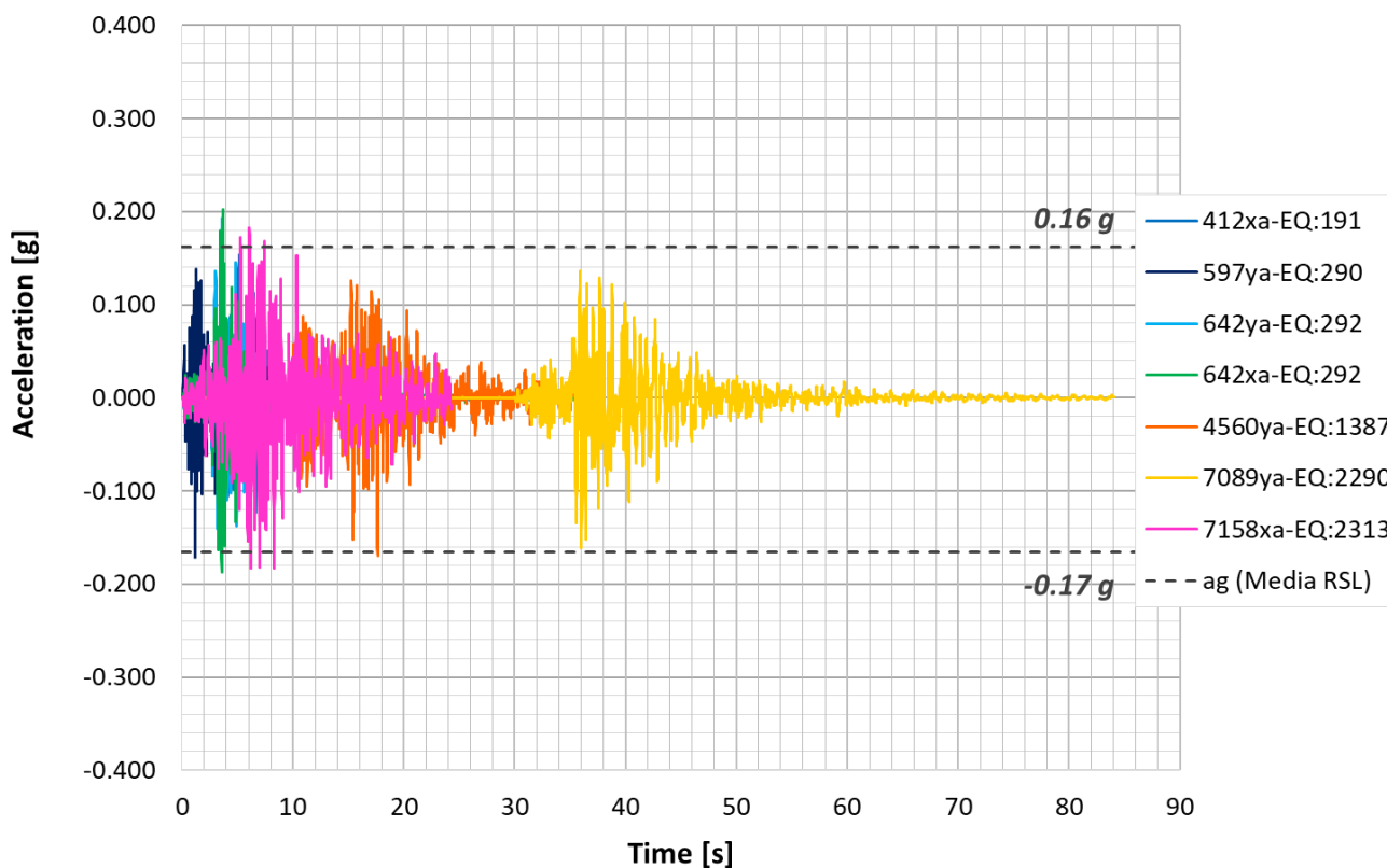
Figura 18 – Risposta Sismica Locale per SLV di L3B – VI09: Accelerogrammi a 4,0 m di profondità
