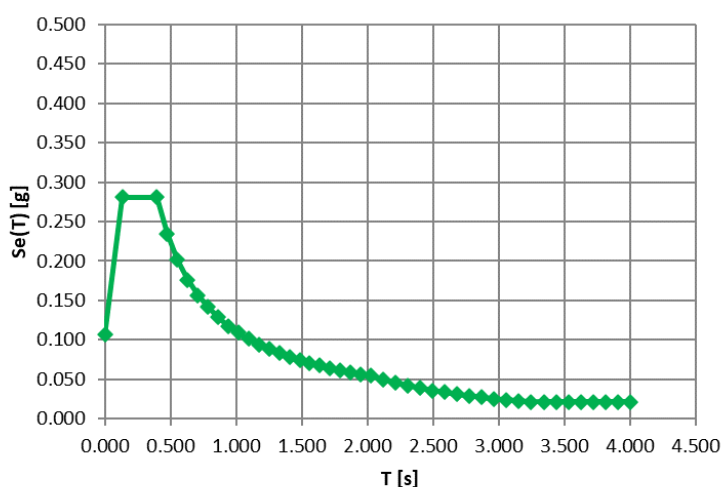
Figura 4 - VI-09 Stato Limite di Salvaguardia della Vita: Spettro di risposta elastico in accelerazione, classe di sottosuolo A, categoria topografica T_1 , V_N = 75 anni e C_U di tipo III (NTC 2018)
