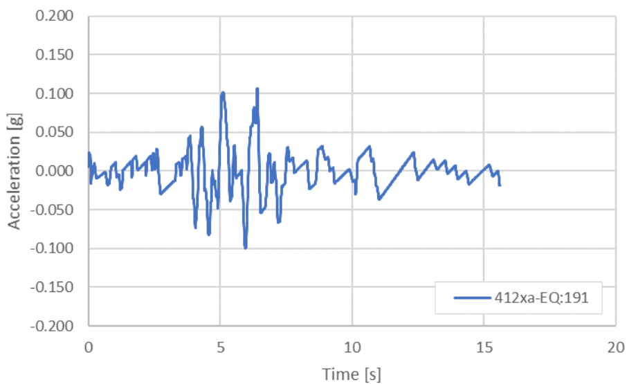
Figura 8 – Accelerogramma naturale: 412xa – Eartquake 191
