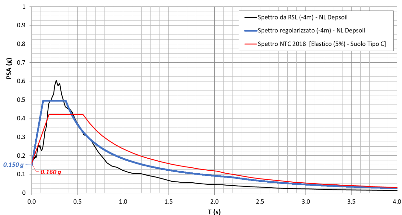
Figura 19 – Risposta Sismica Locale per SLV di L3B – VI09: confronto tra spettro di RSL e spettro di normativa
