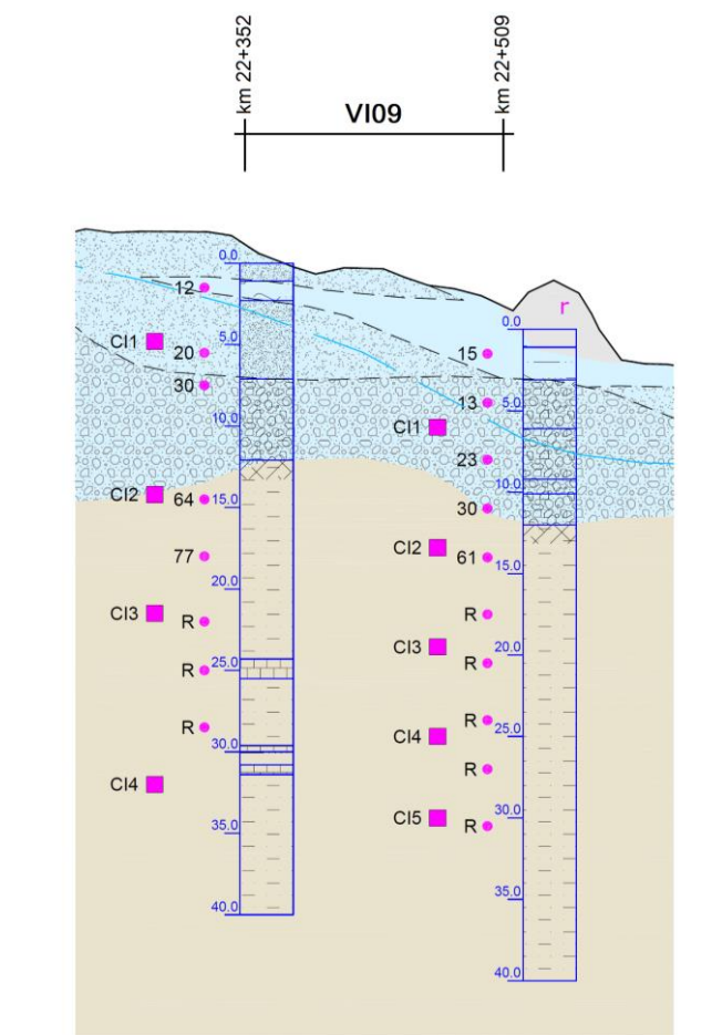
Figura 1: Profilo stratigrafico relativo al viadotto VI09
