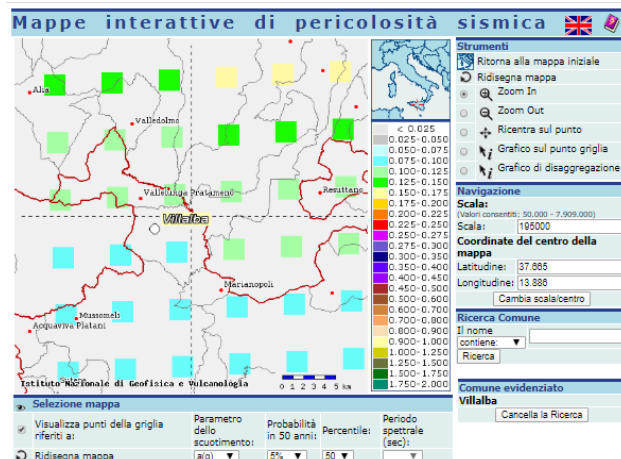
Figura 5 - VI09: Mappa di pericolosità sismica
