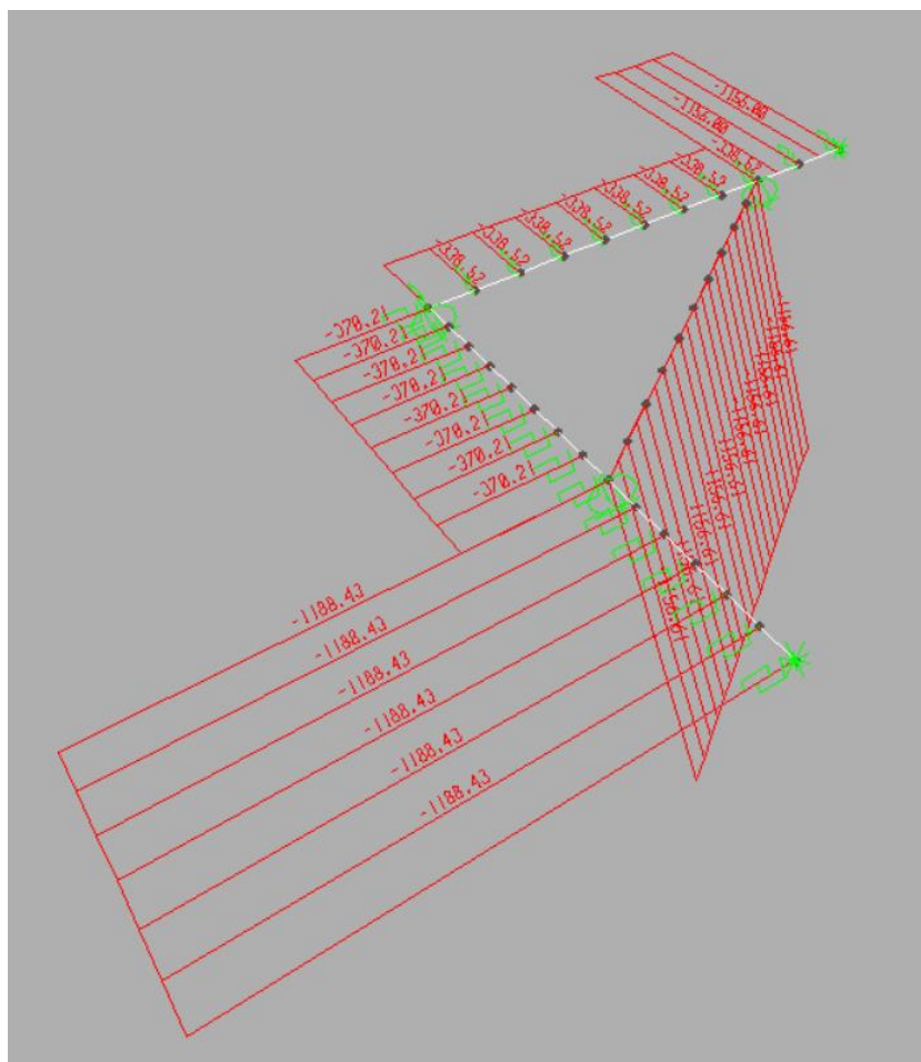
Figura 10: forza assiale allo SLU-STR
