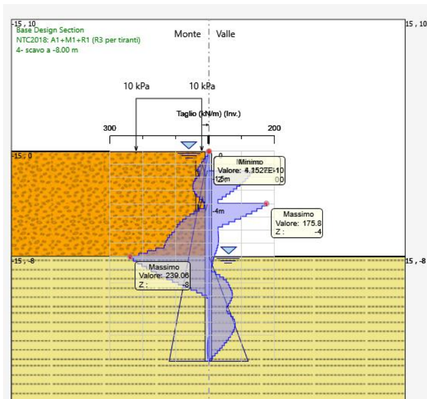
Figura 8: forza di taglio allo SLU-STR
