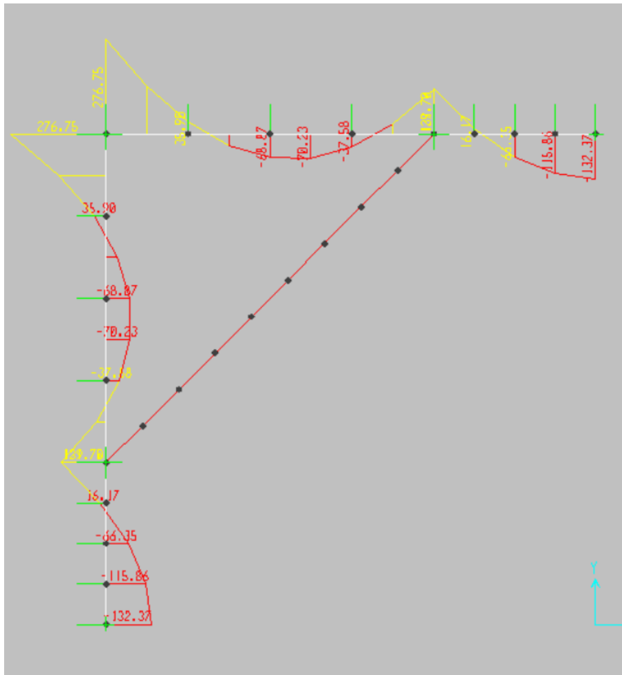
Figura 4: momento flettente allo SLU-STR
