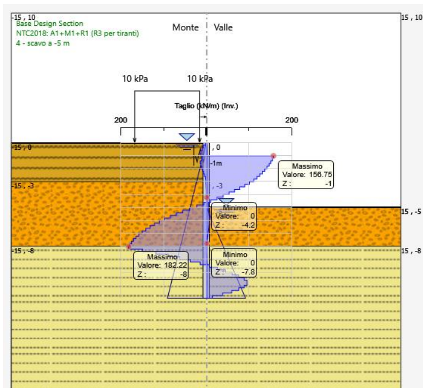
Figura 13: forza di taglio allo SLU-STR
