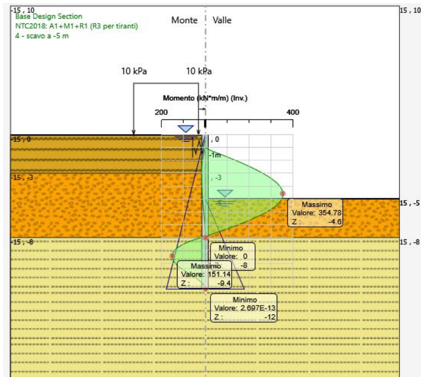
Figura 12: momento flettente allo SLU-STR
