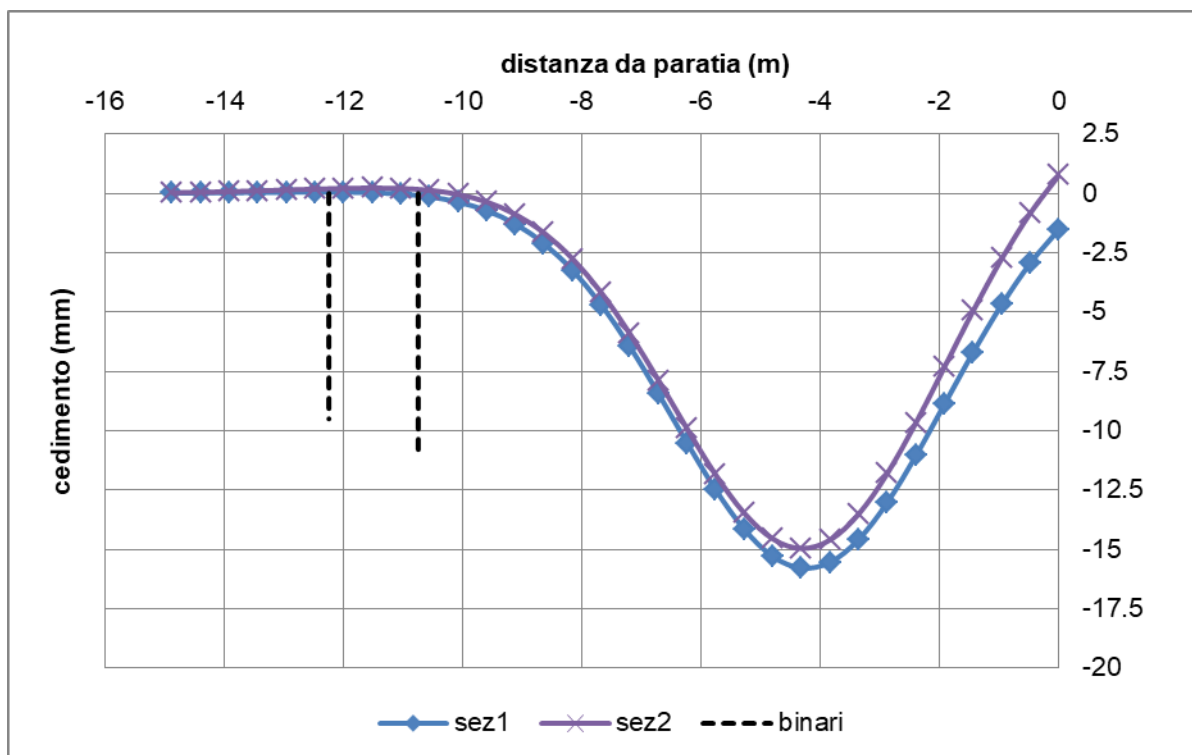
Figura 15: Curva dei cedimenti a tergo paratia
