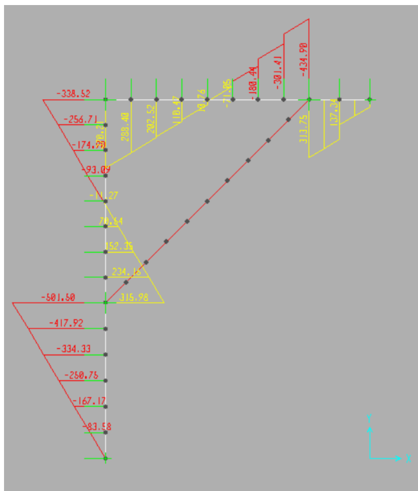
Figura 11: forza di taglio allo SLU-STR
