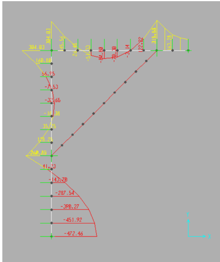
Figura 9: momento flettente allo SLU-STR
