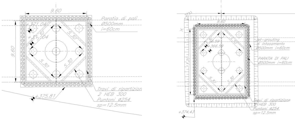
Figura 1: planimetria di scavo tipo con indicazione delle opere di sostegno
