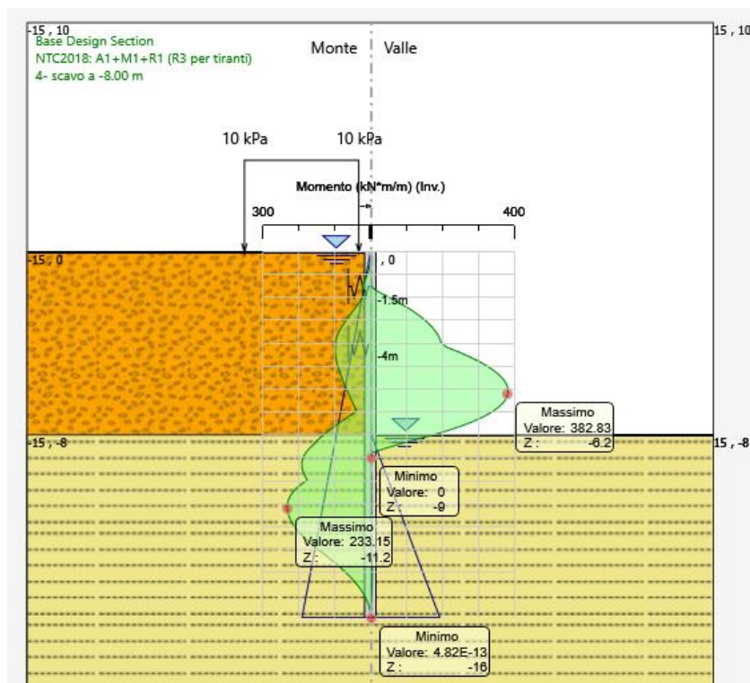
Figura 7: momento flettente allo SLU-STR
