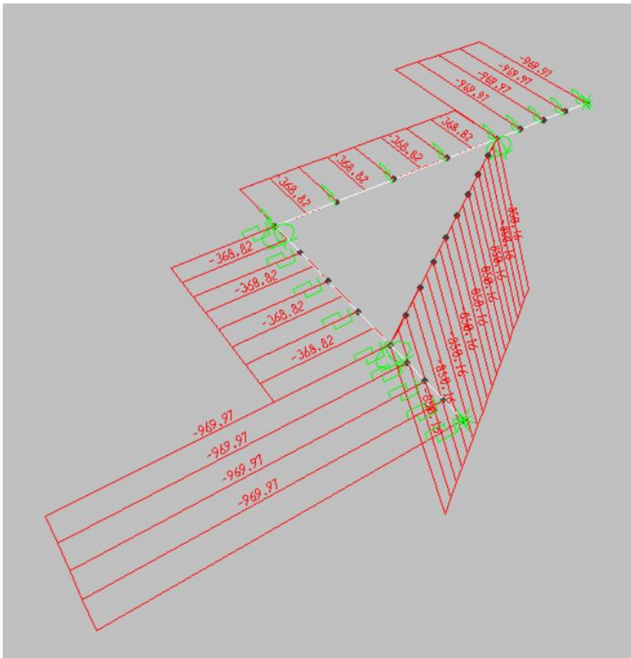
Figura 5: forza assiale allo SLU-STR
