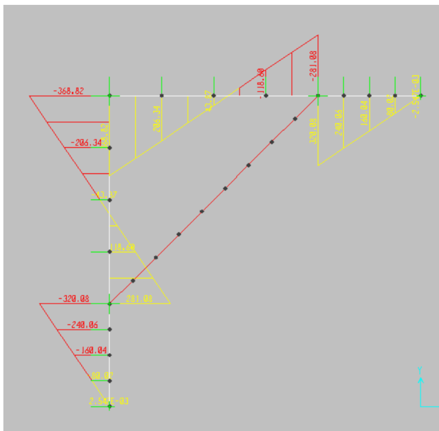
Figura 6: forza di taglio allo SLU-STR
