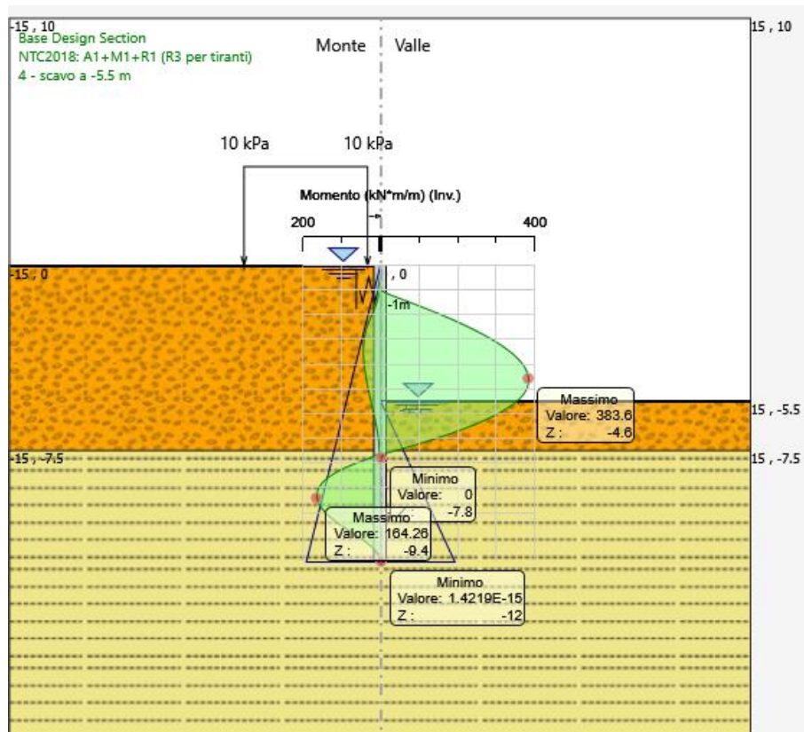
Figura 2: momento flettente allo SLU-STR
