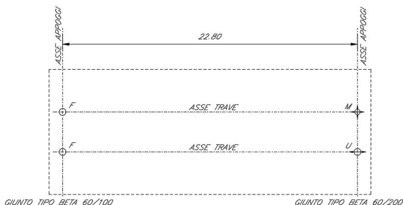
Figura 1-1-1: schema appoggi
