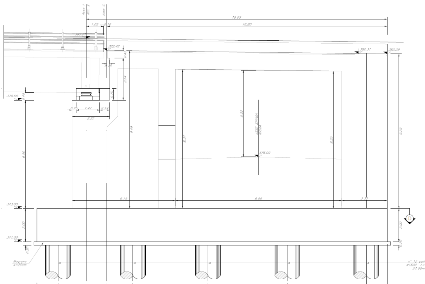
Figura 4-25 – Dettaglio spalla B
