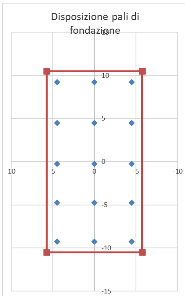
Figura 4-24 - disposizione dei pali di fondazione
