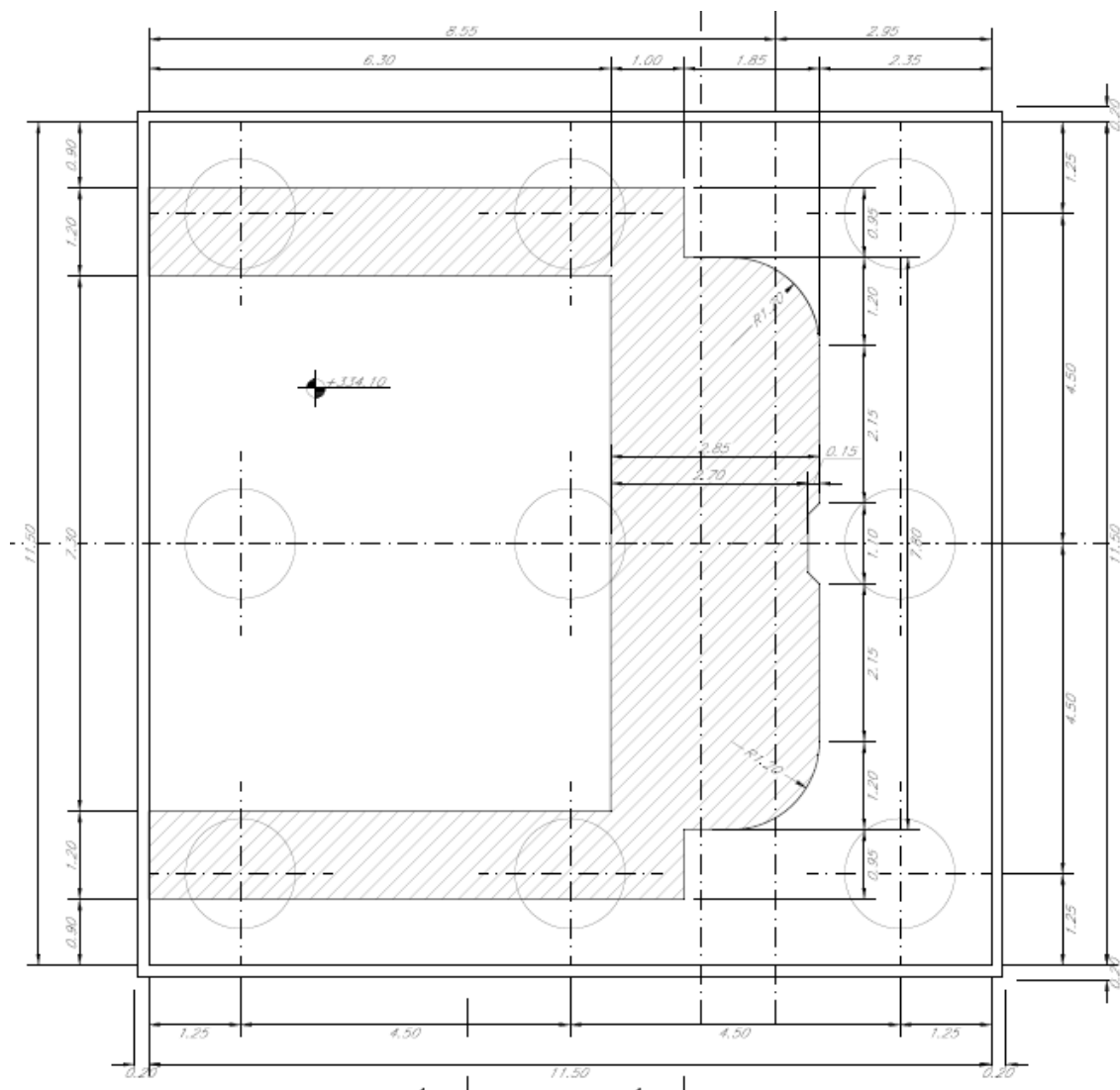
Figura 1-4: elaborati grafici spalla A (mobile)
