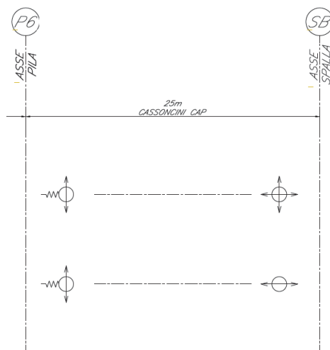
Figura 1-1-1: schema appoggi
