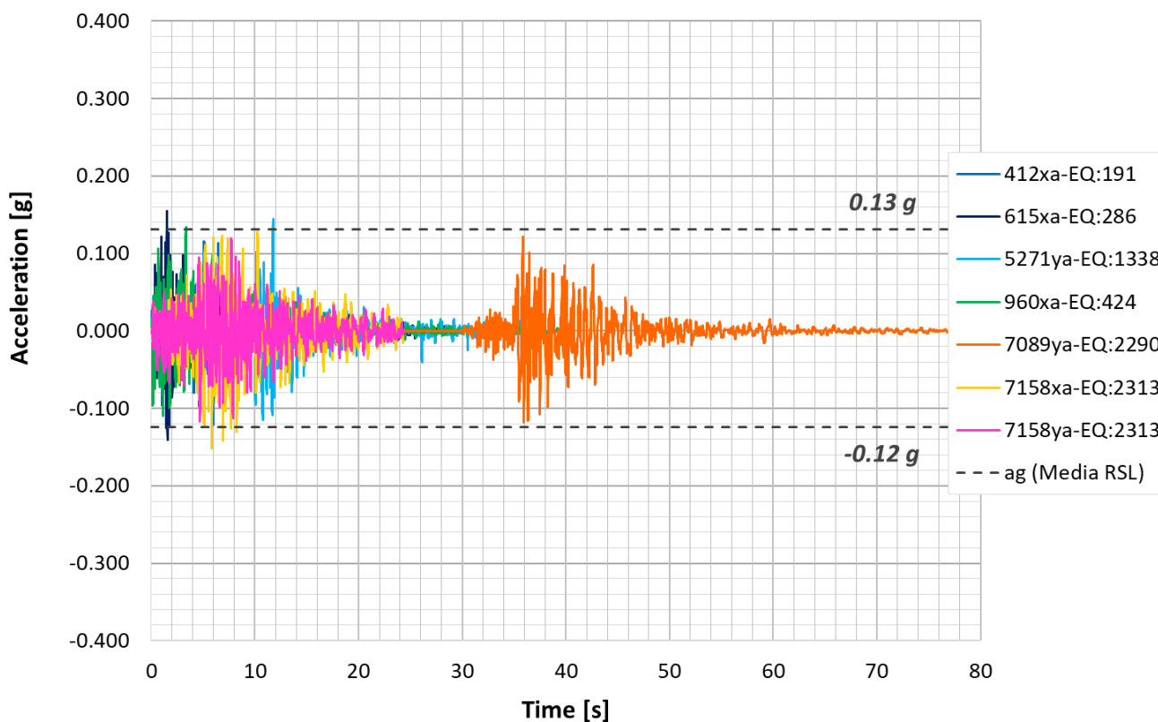
Figura 18 – Risposta Sismica Locale per SLV di L3B – VII3: Accelerogrammi a 4,0 m di profondità
