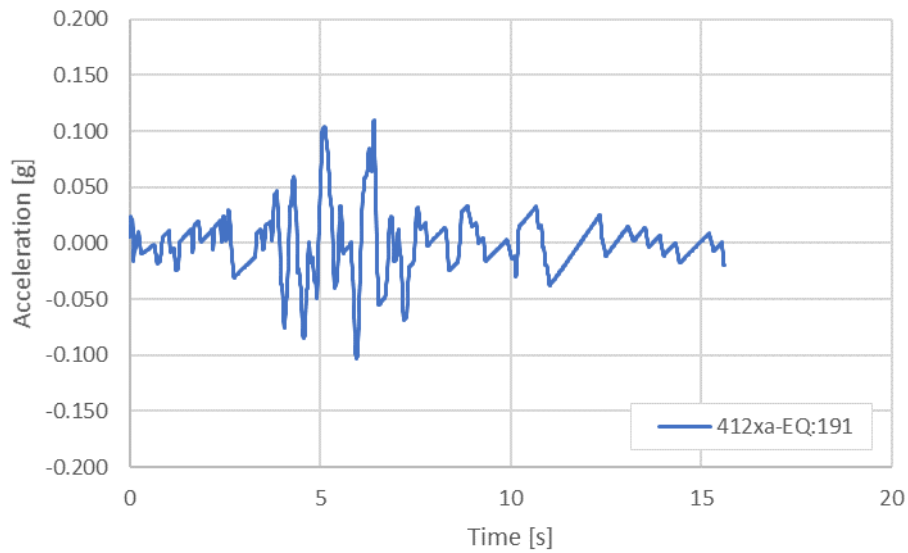
Figura 8 – Accelerogramma naturale: Waveform 412xa – Eartquake 191
