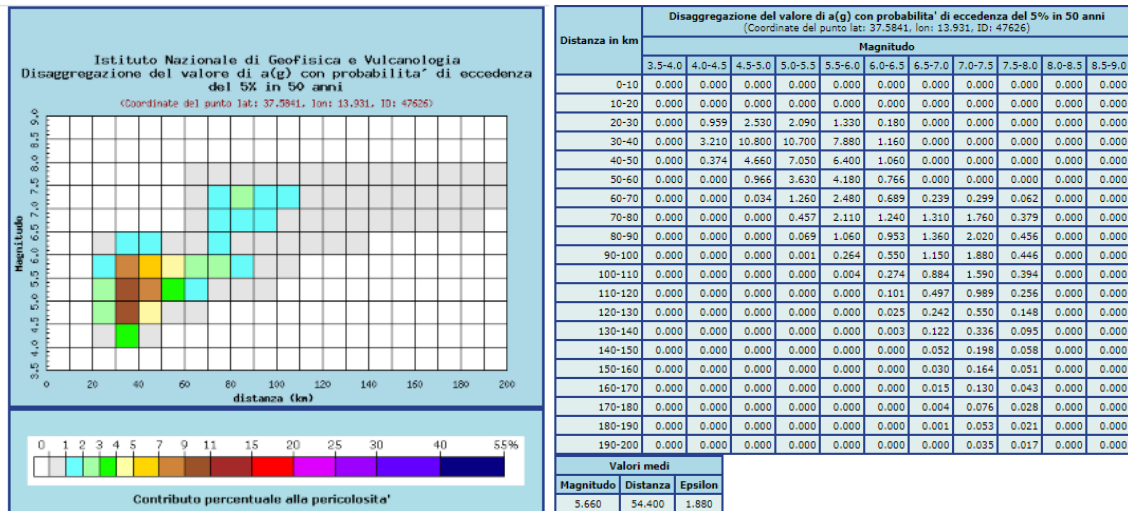
Figura 6 – VII3: Magnitudo e distanza
