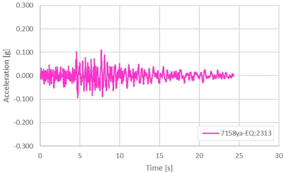
Figura 14 – Accelerogramma naturale: Waveform 7158ya – Eartquake 2313
