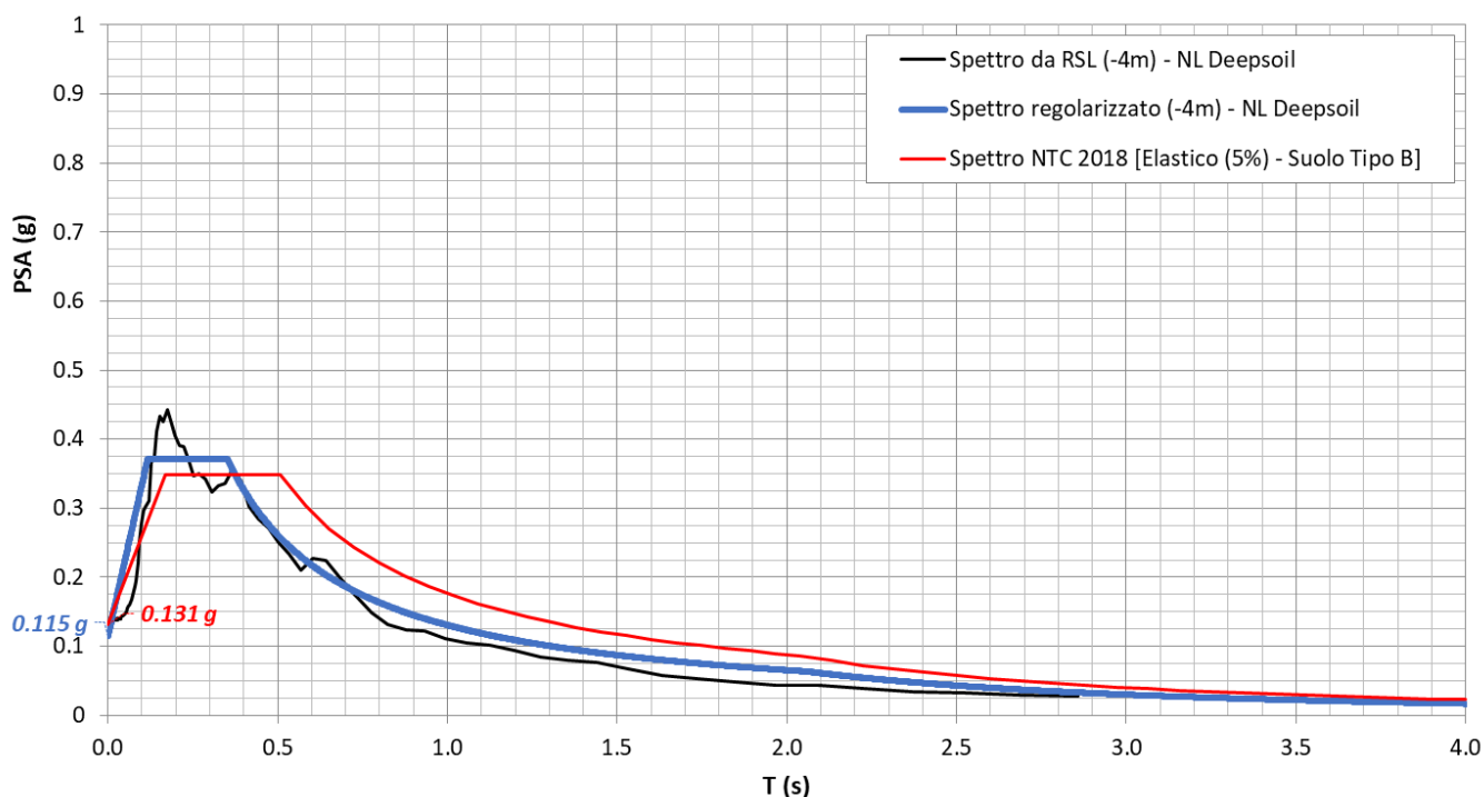
Figura 19 – Risposta Sismica Locale per SLV di L3B – VI13: confronto tra spettro di RSL e spettro di normativa
