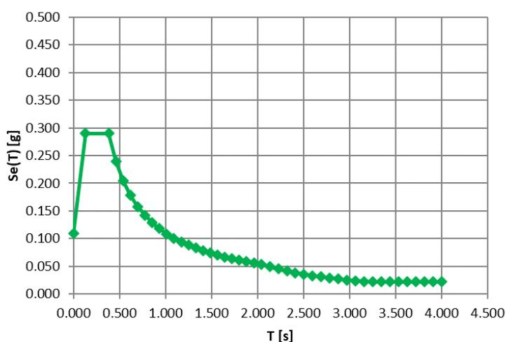
Figura 4 - VI13 Stato Limite di Salvaguardia della Vita: Spettro di risposta elastica in accelerazione, classe di sottosuolo A, categoria topografica T_1 , V_N = 75 anni e C_U di tipo III (NTC 2018)
