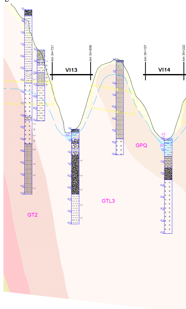
Figura 1: Profilo stratigrafico relativo al viadotto VI13
