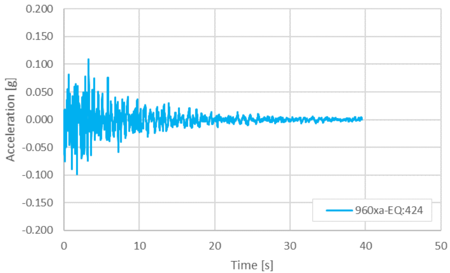
Figura 10 – Accelerogramma naturale: Waveform 960xa – Eartquake 424
