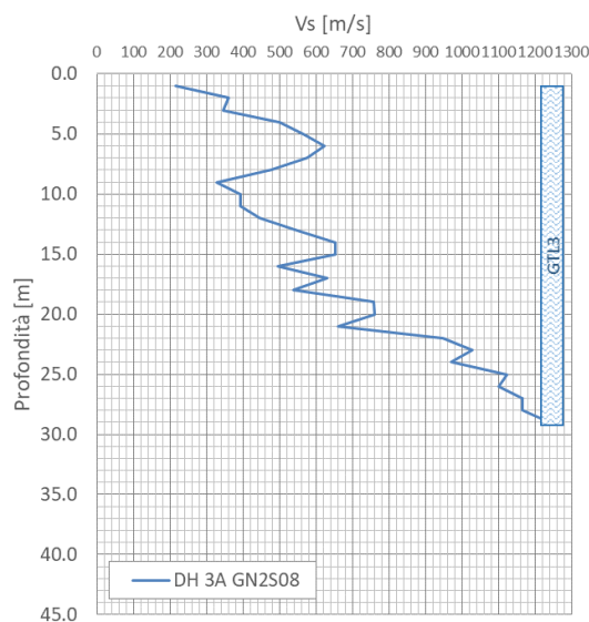
Figura 2 – Prova sismica in foro eseguita per il viadotto VI12 con relativa stratigrafia: la DOWN HOLE 3AGN2S08 ( V_{s,q} = 540 m/s - Suolo tipo B)
