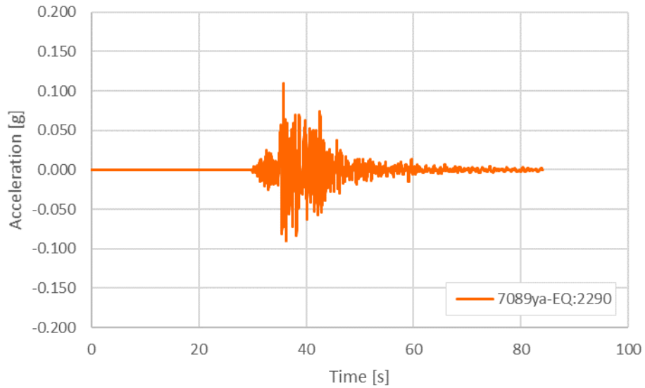
Figura 12 – Accelerogramma naturale: Waveform 7089ya – Eartquake 2290
