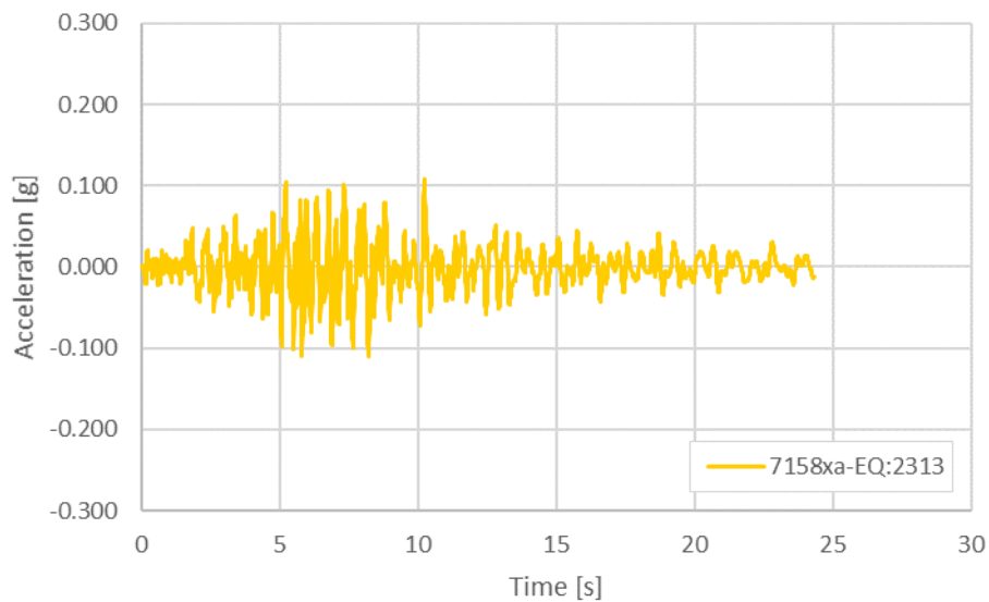
Figura 13 – Accelerogramma naturale: Waveform 7158xa – Eartquake 2313
