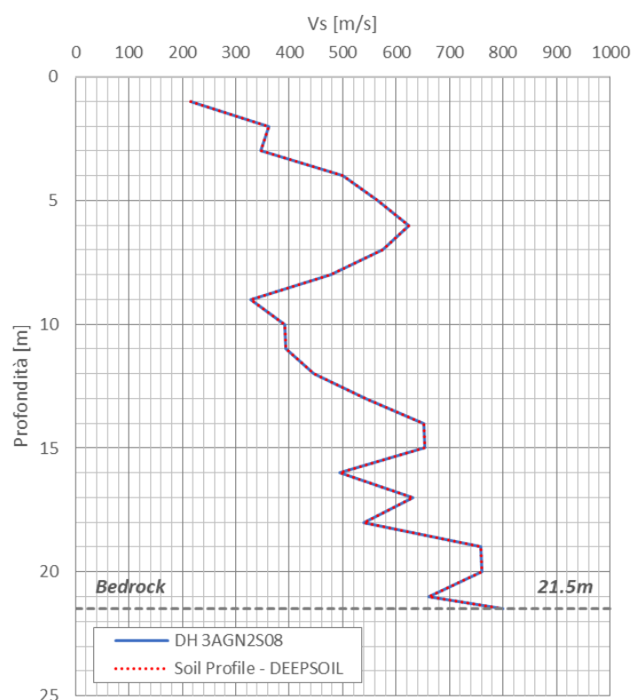
Figura 17 – Soil Profile adottato
