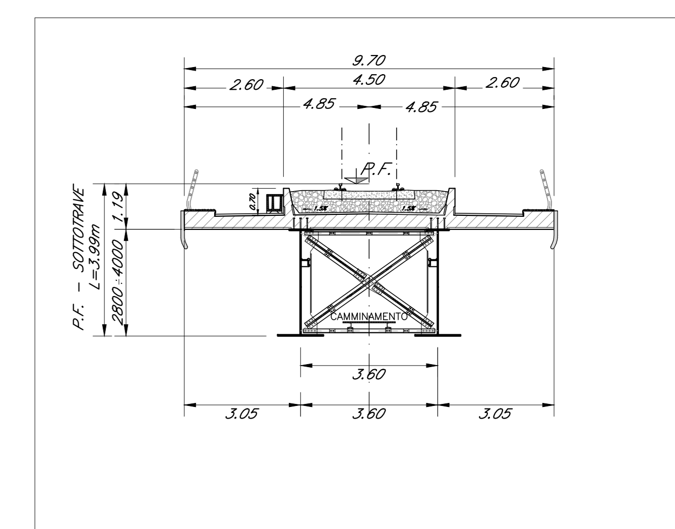
SEZIONE TIPO ACCIAIO 50m Scala 1:100
