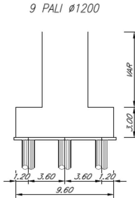
Figura 2 stralcio del profilo longitudinale
