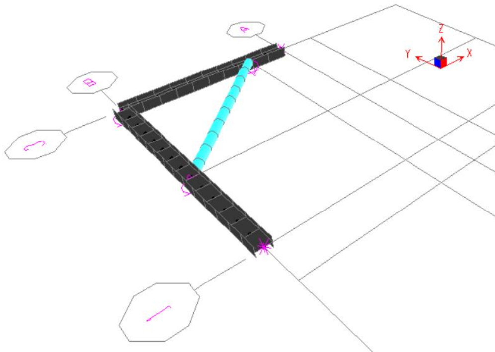
Figura 11: schema statico utilizzato nel codice di calcolo SAP2000 per la valutazione della rigidezza da assegnare al sistema di controventamento della paratia
