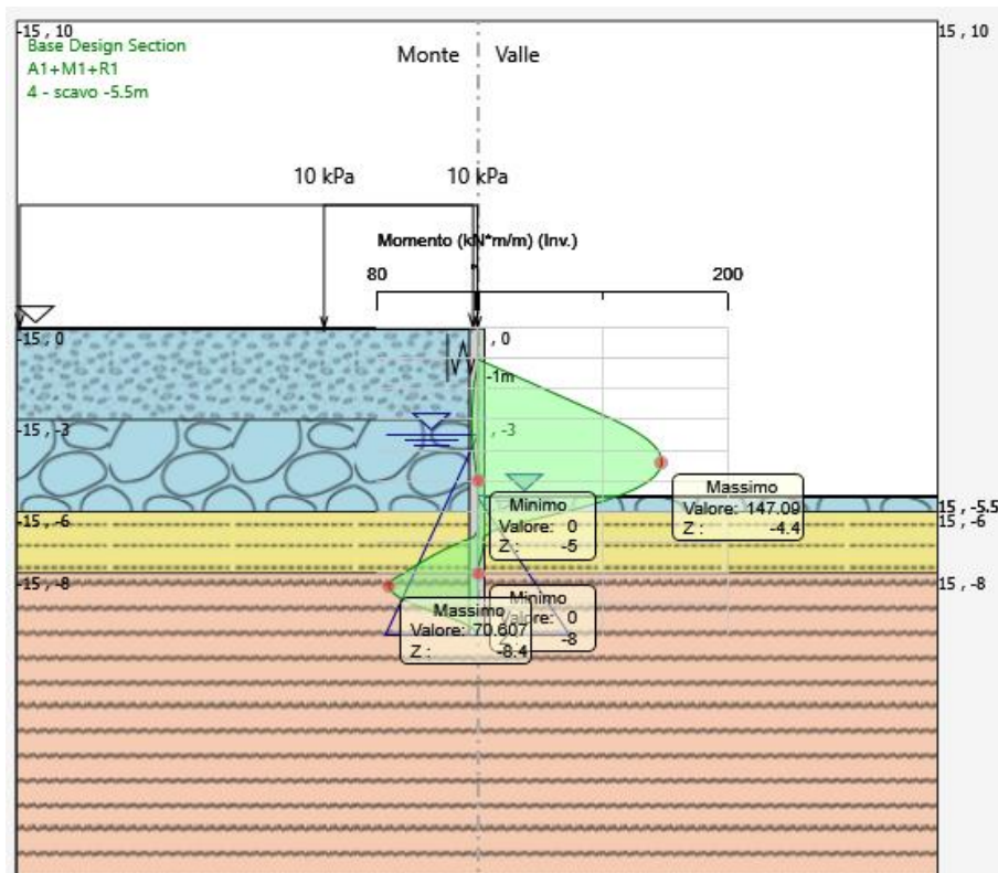
Figura 6: momento flettente allo SLU-STR
