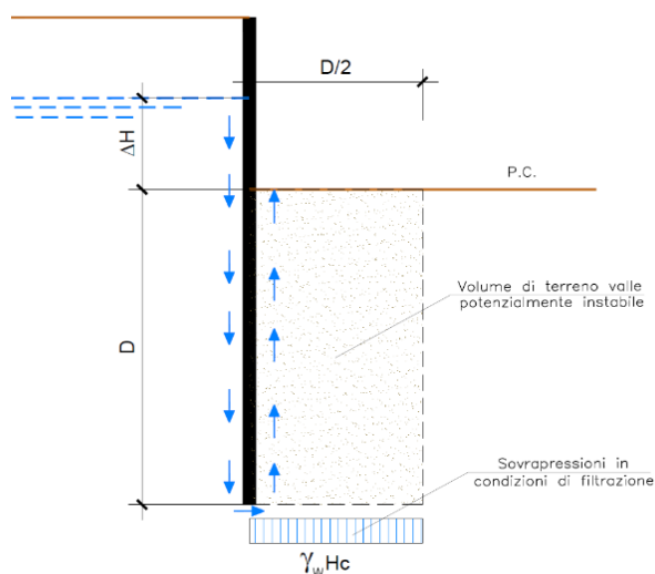
Figura 14: Schema di filtrazione per effetto di scavi sotto falda a valle di opere di sostegno
