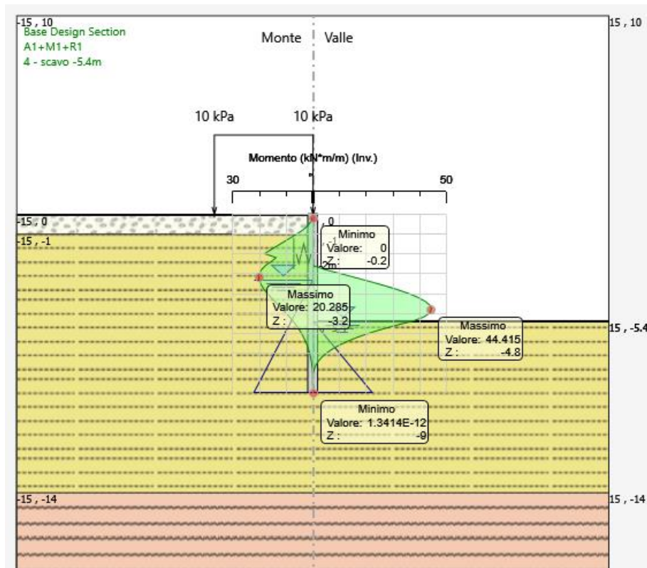
Figura 12: momento flettente allo SLU-STR
