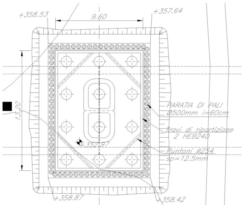
Figura 1: planimetria di scavo tipo con indicazione delle opere di sostegno
