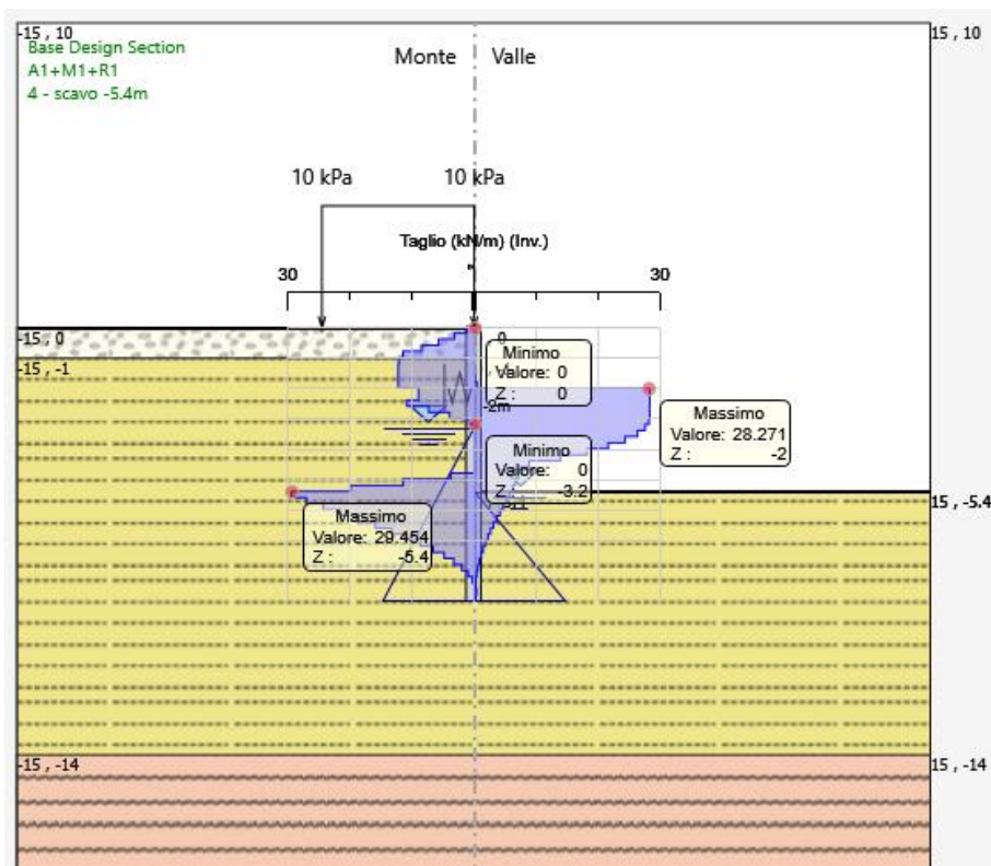
Figura 13: forza di taglio allo SLU-STR
