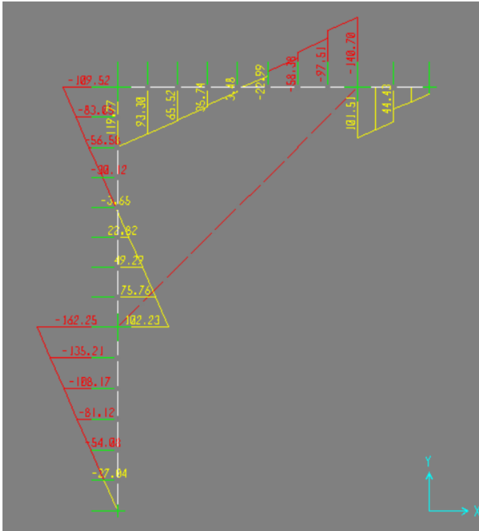
Figura 10: forza di taglio allo SLU-STR
