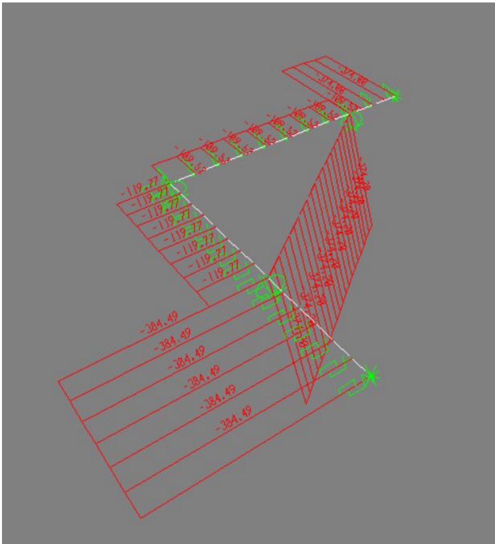
Figura 9: forza assiale allo SLU-STR
