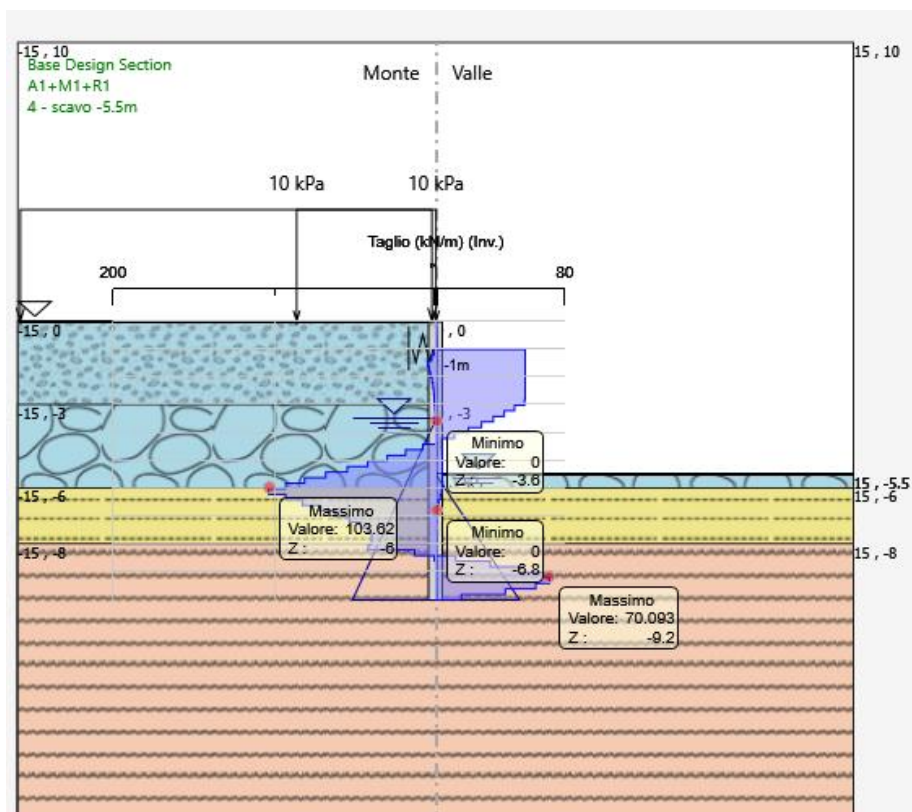
Figura 7: forza di taglio allo SLU-STR
