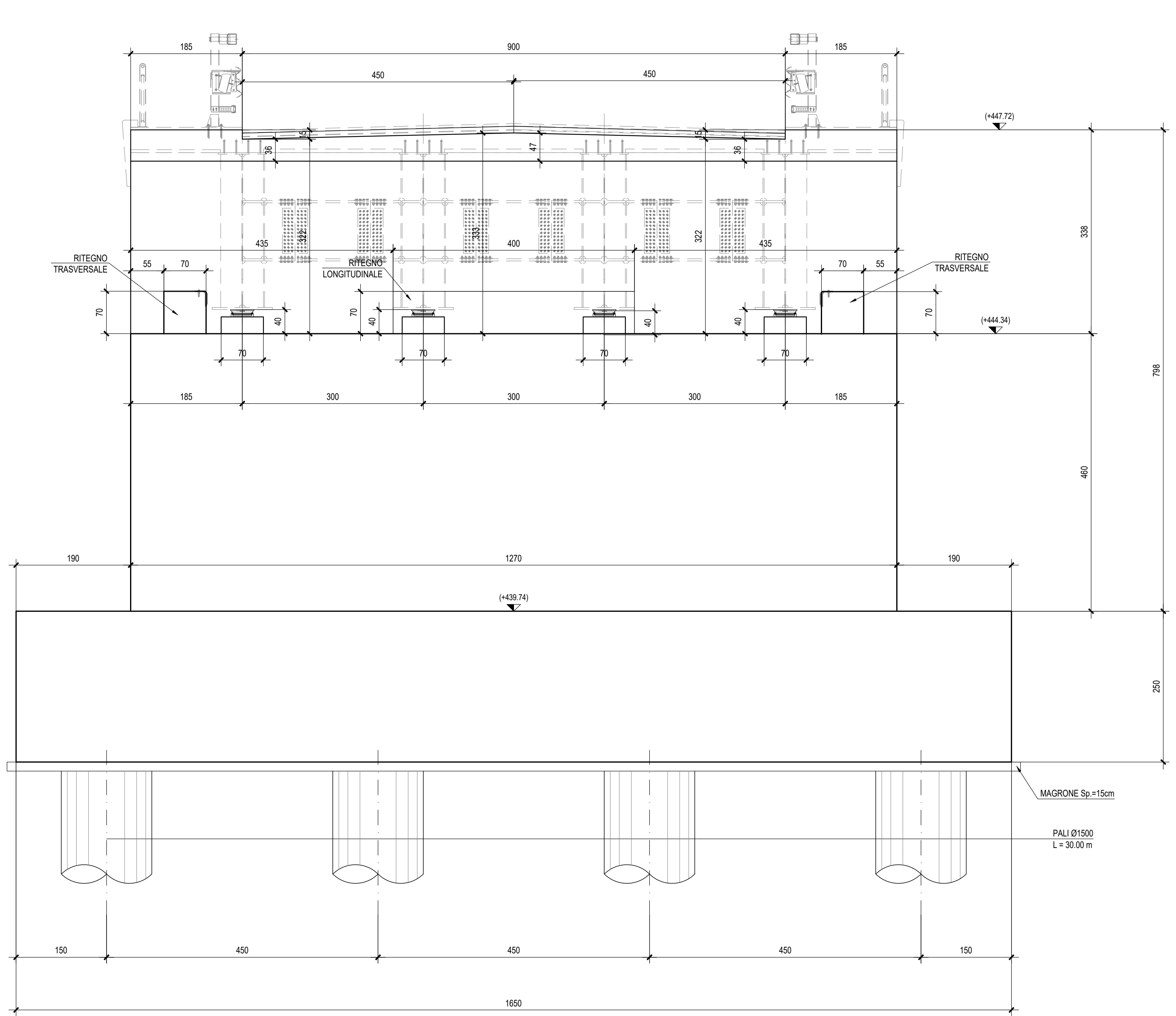
VISTA A-A - Scala 1:50
