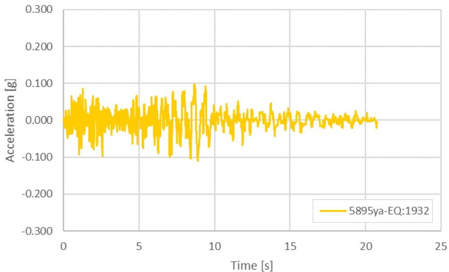
Figura 13 – Accelerogramma naturale: Waveform 5895ya – Eartquake 1932
