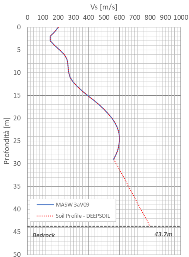
Figura 17 – Soil Profile adottato
