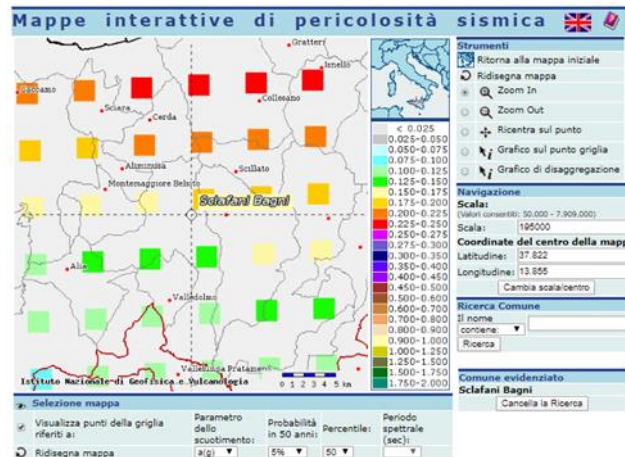
Figura 5 - IV01 (NV07): Mappa di pericolosità sismica
