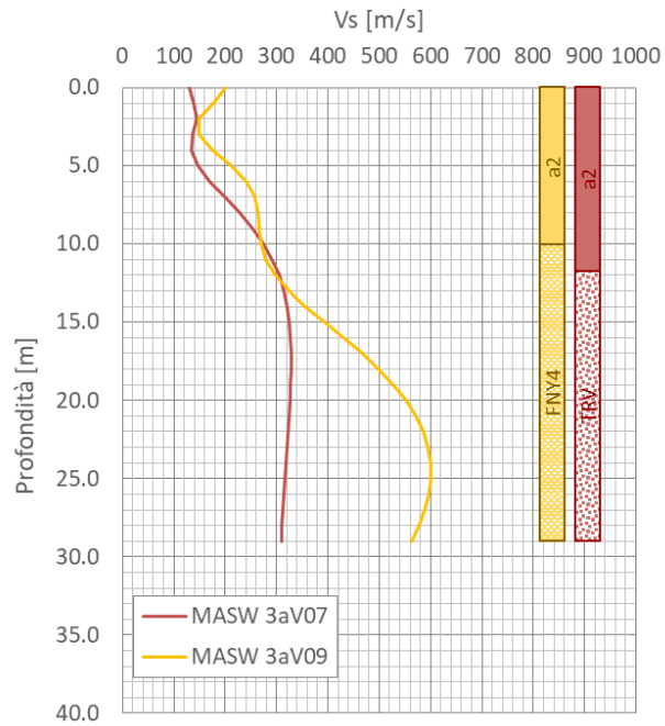
Figura 2 – Indagine sismica eseguita per il viadotto IV01 (NV07) con relativa stratigrafia: MASW 3AV07 ( V_s, q = 238 m/s – Suolo tipo C) e la MASW 3AV09 ( V_s, q = 317 m/s – Suolo tipo C)
