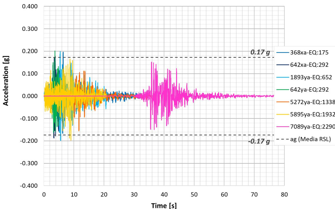
Figura 18 – Risposta Sismica Locale per SLV di L3A - IV01 (NV07): Accelerogrammi a 4,0 m di profondità
