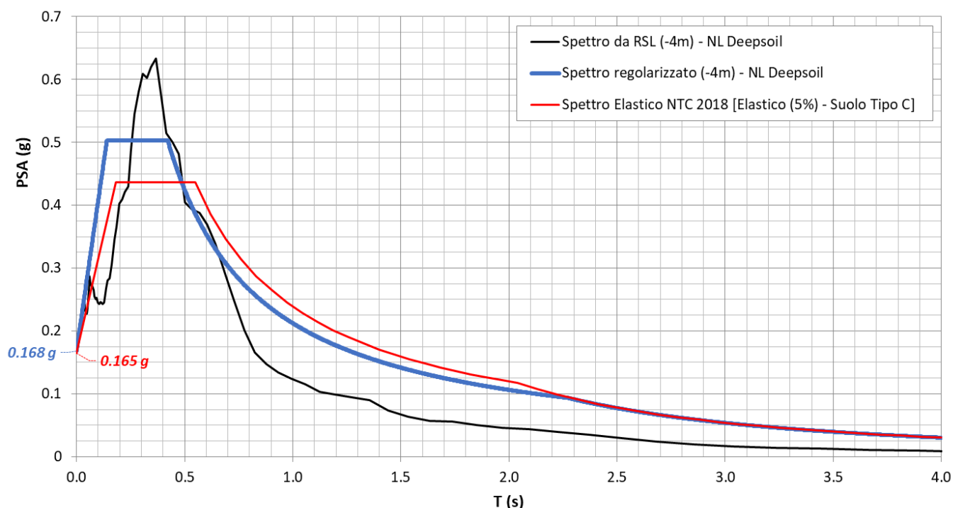
Figura 19 – Risposta Sismica Locale per SLV di L3A – IV01 (NV07): confronto tra spettro di RSL e spettro di normativa
