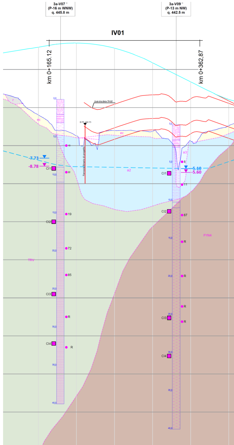
Figura 1: Profilo stratigrafico relativo al viadotto IV01 (NV07)
