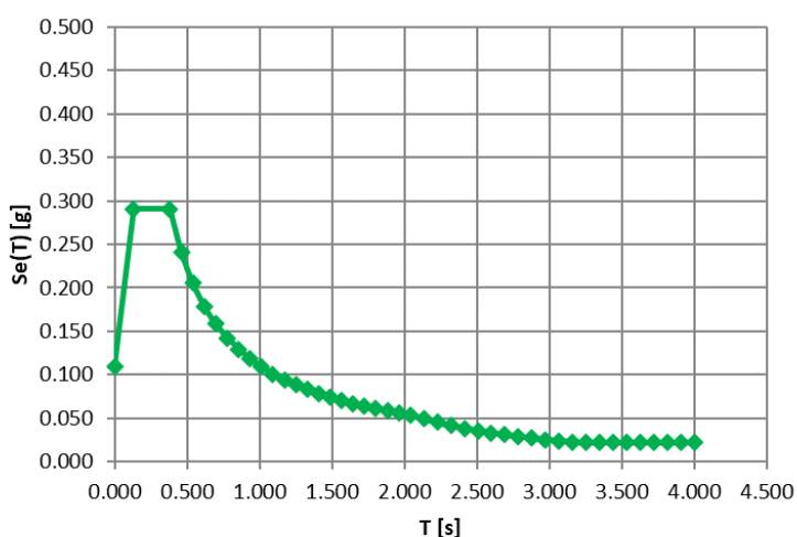
Figura 4 - IV01 (NV07) Stato Limite di Salvaguardia della Vita: Spettro di risposta elastico in accelerazione, classe di sottosuolo A, categoria topografica T_I , V_N = 75 anni e C_U di tipo III (NTC 2018)
