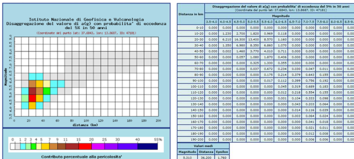
Figura 6 - IV01 (NV07): Magnitudo e distanza
