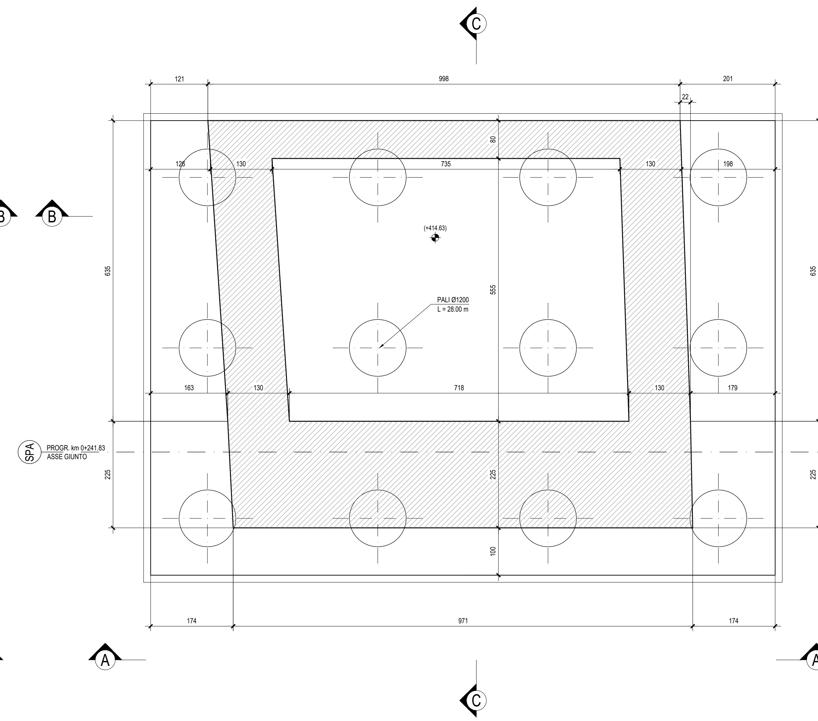
PIANTA SPICCATO - Scala 1:50
