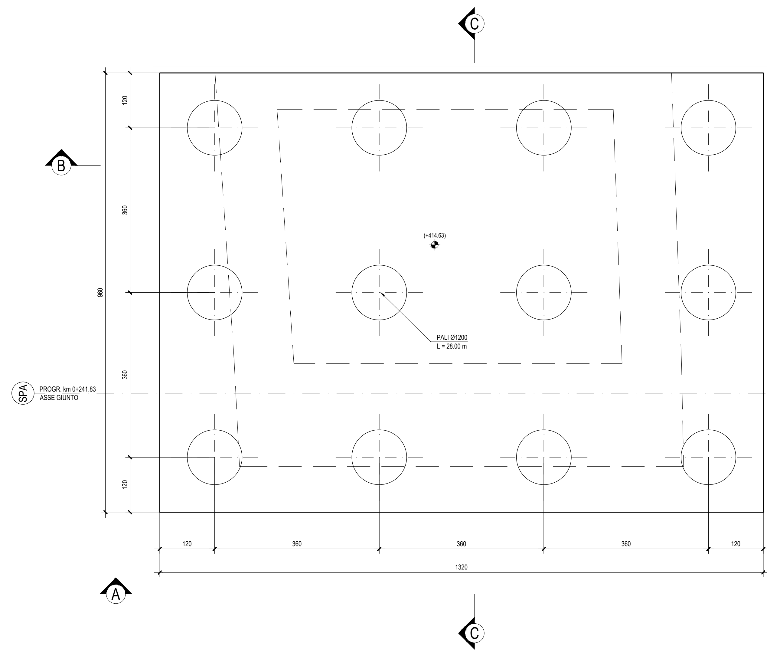
PIANTA FONDAZIONI - Scala 1:50
