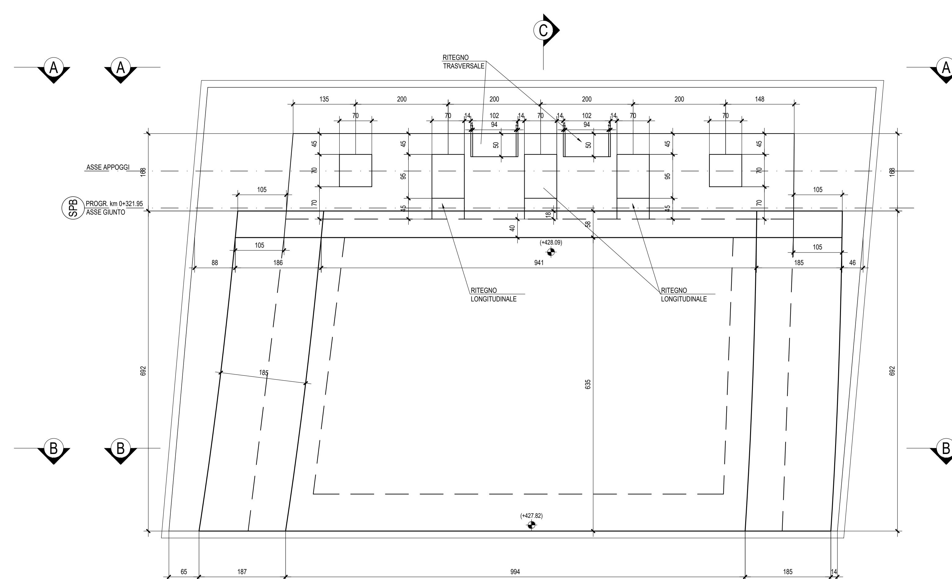
VISTA DALL'ALTO - Scala 1:50
