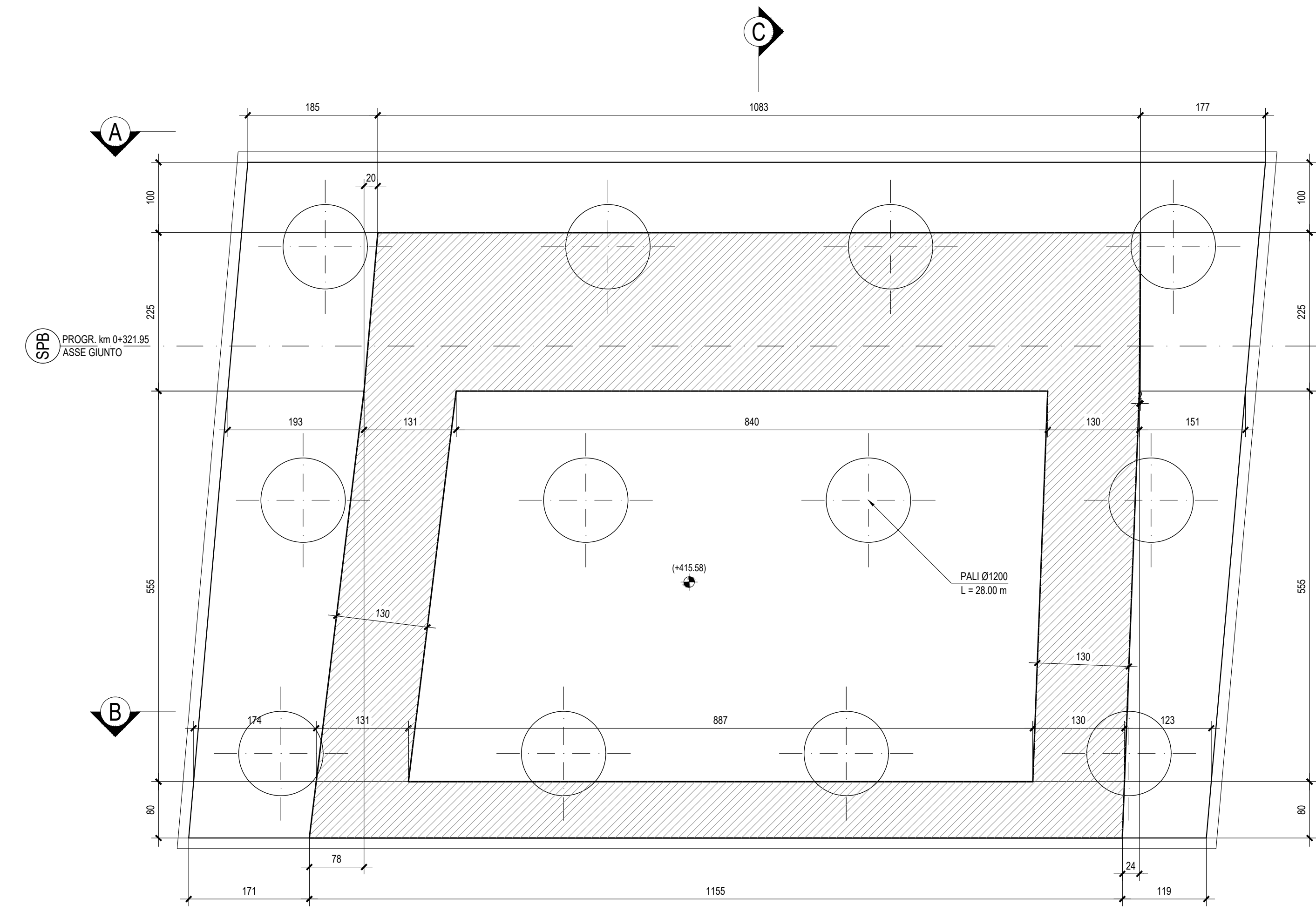
PIANTA SPICCATO - Scala 1:50
