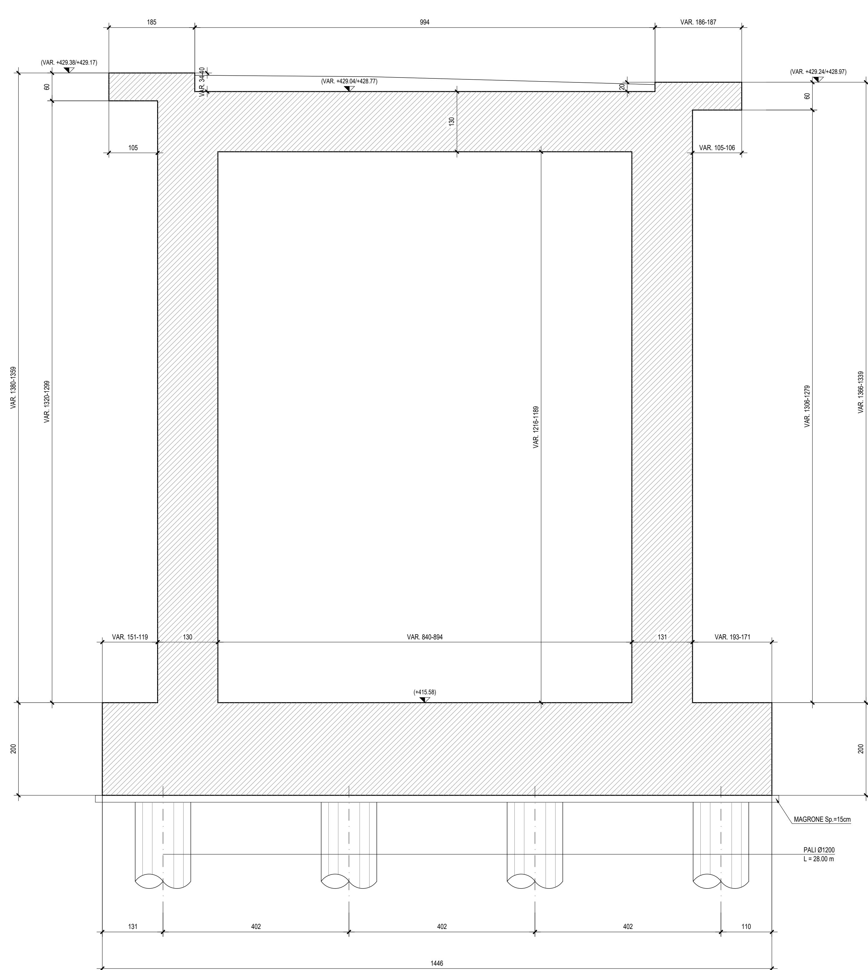
SEZIONE B-B - Scala 1:50
