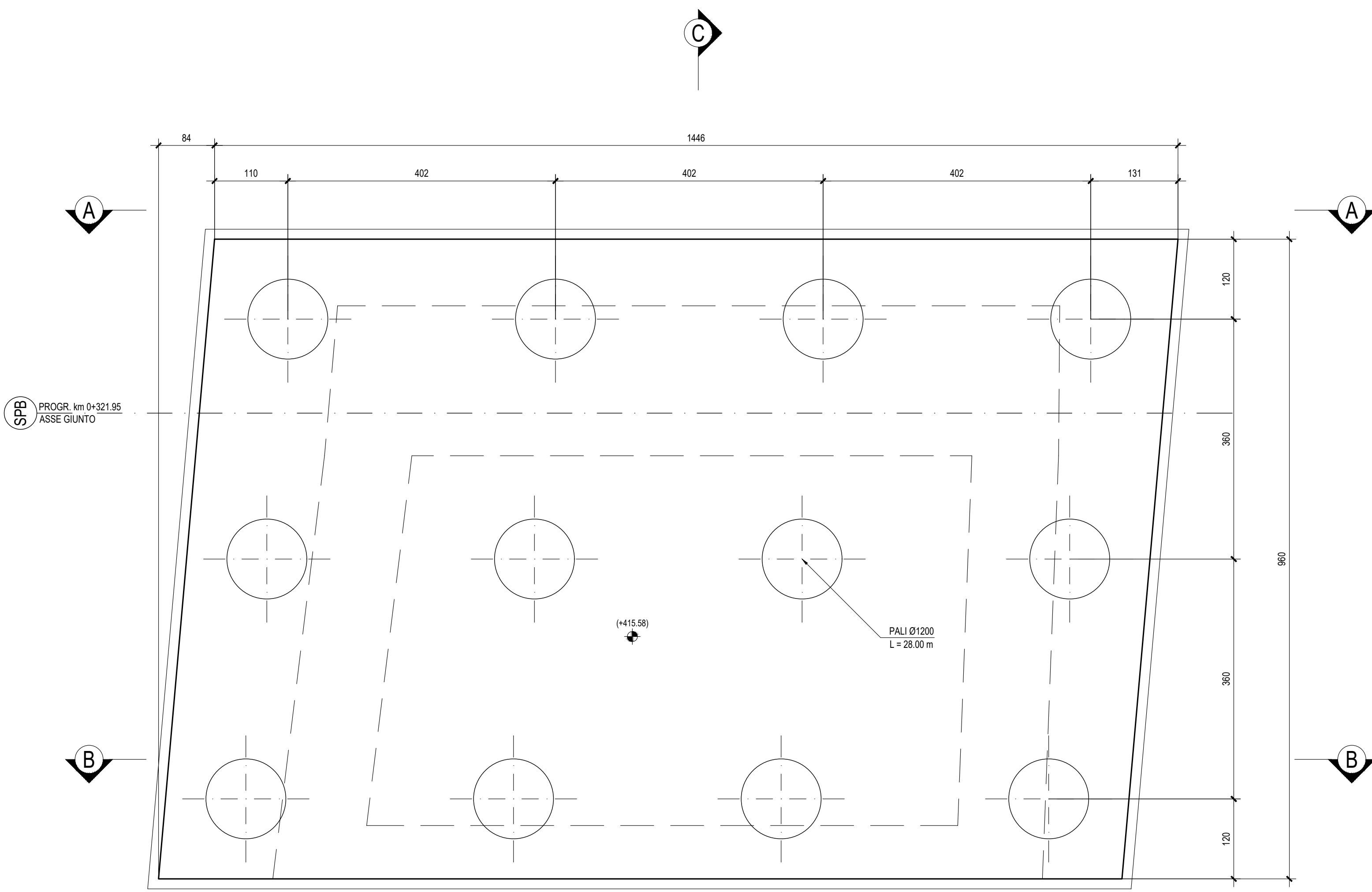
PIANTA FONDAZIONI - Scala 1:50
