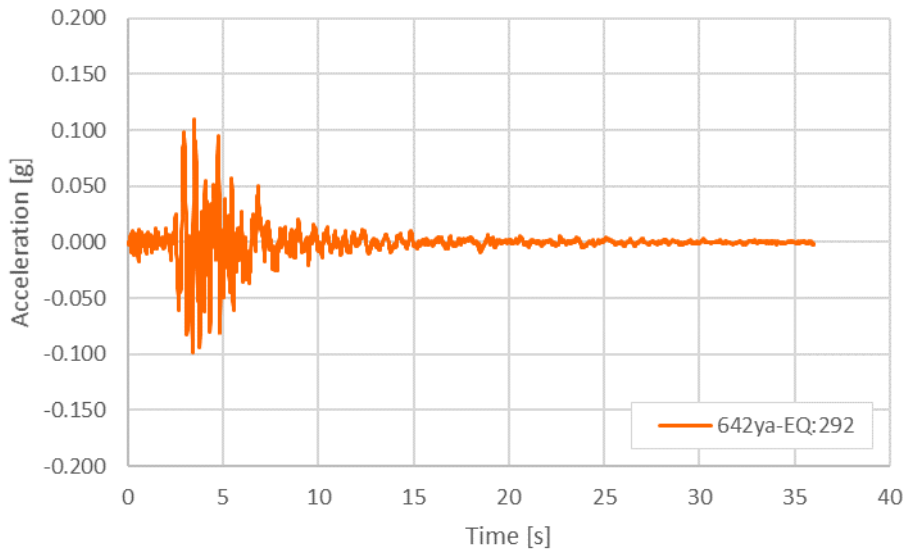
Figura 12 – Accelerogramma naturale: Waveform 642ya – Eartquake 292
