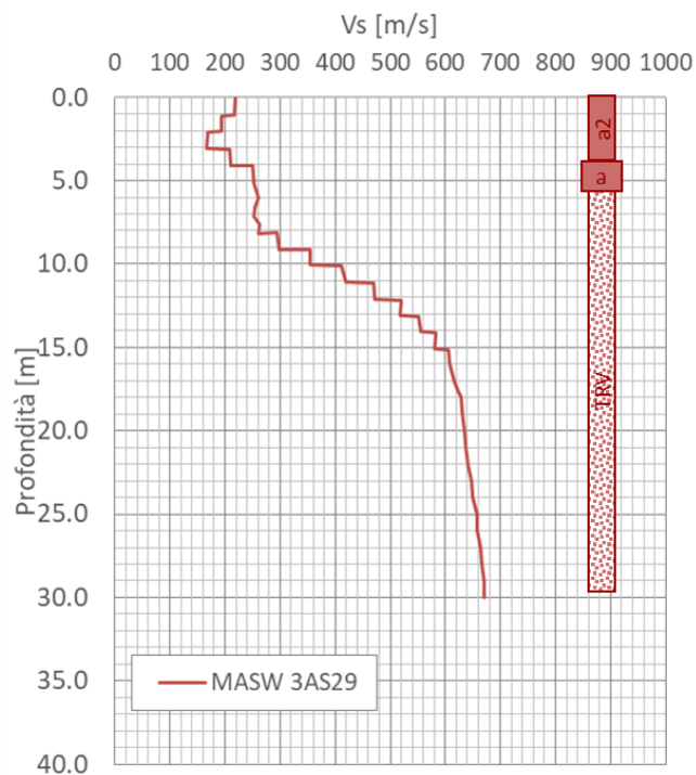
Figura 2 – Indagine sismica eseguita per il viadotto IV02 (NV51a) con relativa stratigrafia: MASW 3AS29 ( V_s, q= 393 m/s - Suolo tipo B)
