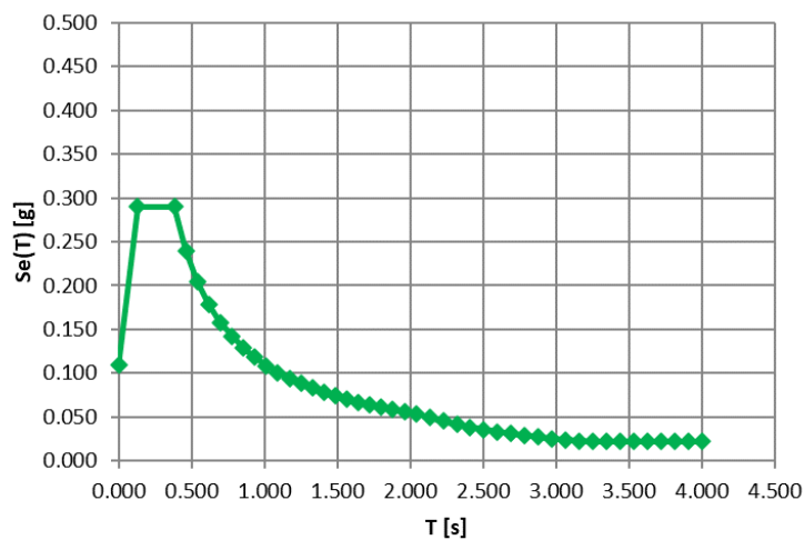
Figura 4 - IV02 (NV51a) Stato Limite di Salvaguardia della Vita: Spettro di risposta elastico in accelerazione, classe di sottosuolo A, categoria topografica T_I , V_N = 75 anni e C_U di tipo III (NTC 2018)
