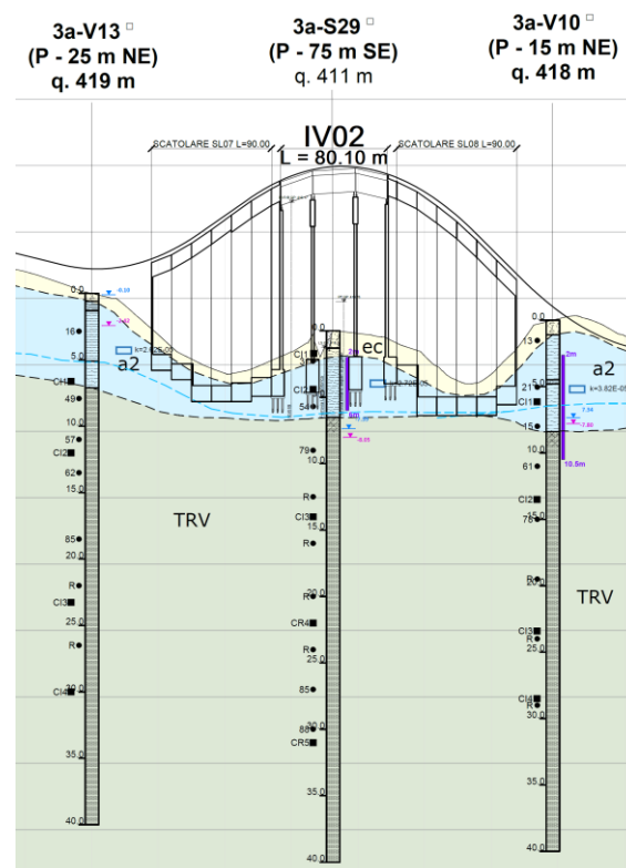
Figura 1: Profilo stratigrafico relativo al viadotto IV02 (NV51a)
