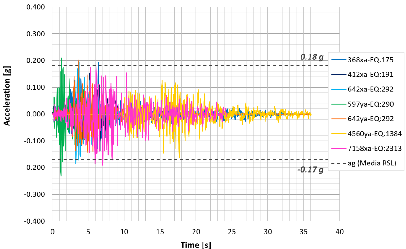
Figura 18 – Risposta Sismica Locale per SLV di L3A – IV02 (NV51a): Accelerogrammi a 4,0 m di profondità
