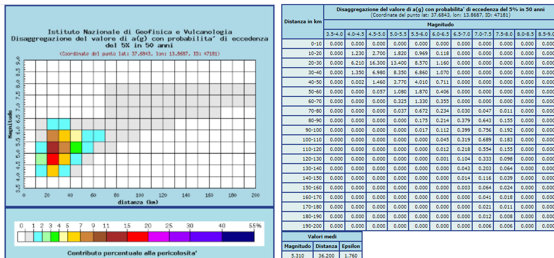
Figura 6 - IV02 (NV51a): Magnitudo e distanza
