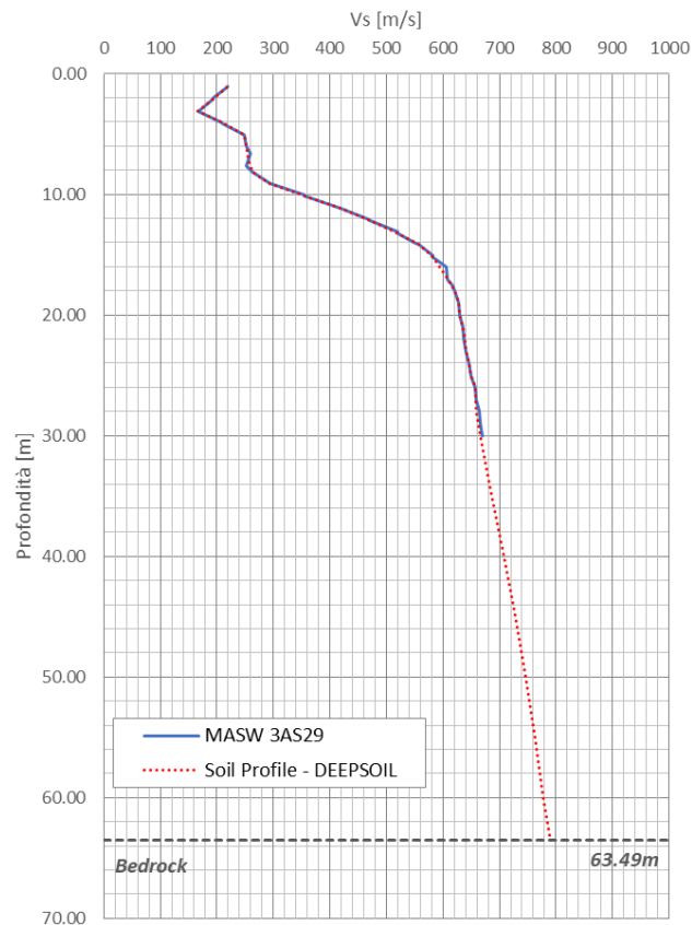
Figura 17 – Soil Profile adottato
