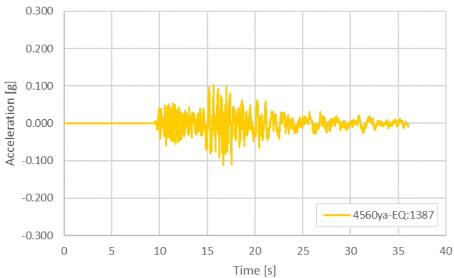
Figura 13 – Accelerogramma naturale: Waveform 4560ya – Eartquake 1387
