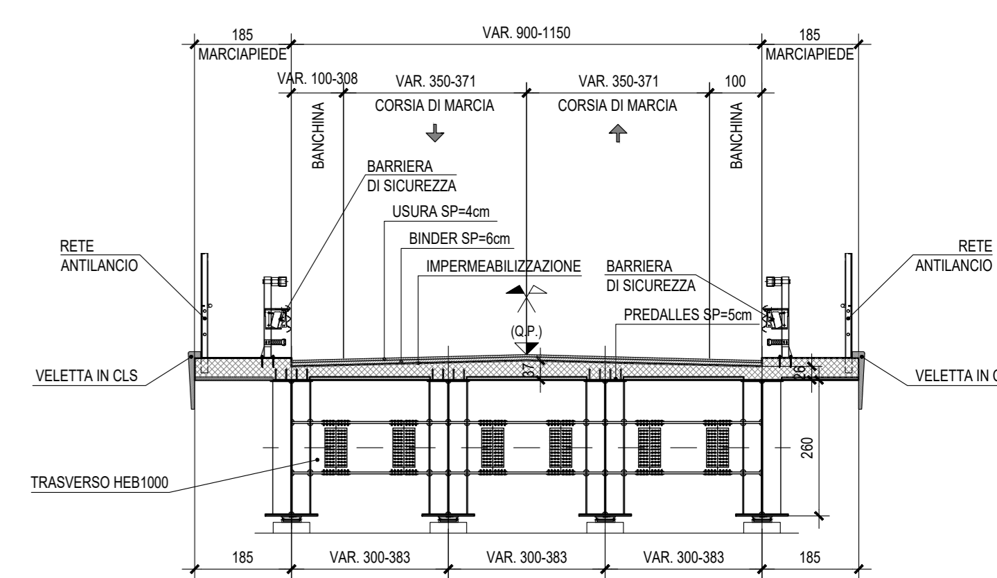
SEZIONE TRASVERSALE CAMPATA Scala 1:100
