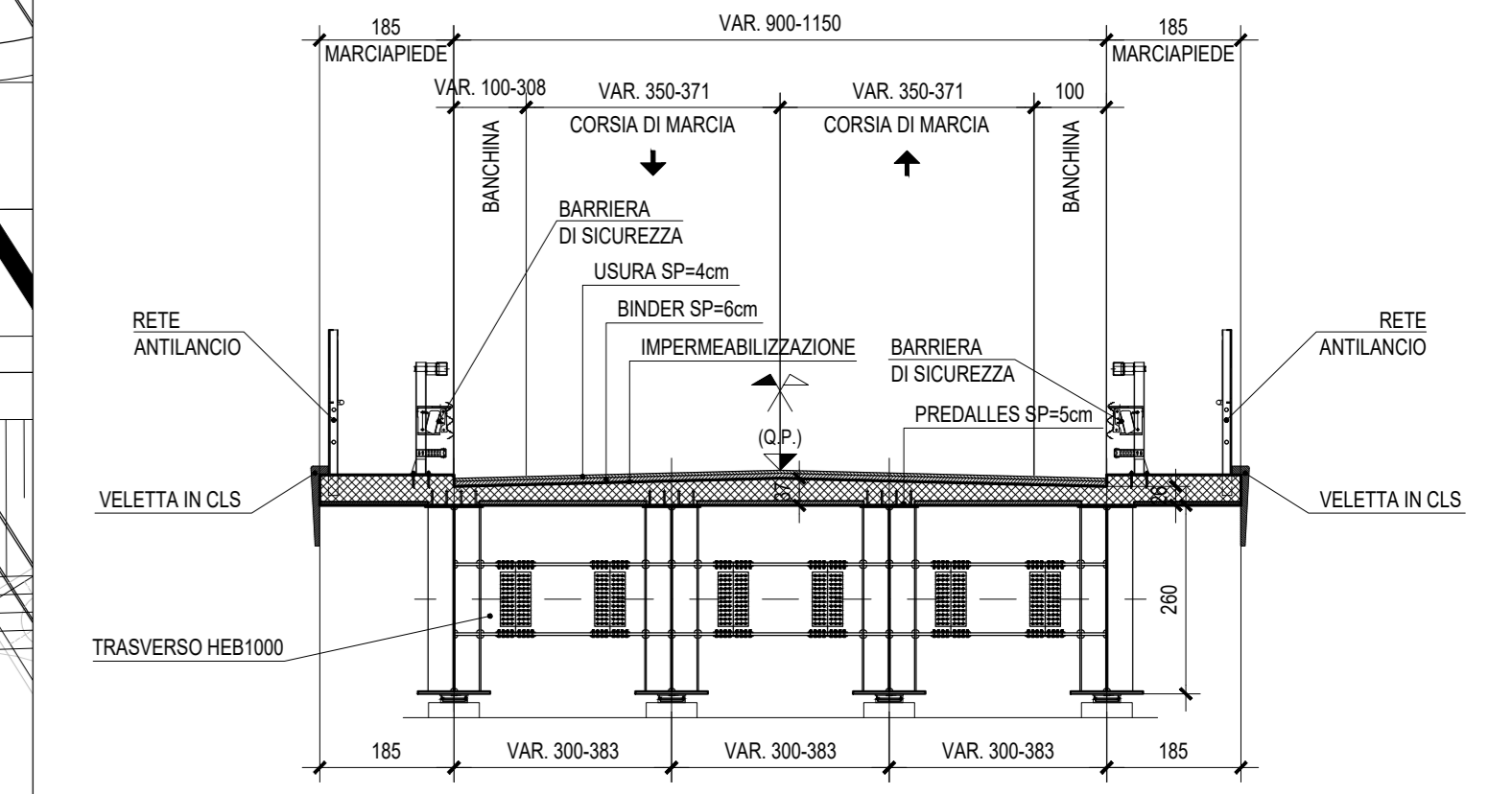
SEZIONE TRASVERSALE CAMPATA Scala 1:100
