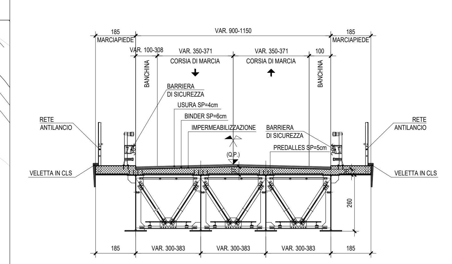
SEZIONE TRASVERSALE CAMPATA Scala 1:100
