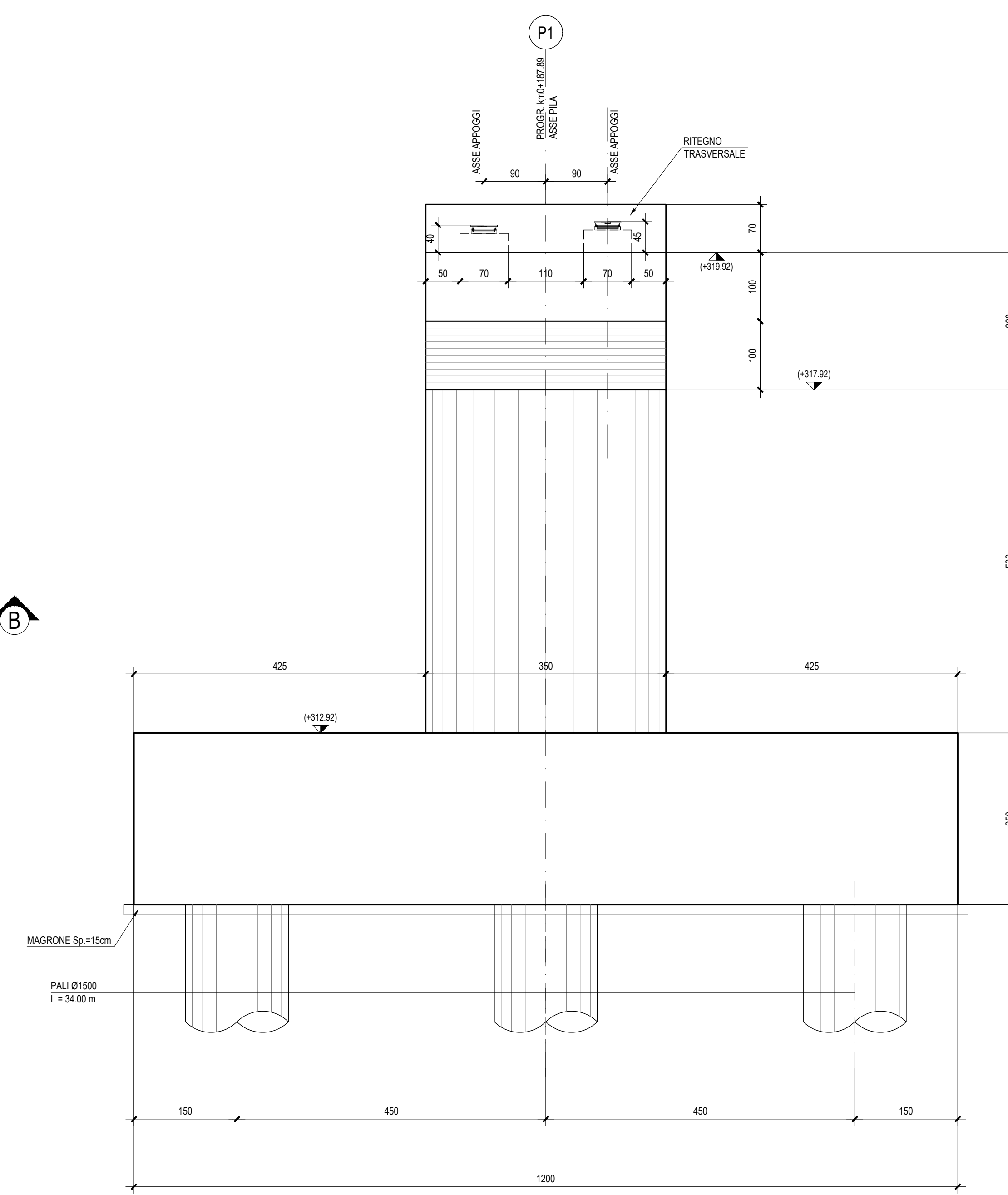
VISTA LATERALE - Scala 1:50
