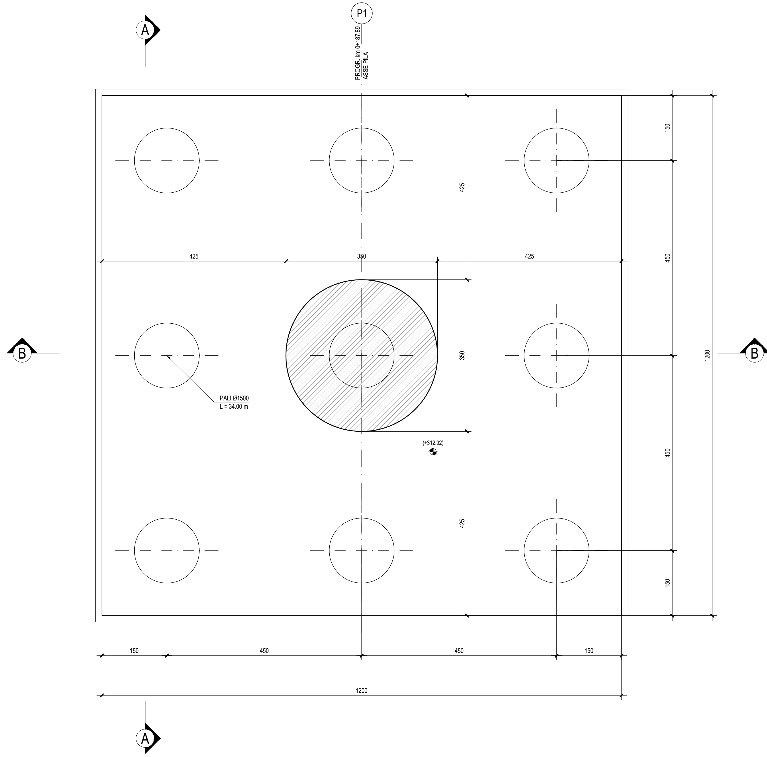
PIANTA SPICCATO - Scala 1:50
