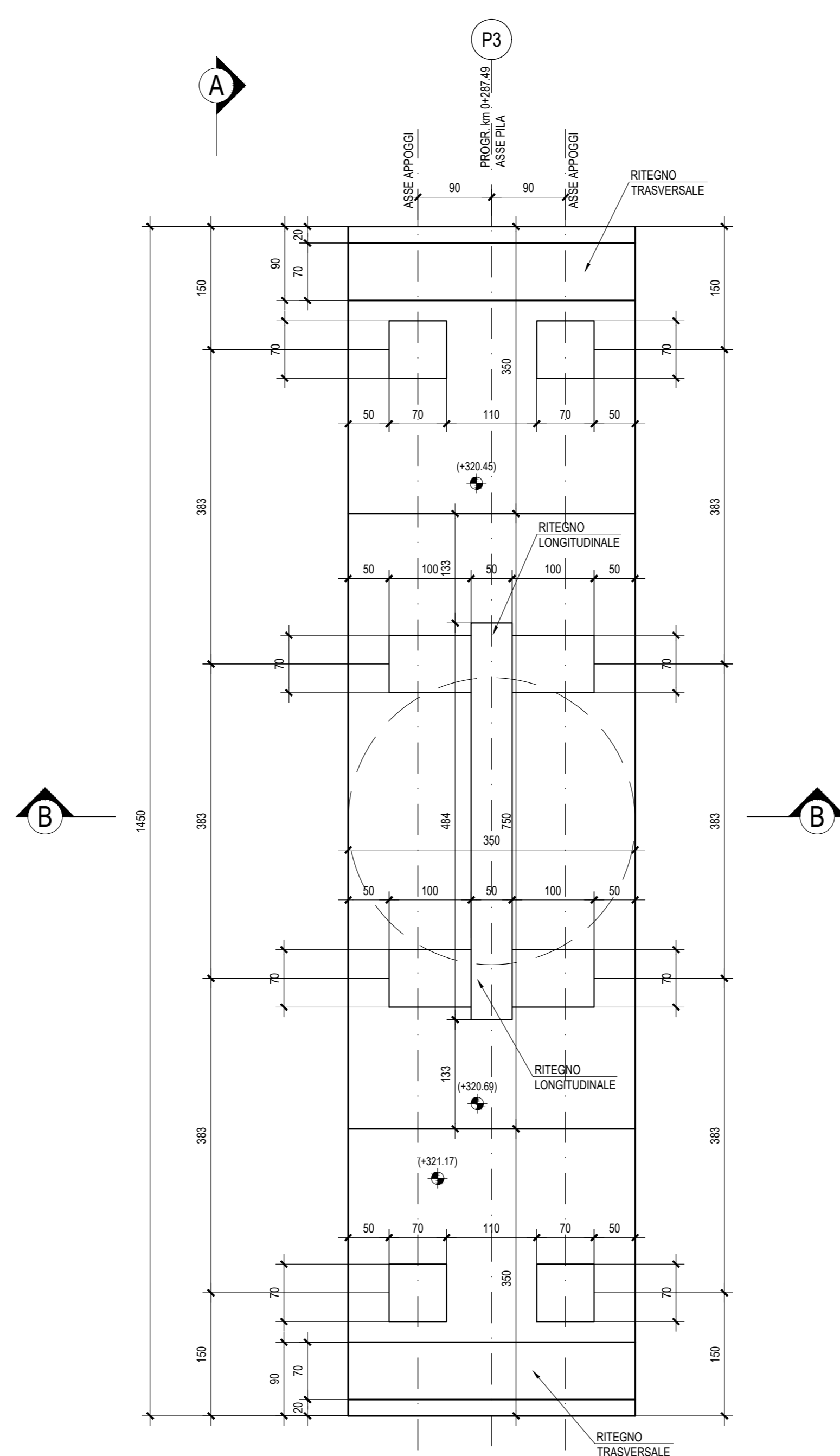
PIANTA PULVINO - Scala 1:50
