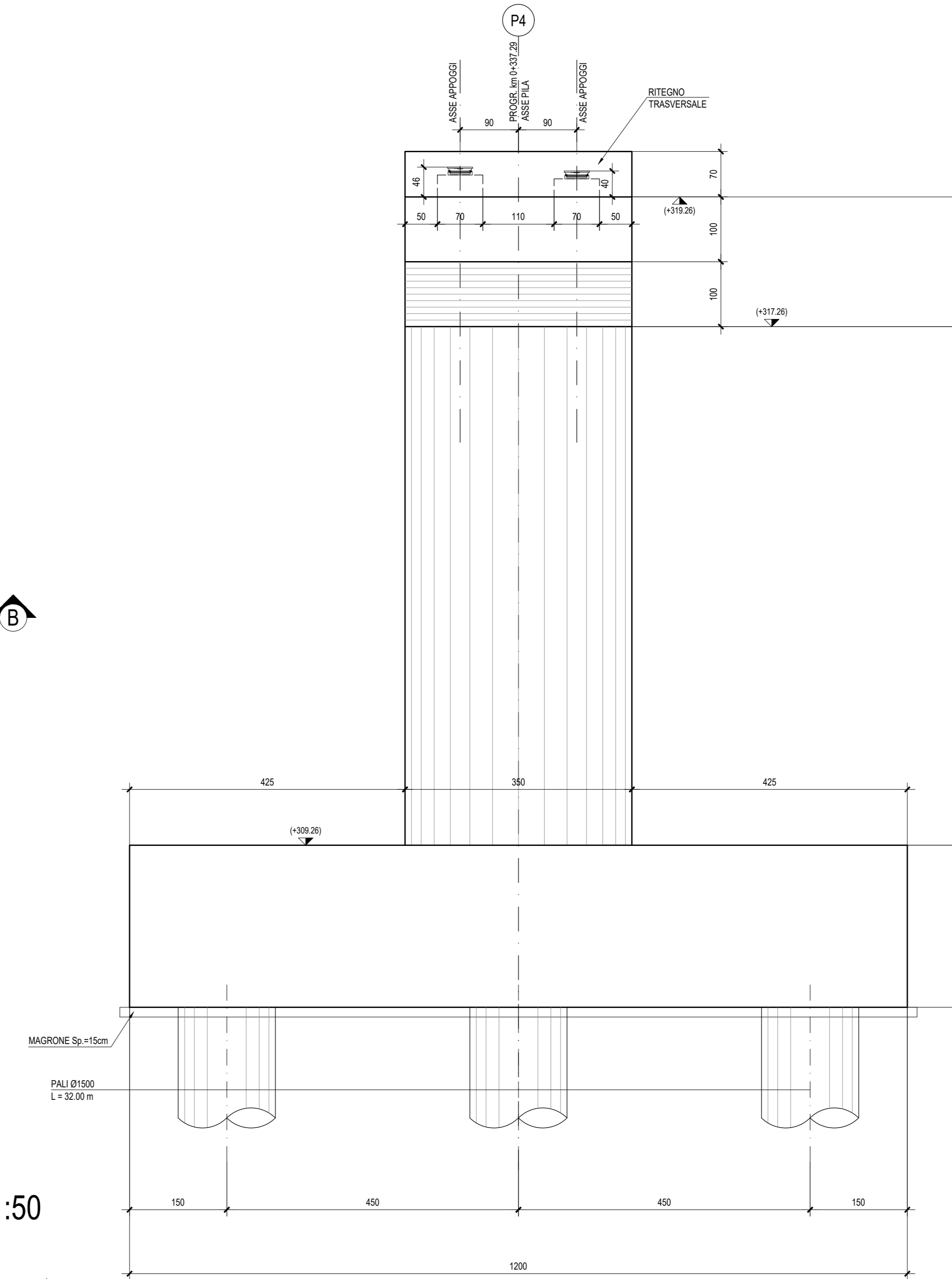
VISTA LATERALE - Scala 1:50
