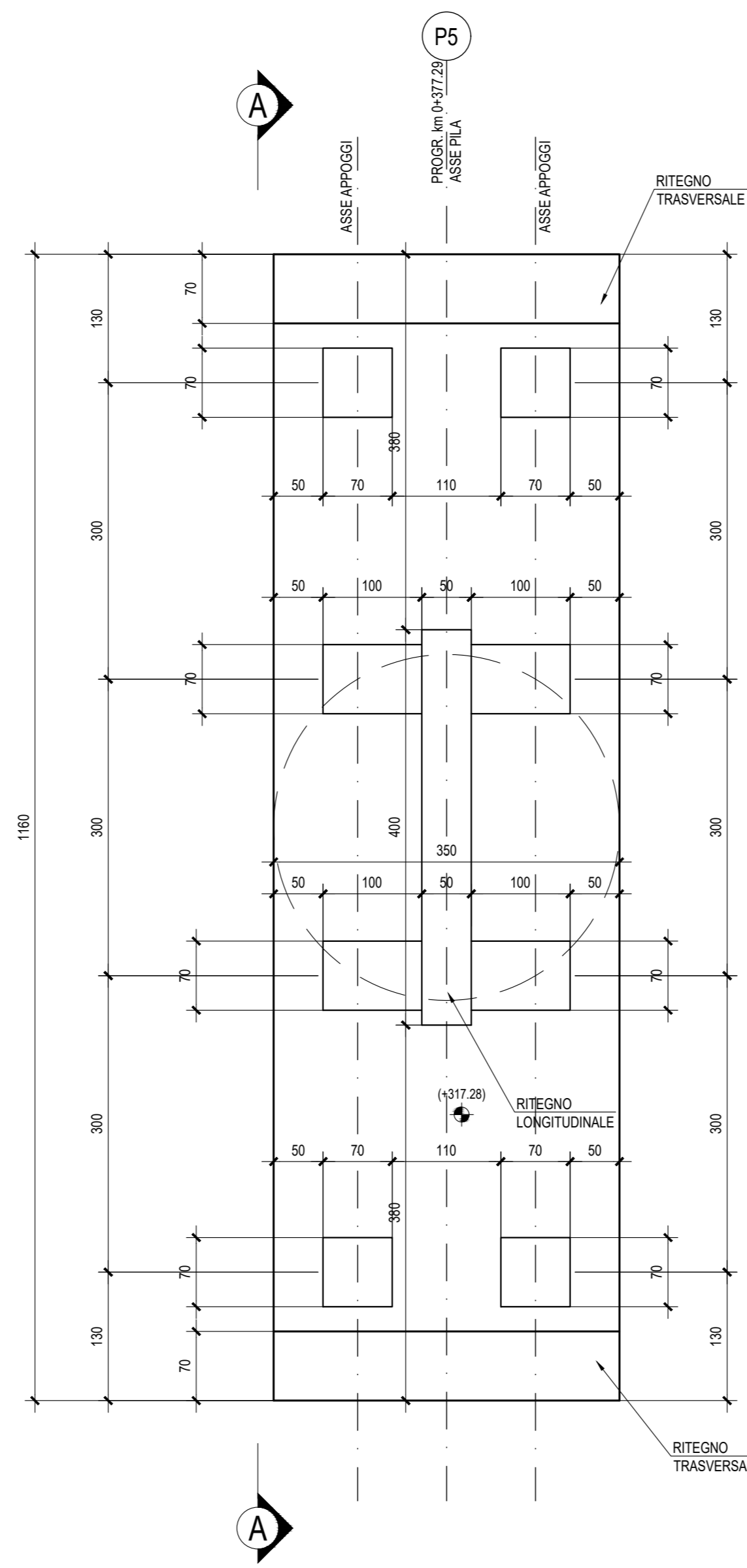
PIANTA PULVINO - Scala 1:50
