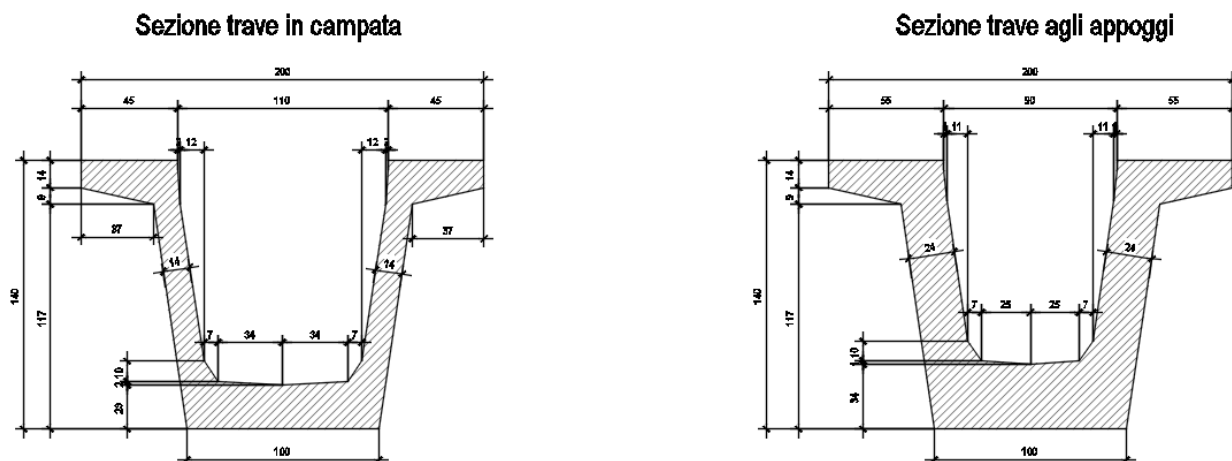
Figura 2 – Sezione della trave in c.a.p.
