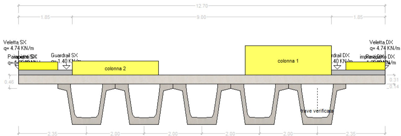
Figura 14 - Disposizione per calcolo M min su trasverso
