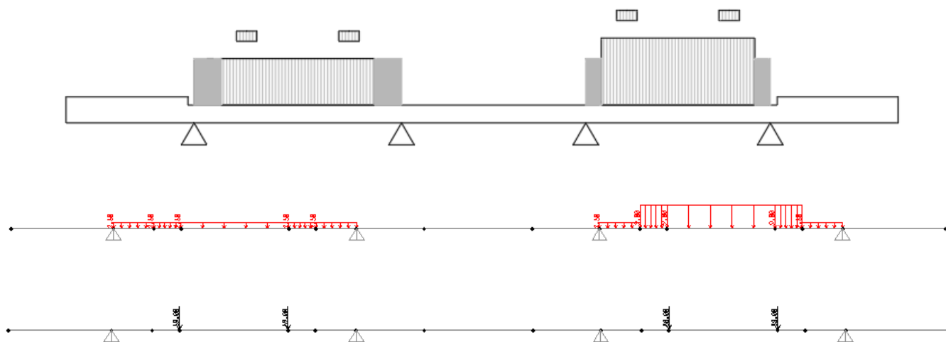
Figura 15: condizione di carico 2
