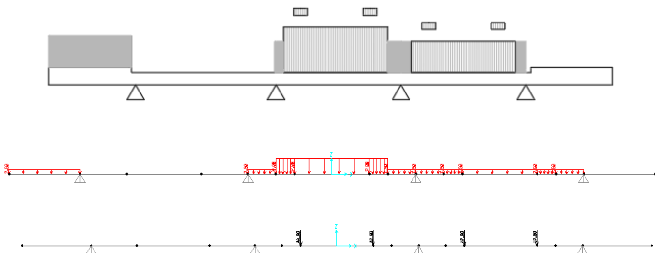
Figura 16: condizione di carico 2
