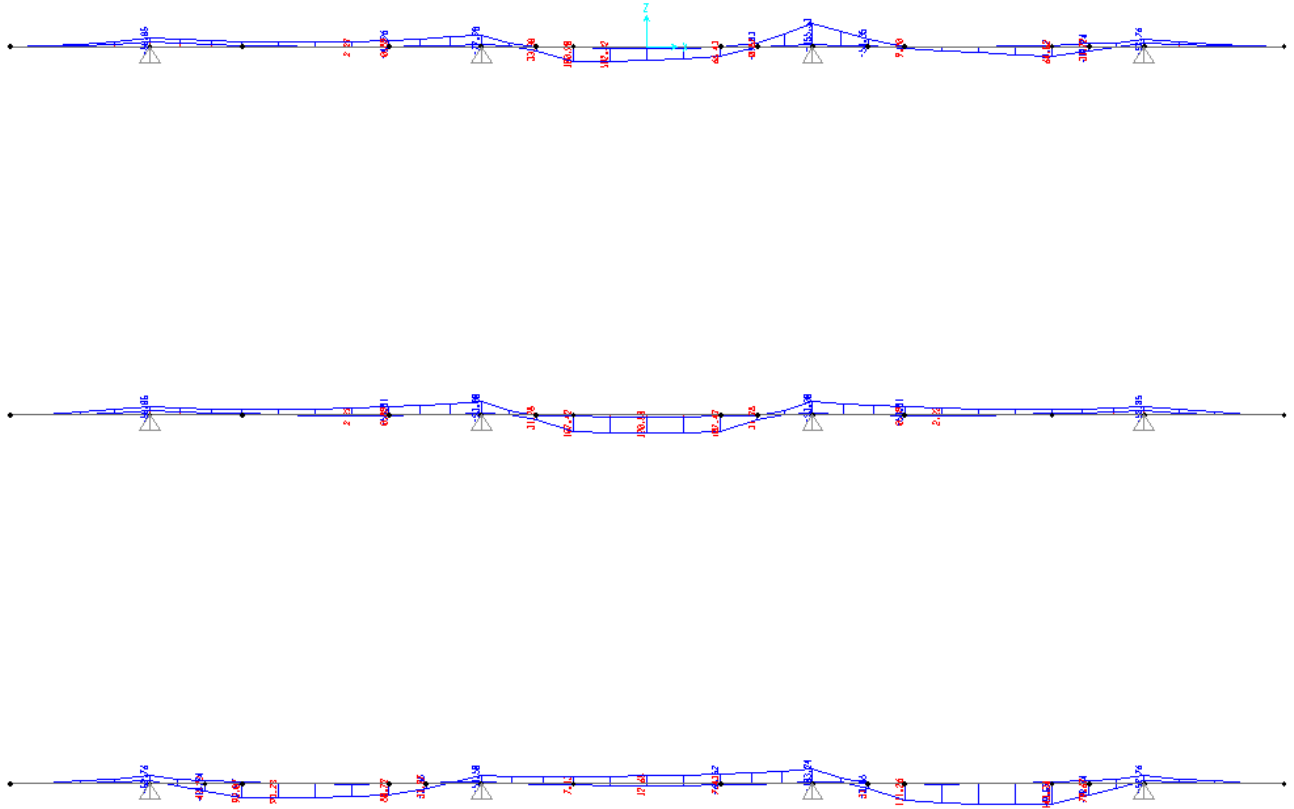
Figura 17: involuppo momento flettente SLU
