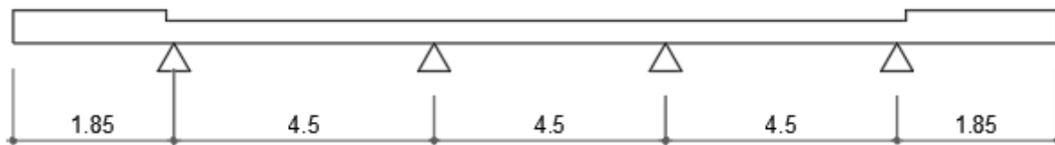
Figura 7. Schema statico
