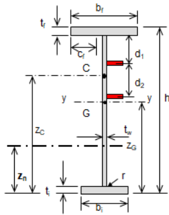
SEZIONE MONO-SIMMETRICA
