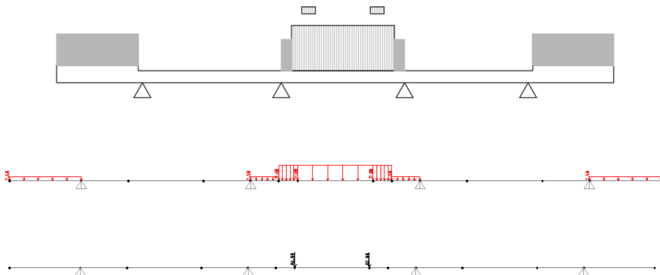
Figura 14: condizione di carico 1
