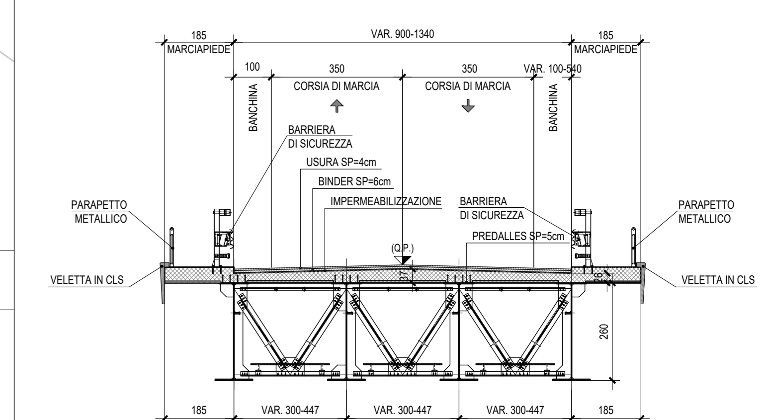
SEZIONE TRASVERSALE CAMPATA Scala 1:100
