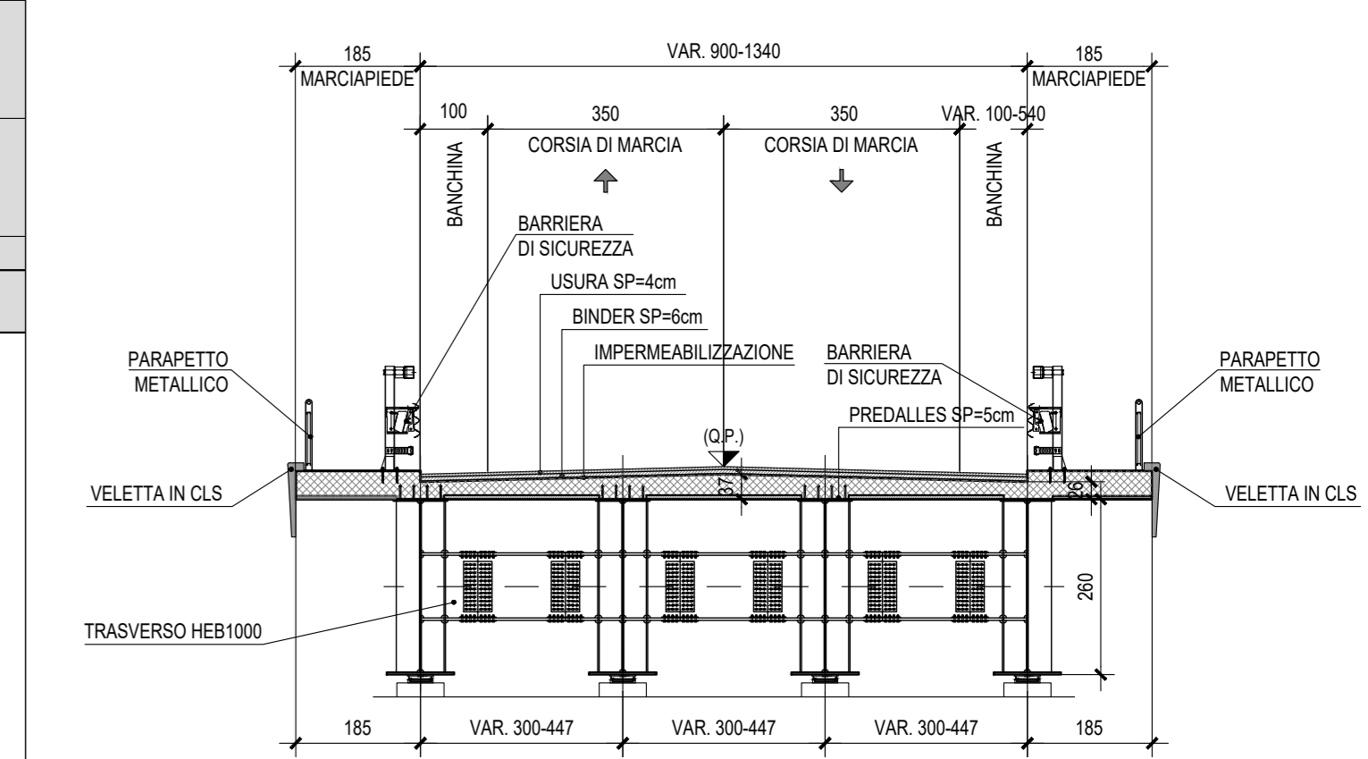
SEZIONE TRASVERSALE APPOGGI Scala 1:100
