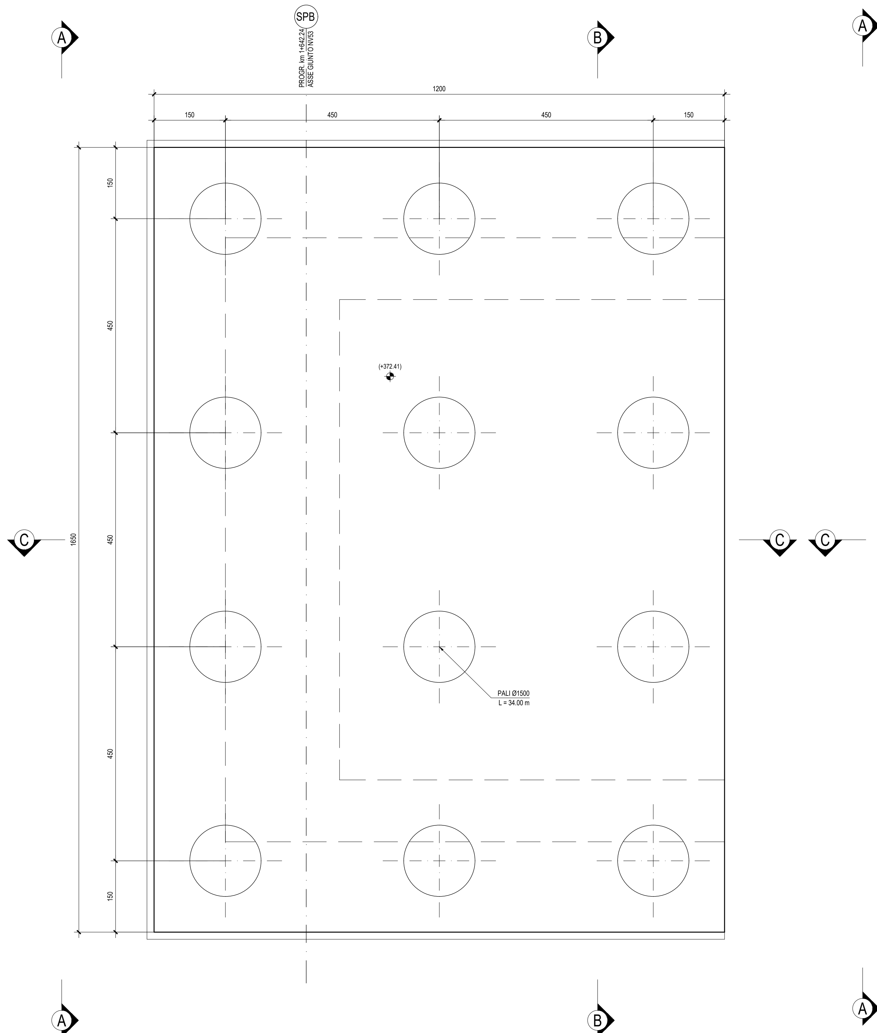
PIANTA FONDAZIONI - Scala 1:50
