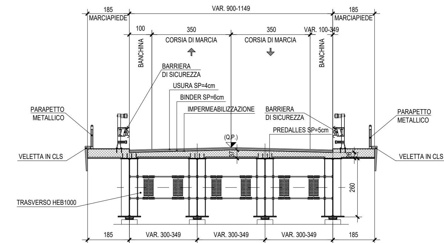
SEZIONE TRASVERSALE CAMPATA SCALA 1:100
