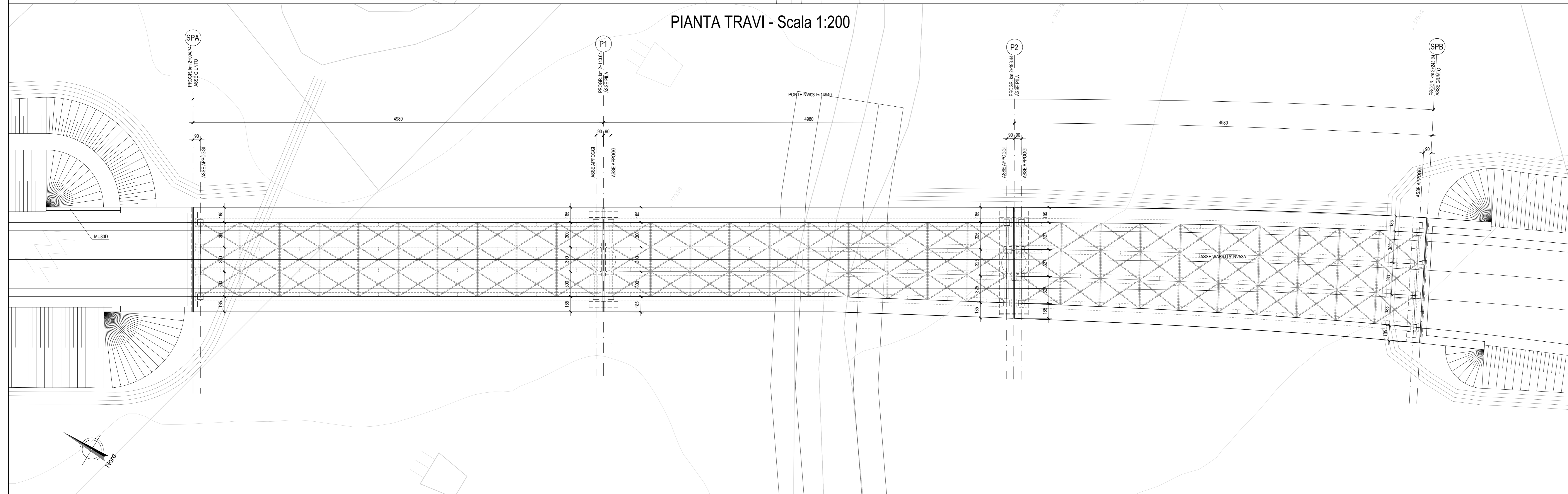
PROSPETTO - Scala 1:200
