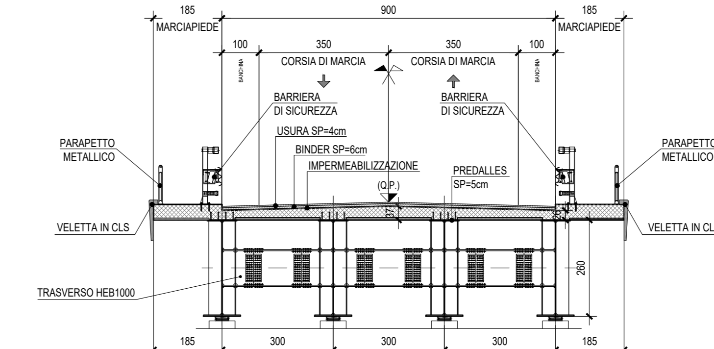
SEZIONE TRASVERSALE IMPALCATO METALLICO CAMPATA - SCALA 1:100
