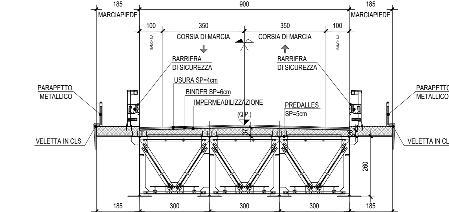
SEZIONE TRASVERSALE IMPALCATO METALLICO CAMPATA - SCALA 1:100
