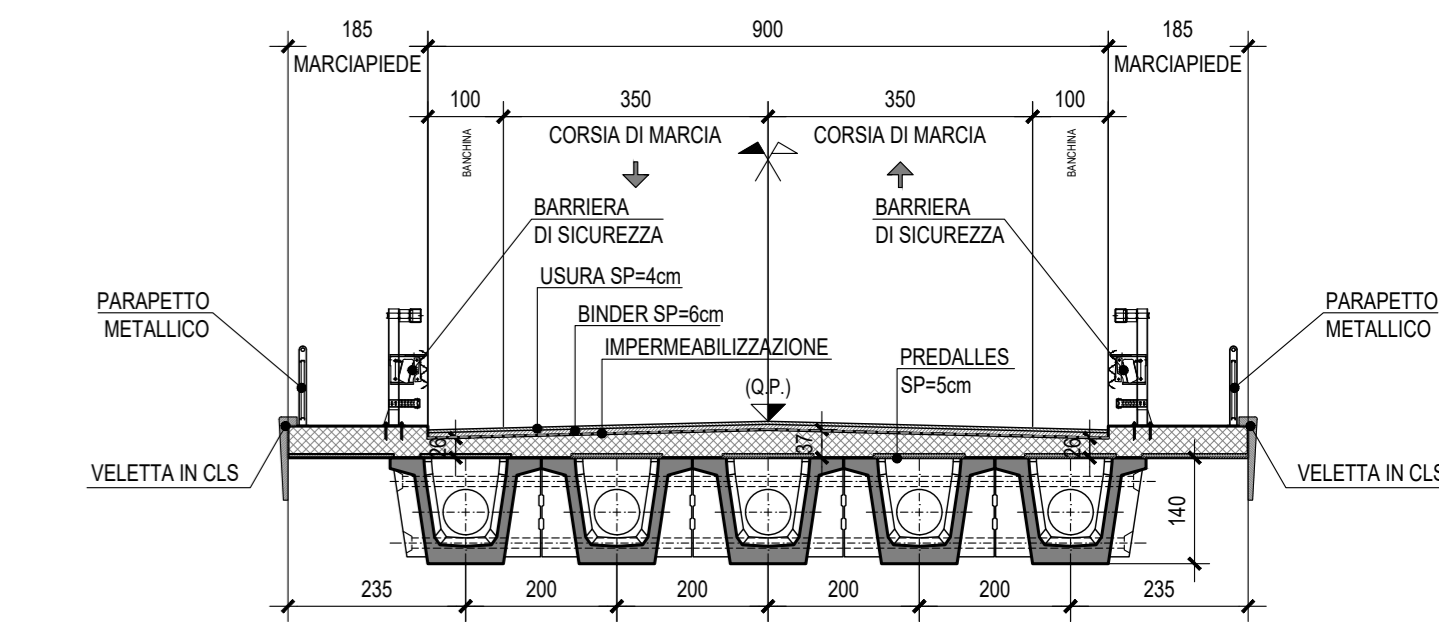
SEZIONE TRASVERSALE IMPALCATO IN CAP SCALA 1:100
