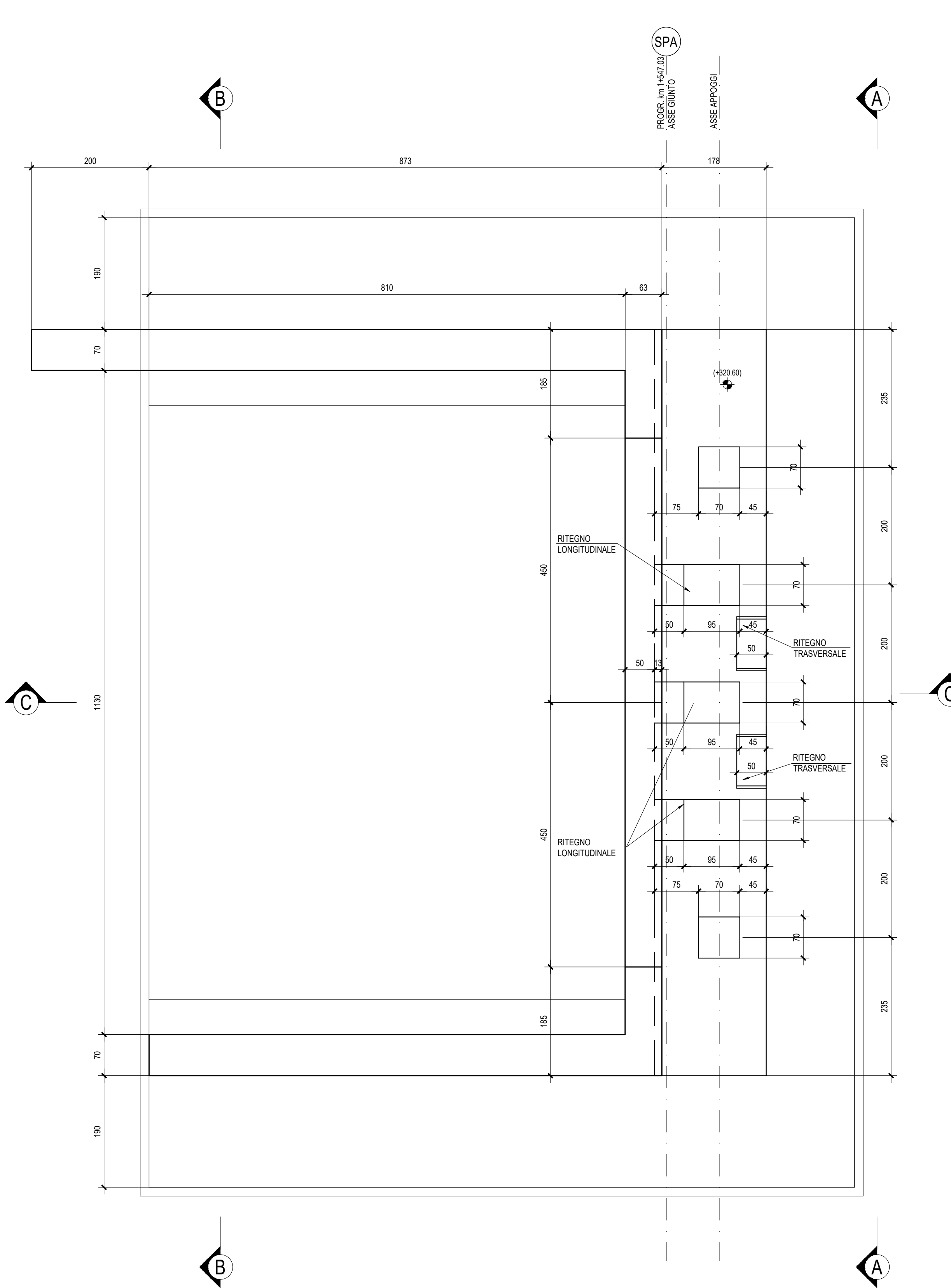
VISTA DALL'ALTO - Scala 1:50
