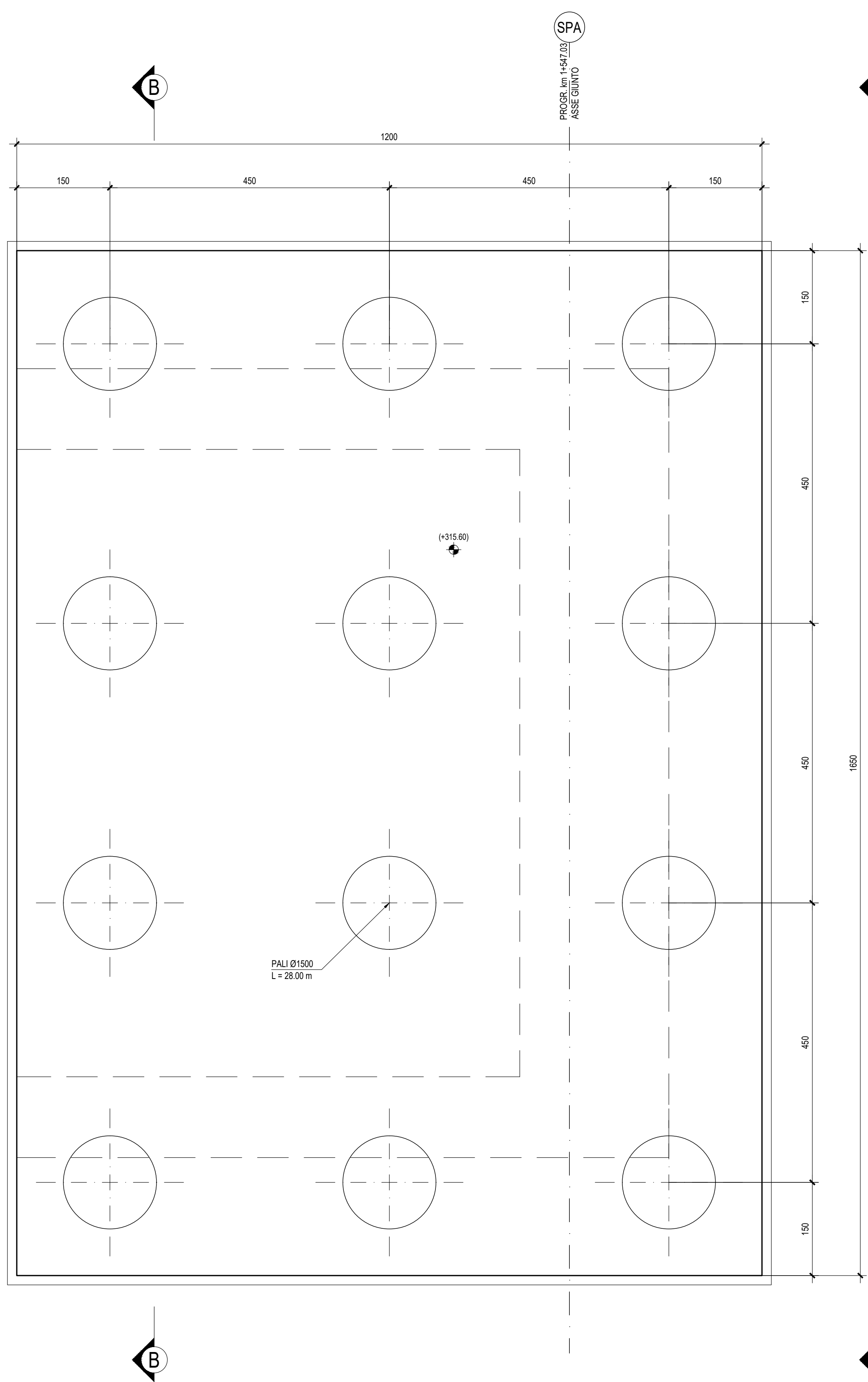
PIANTA FONDAZIONI - Scala 1:50
