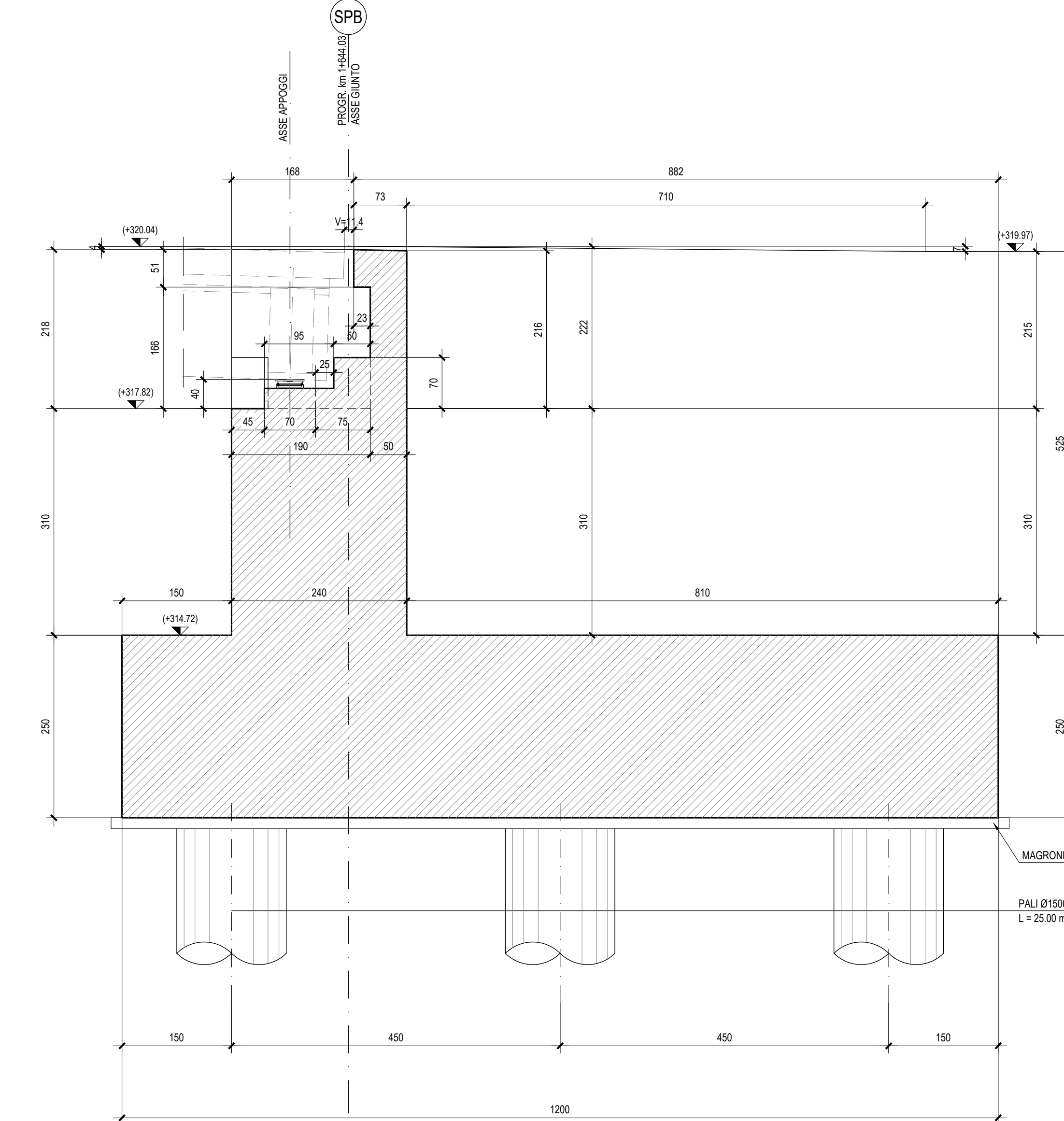
SEZIONE C-C - Scala 1:50
