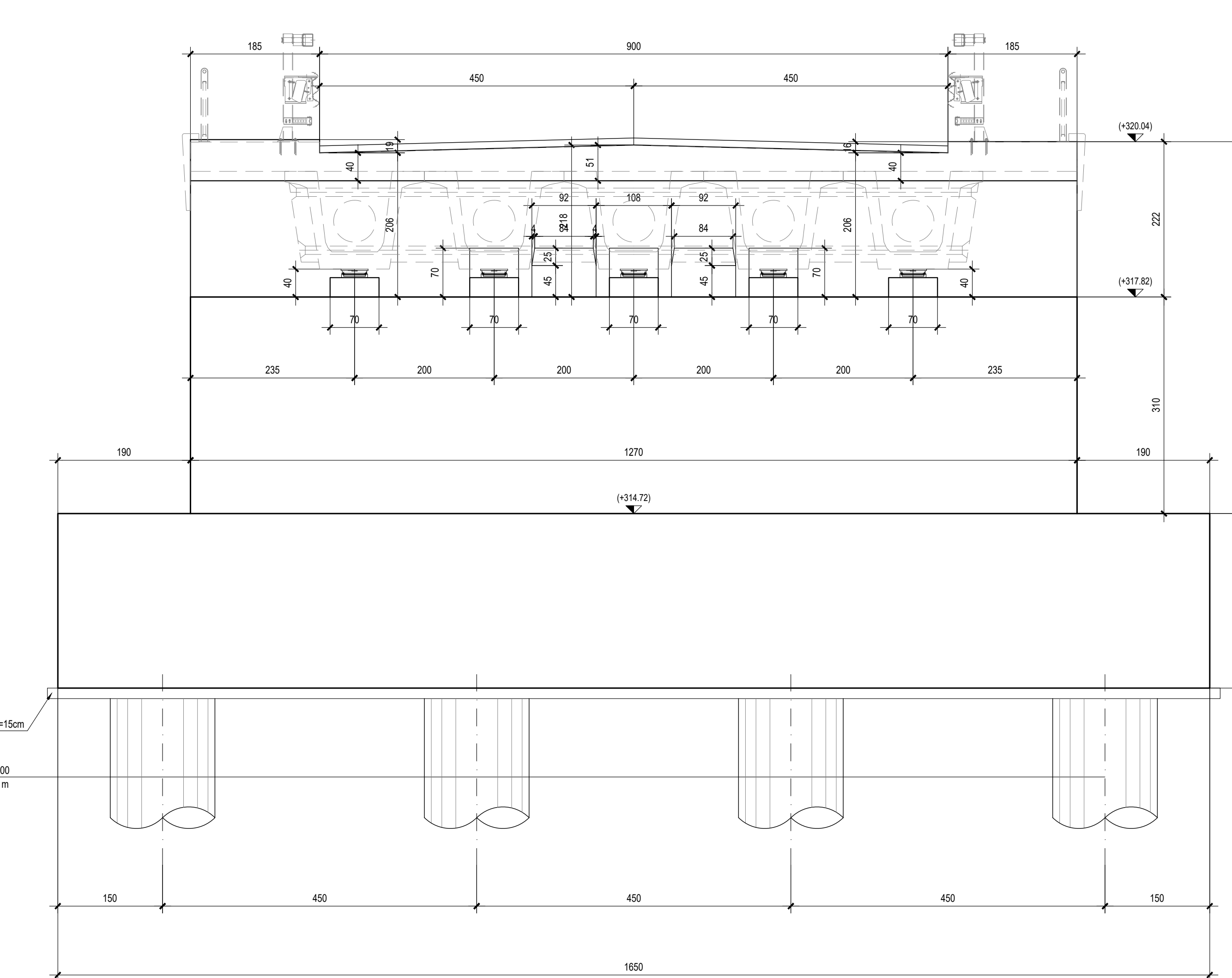
VISTA A-A - Scala 1:50
