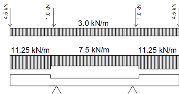
Figura 8: carichi permanenti sulla soletta
