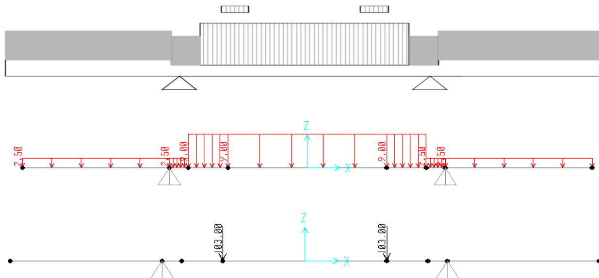
Figura 14: condizione di carico 1
