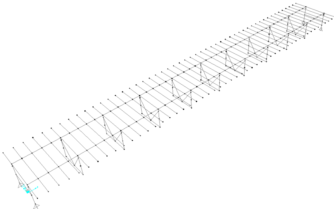
Figura 1. Modello di calcolo impalcato-Sap2000
