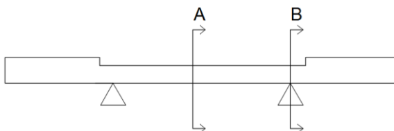
Figura 13: sezioni di interesse per la massimizzazione delle sollecitazioni
