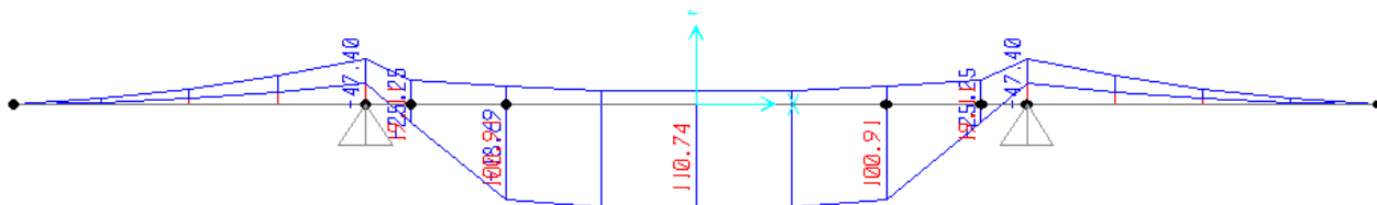
Figura 15: involuppo momento flettente SLU
