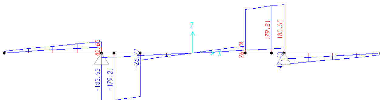
Figura 16: involuppo del taglio SLU
