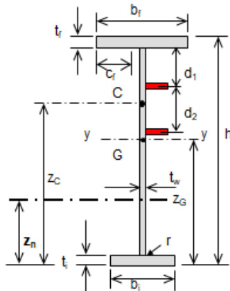
SEZIONE MONO-SIMMETRICA
