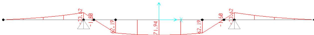
Figura 16: involuppo del taglio SLU
