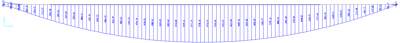
Figura 9.5 - Momento flettente (kN*m)
