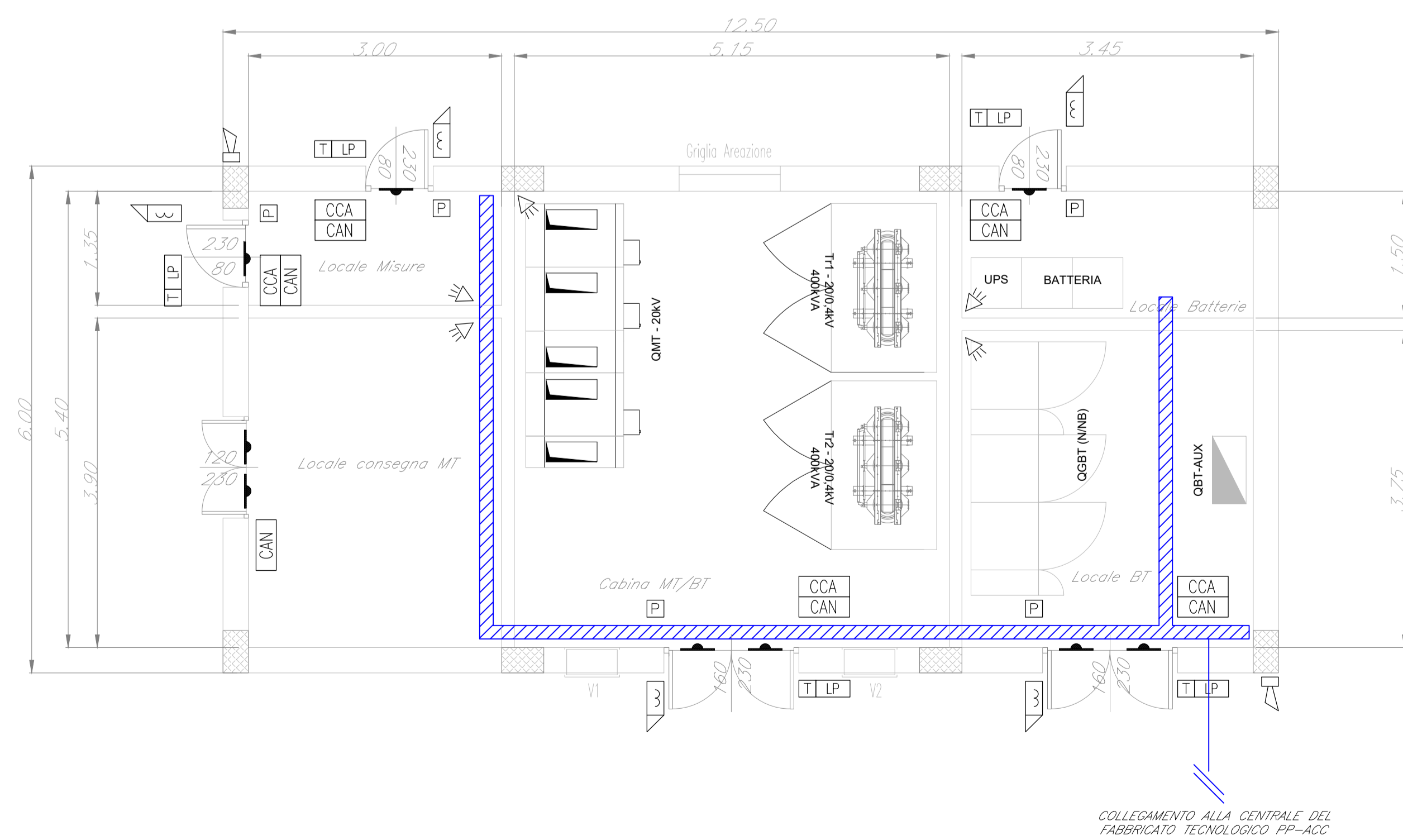
LAYOUT IMPIANTI ANTINTRUSIONE / CONTROLLO ACCESSI
