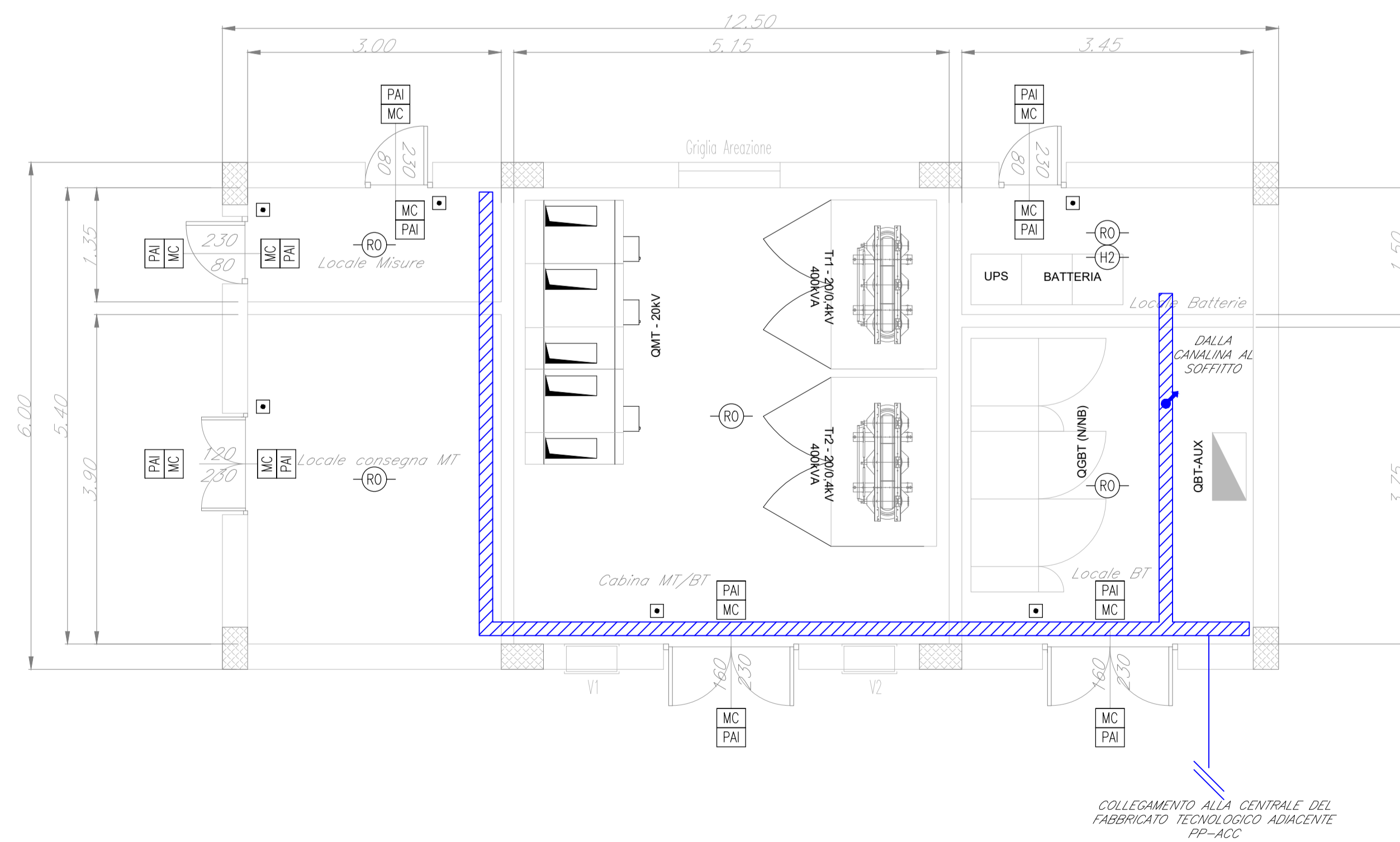
LAYOUT IMPIANTO RIVELAZIONE INCENDI - PIANO TERRA
