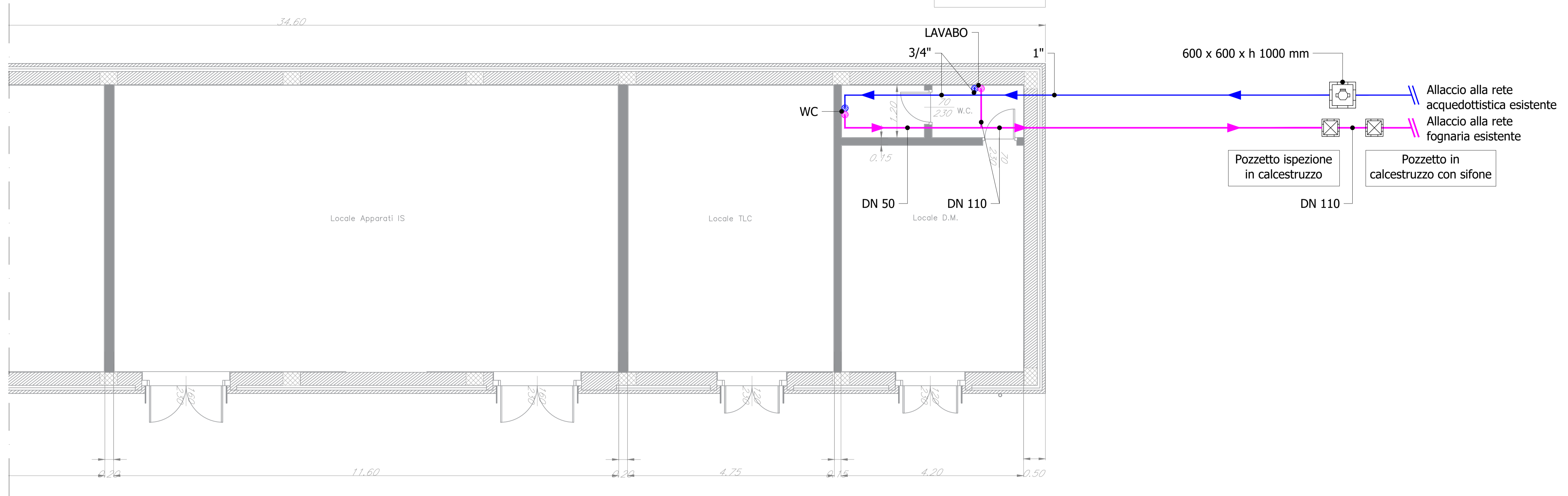
LAYOUT IMPIANTO IDRICO SANITARIO
