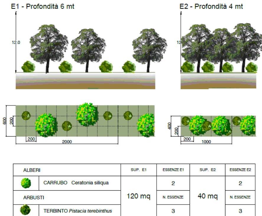
Figura 3-5: Modulo E
