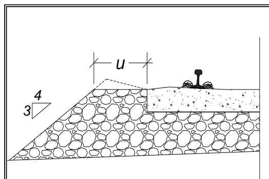
Figura 5 - Distanza minima tra testa traversa e ciglio massicciata
