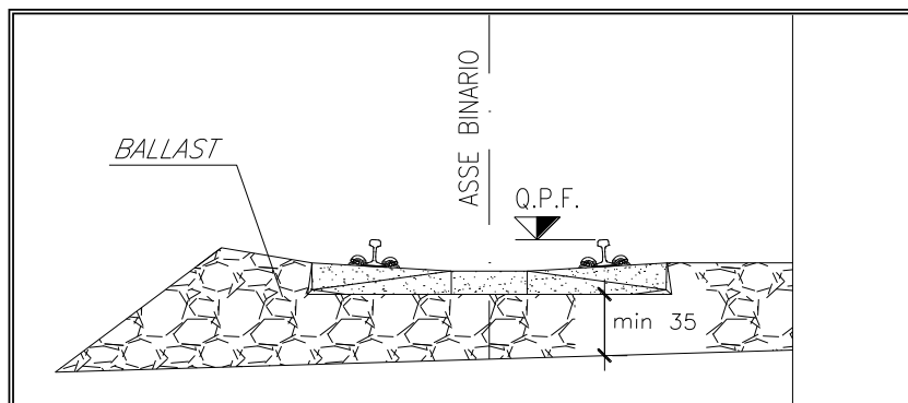
Figura 4 - Distanza minima sotto traversa per binari di corsa
