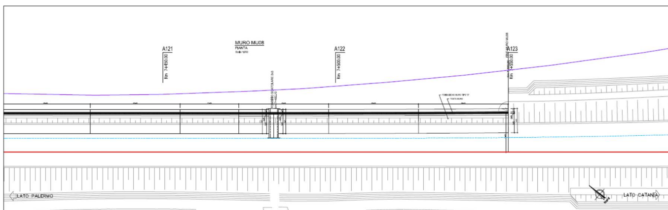
Figura 1-2 – RI05: Muro di sostegno in sx MU08 - Pianta.
