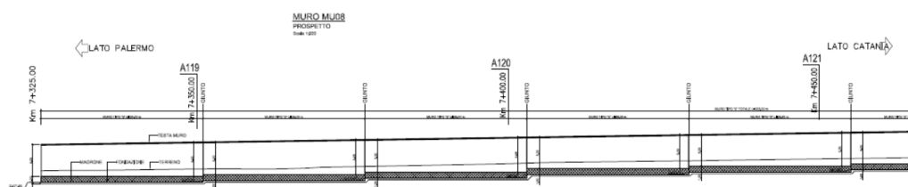
Figura 1-3 – RI05: Muro di sostegno in sx MU08 - Prospetto.
