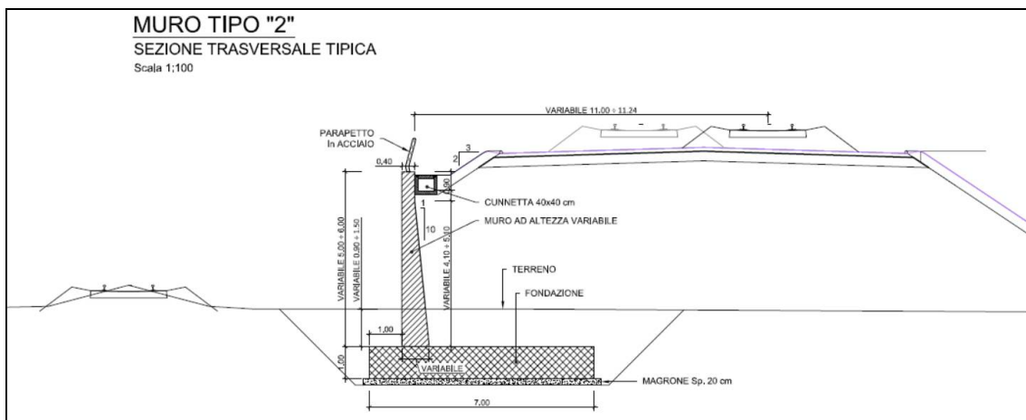
Figura 1-5 – RI05: Muro di sostegno in sx MU08 – Sezione trasversale muro tipo 2.
