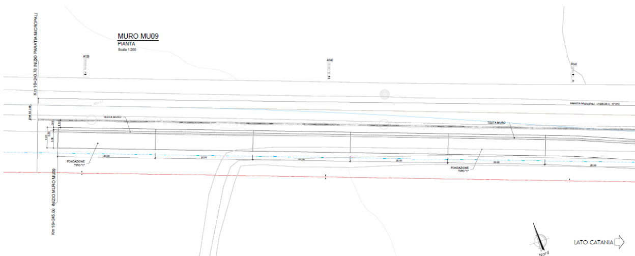
Figura 1-1 – TR04: Muro di sostegno in sx MU09 - Pianta.
