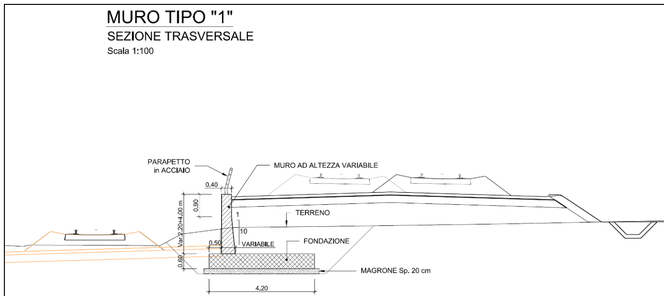
Figura 1-5 – TR04: Muro di sostegno in sx MU09 – Sezione trasversale muro tipo 1.
