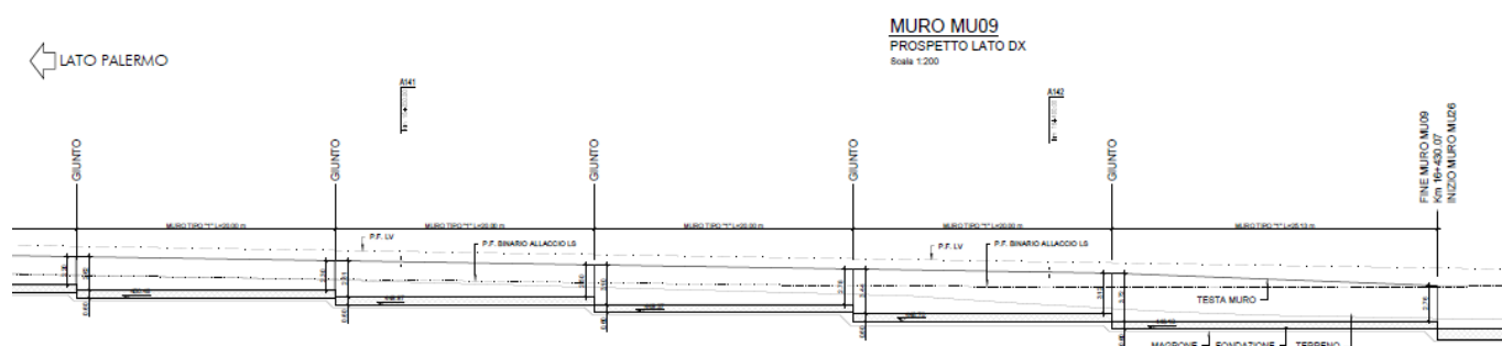
Figura 1-4 – TR04: Muro di sostegno in sx MU09 - Prospetto.
