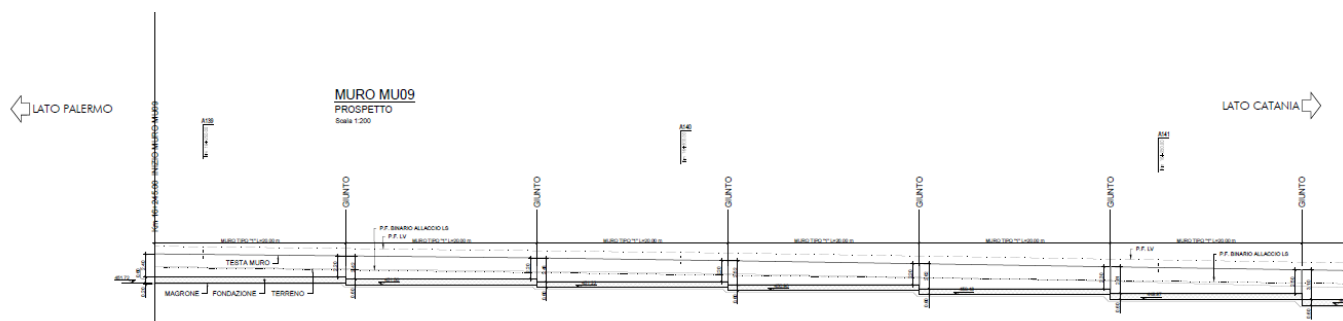
Figura 1-3 – TR04: Muro di sostegno in sx MU09 - Prospetto.
