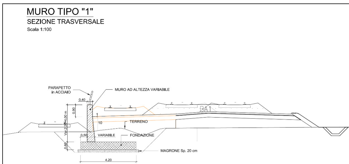
Figura 1-9 – TR04: Muro di sostegno in sx MU10 – Sezione trasversale muro tipo 1.
