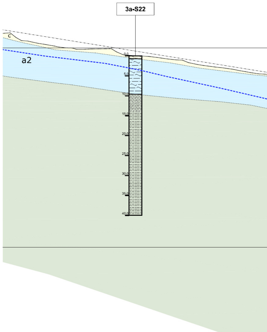
Figura 6-1 – Stralcio del profilo geotecnico.
