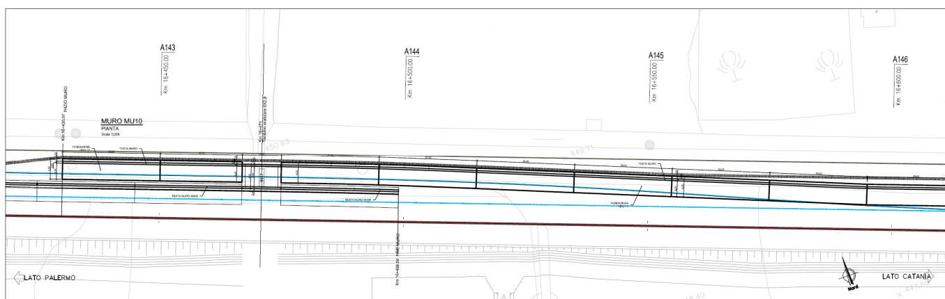
Figura 1-1 – TR04: Muro di sostegno in sx MU10 - Pianta.
