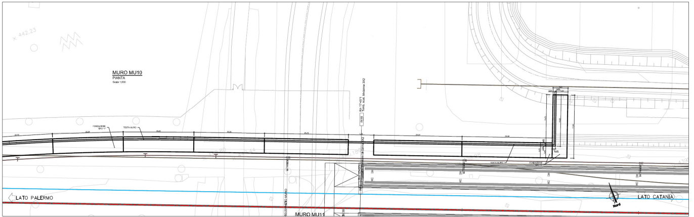
Figura 1-4 – TR04: Muro di sostegno in sx MU10 - Pianta.
