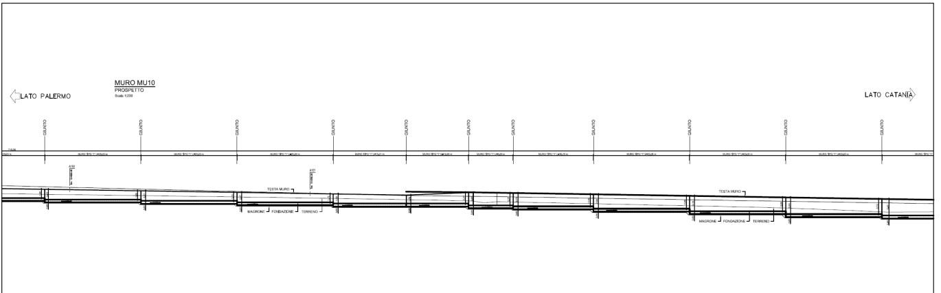
Figura 1-7 – TR04: Muro di sostegno in sx MU10 - Prospetto.
