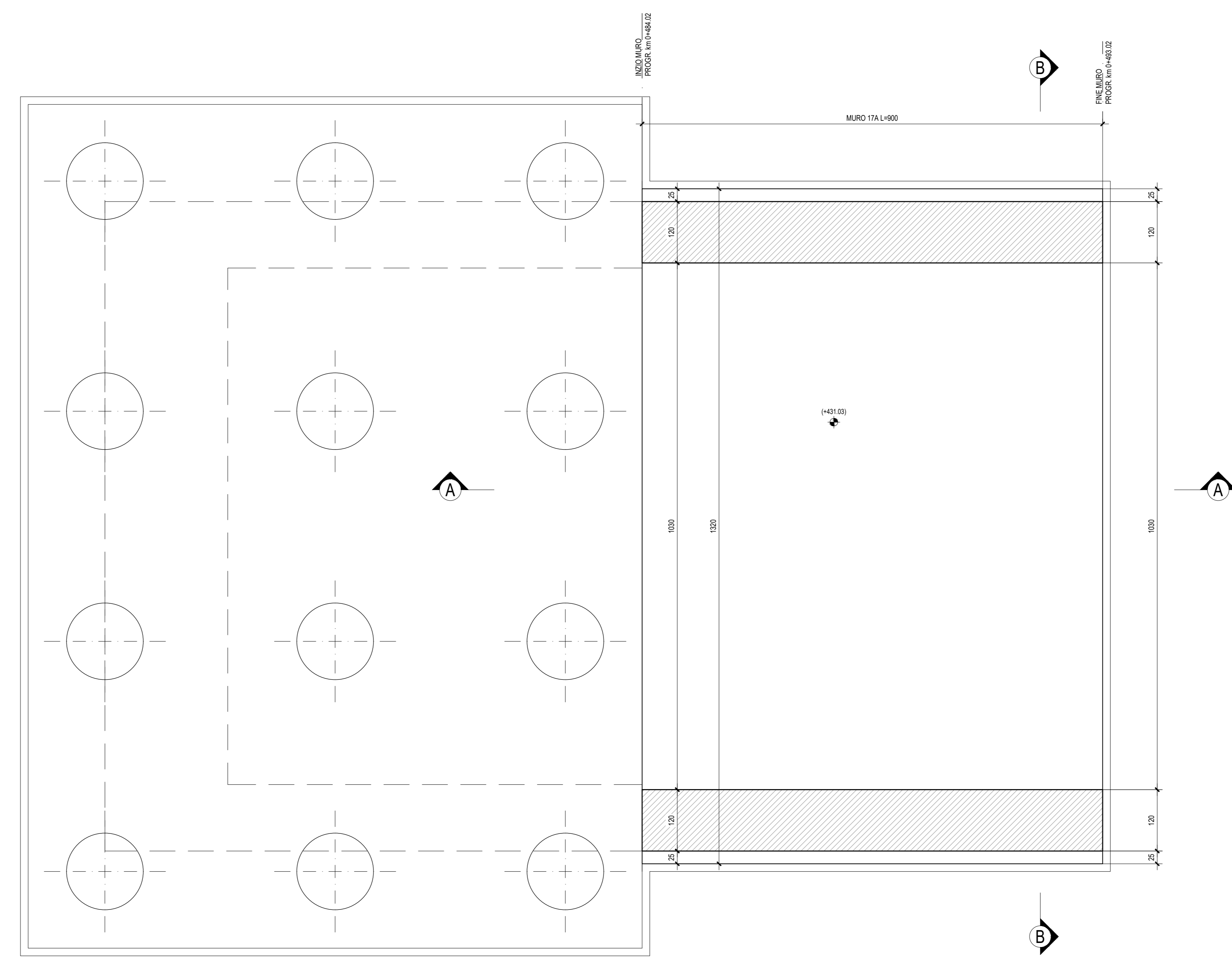
PIANTA SPICCATO - Scala 1:50
