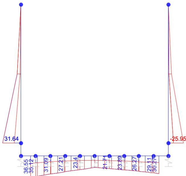
Momento Flettente
