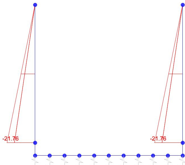
Sforzo normale
