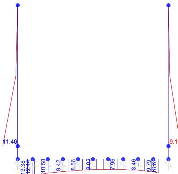
Momento flettente
