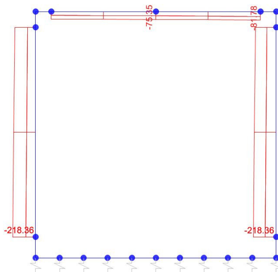
Sforzo normale
