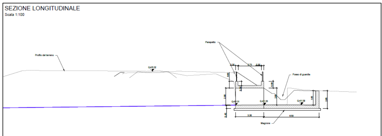
Figura 1b. Sezione longitudinale dello scatolare
