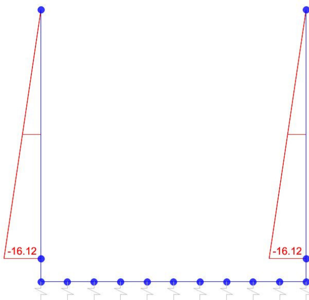
Sforzo normale
