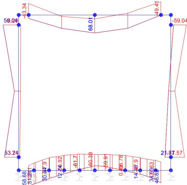
Momento Flettente
