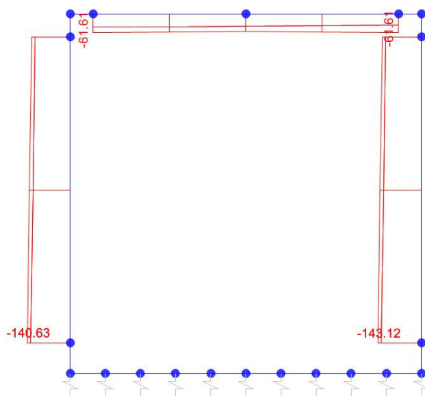
Sforzo normale
