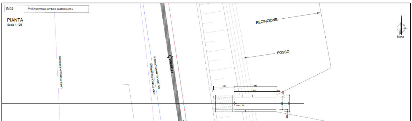
Figura 1a. Stralcio planimetrico dello scatolare
