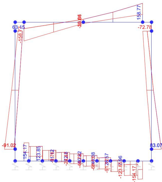
Taglio
