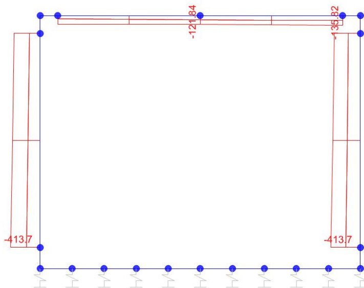
Sforzo normale
