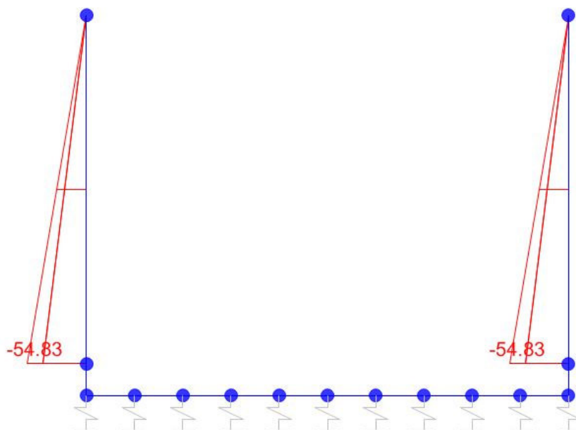
Sforzo normale
