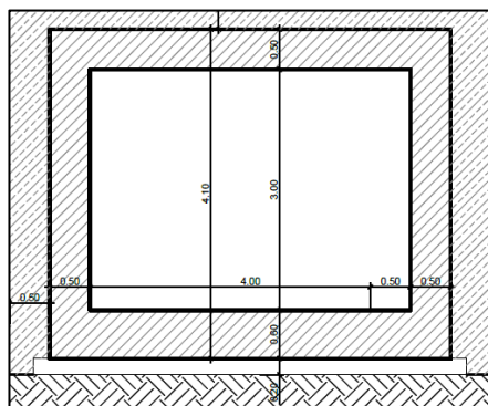
Figura 1c. Sezione trasversale dello scatolare
