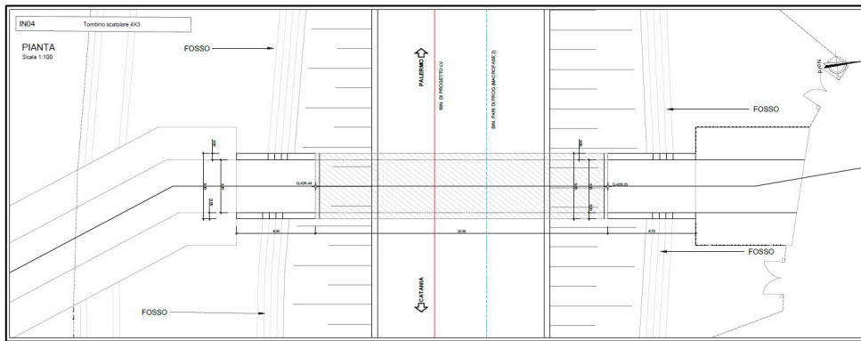
Figura 1a. Stralcio planimetrico dello scatolare
