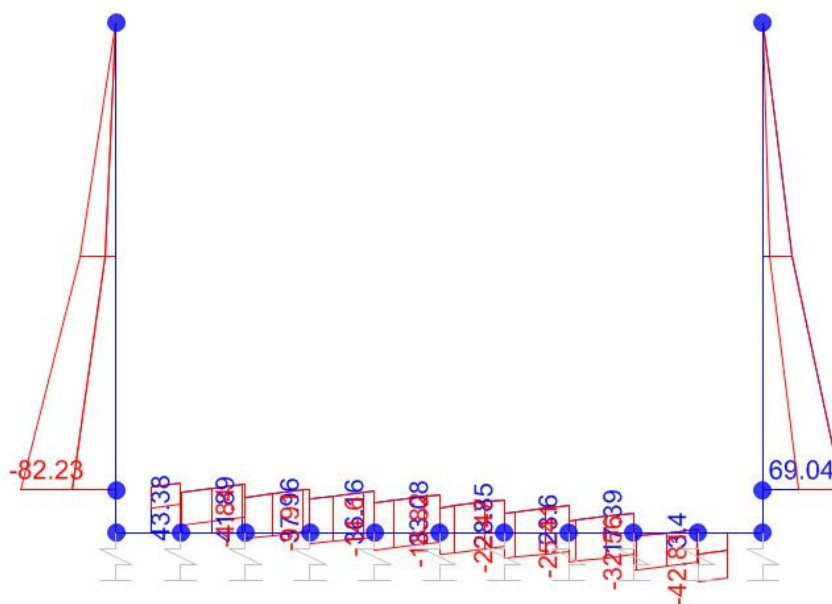
Taglio
