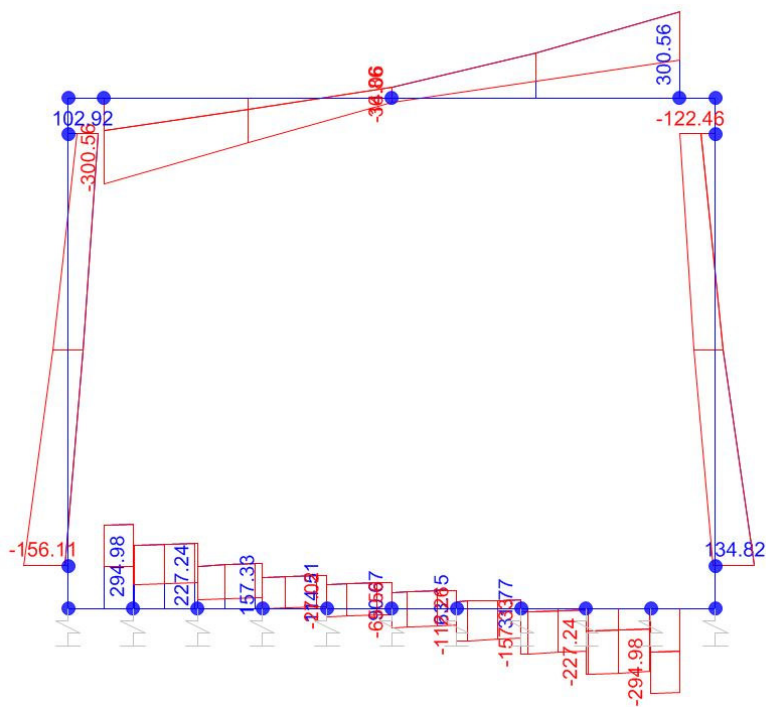
Taglio
