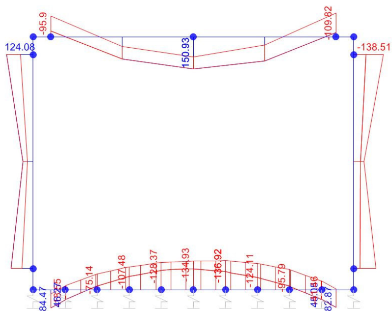
Momento Flettente
