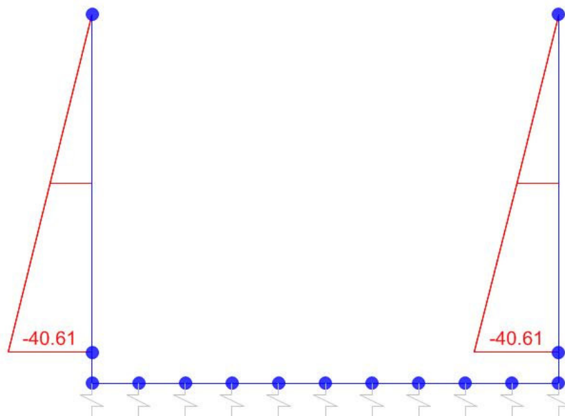
Sforzo normale
