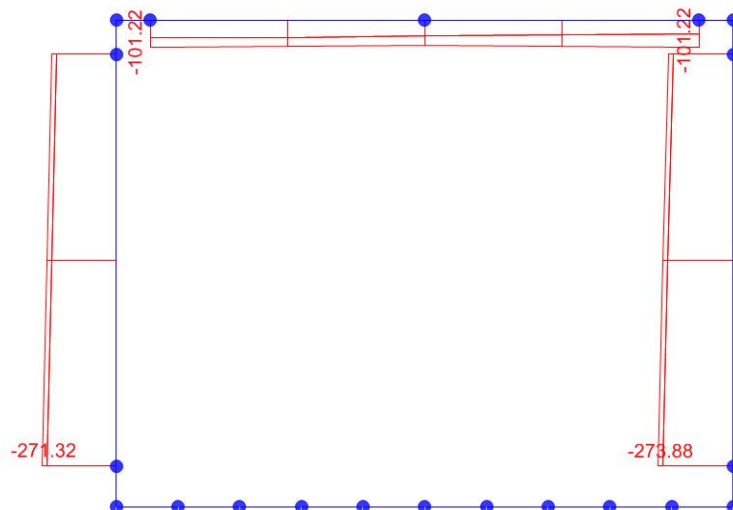
Sforzo normale
