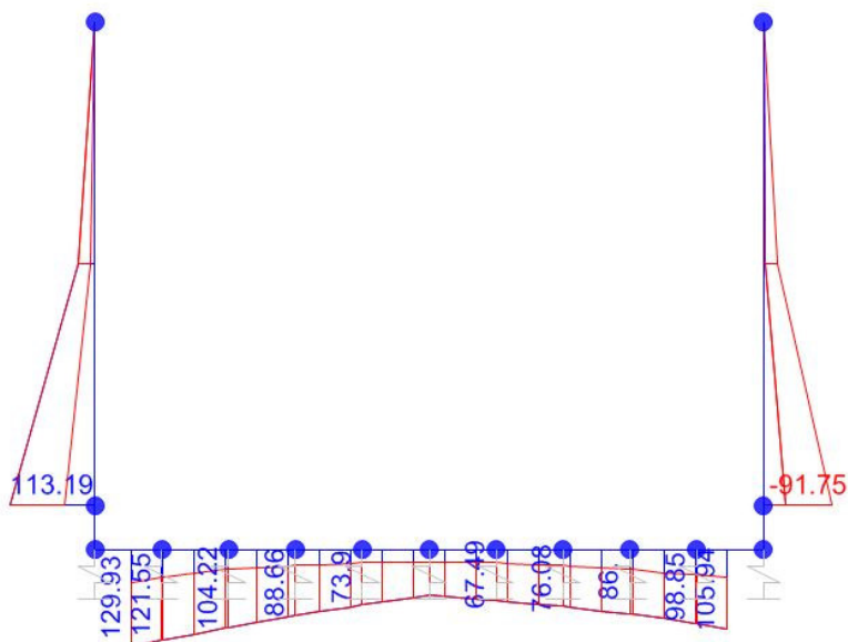
Momento Flettente
