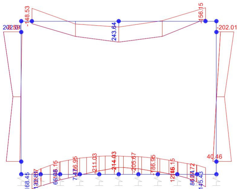
Momento Flettente
