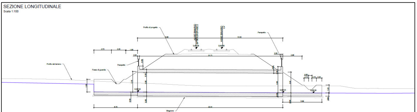
Figura 1b. Sezione longitudinale dello scatolare
