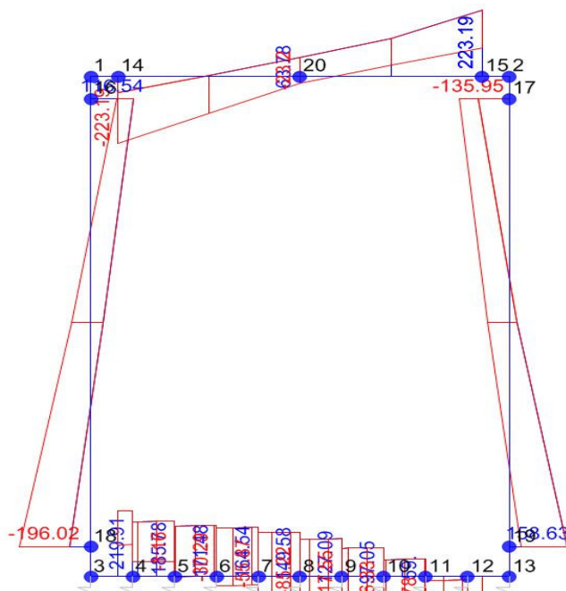
Taglio
