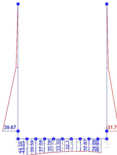
Taglio
