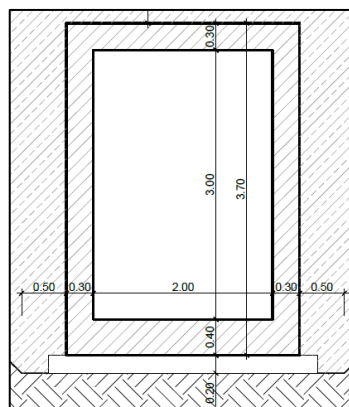
Figura 1c. Sezione trasversale dello scatolare
