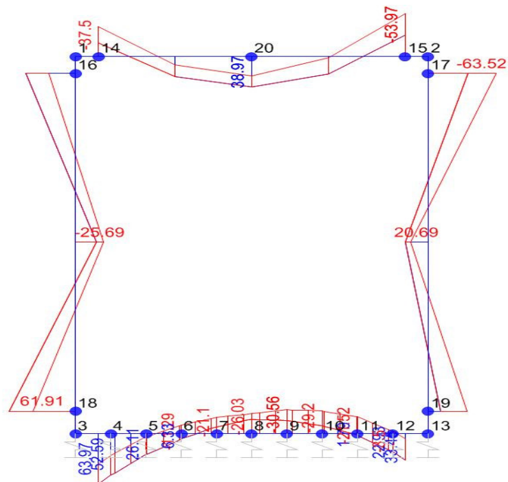
Momento Flettente
