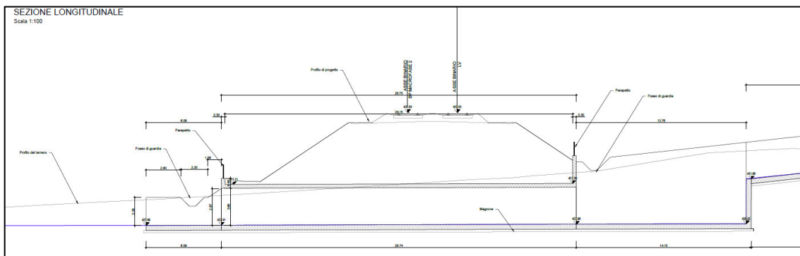
Figura 1b. Sezione longitudinale dello scatolare
