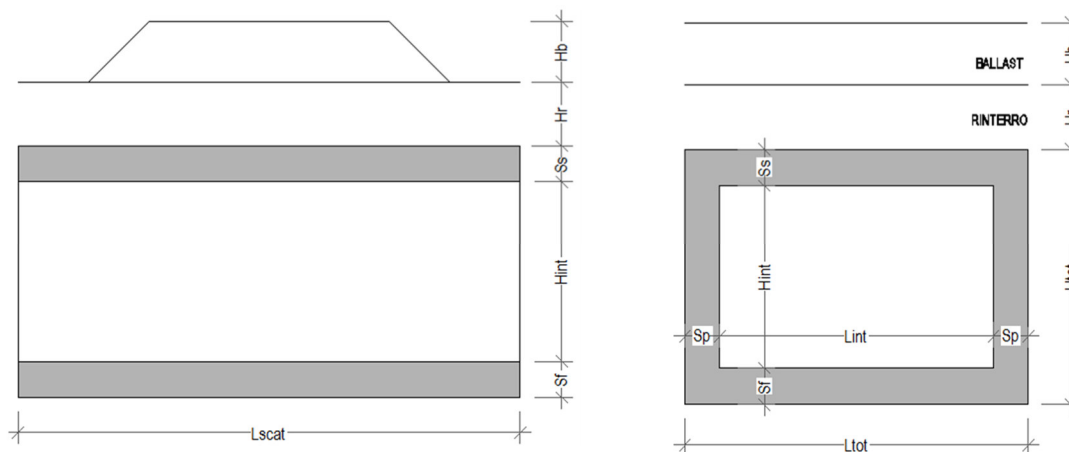
Figura 2. Simbologia adottata
