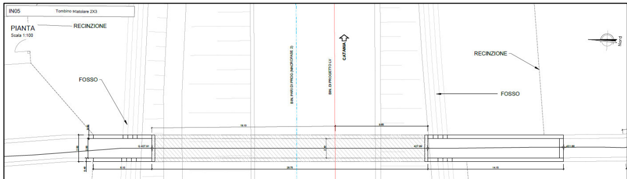
Figura 1a. Stralcio planimetrico dello scatolare
