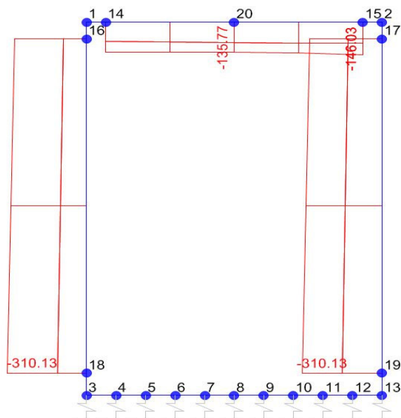
Sforzo normale
