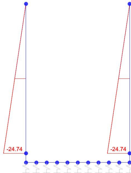
Sforzo normale
