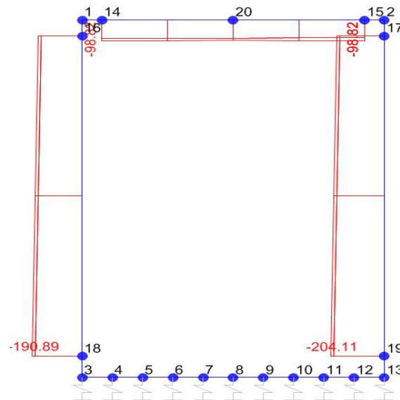
Sforzo normale
