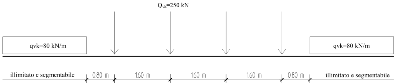
Figura 5. Treno LM71
