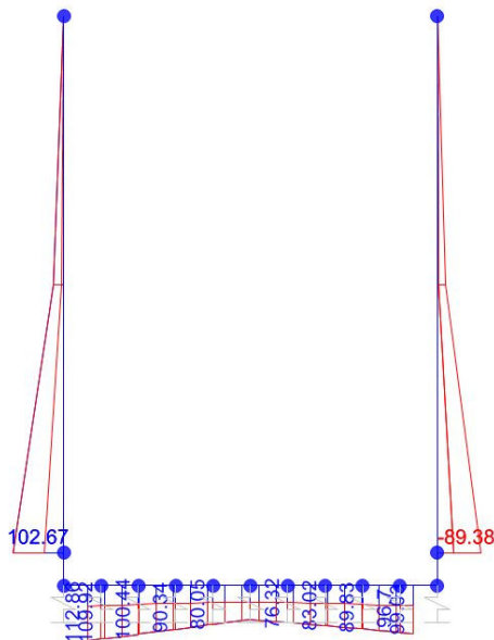
Momento Flettente
