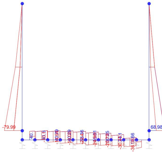
Taglio
