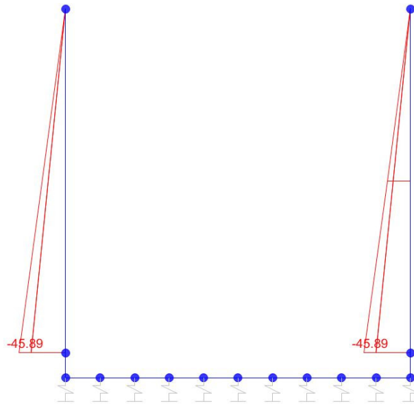
Sforzo normale
