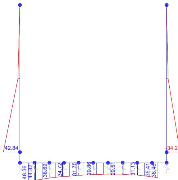
Momento
