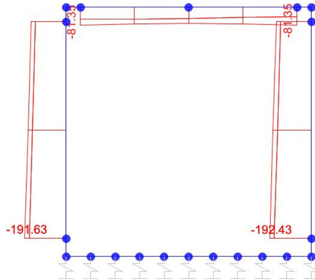
Sforzo normale
