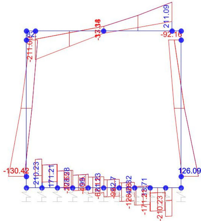
Taglio
