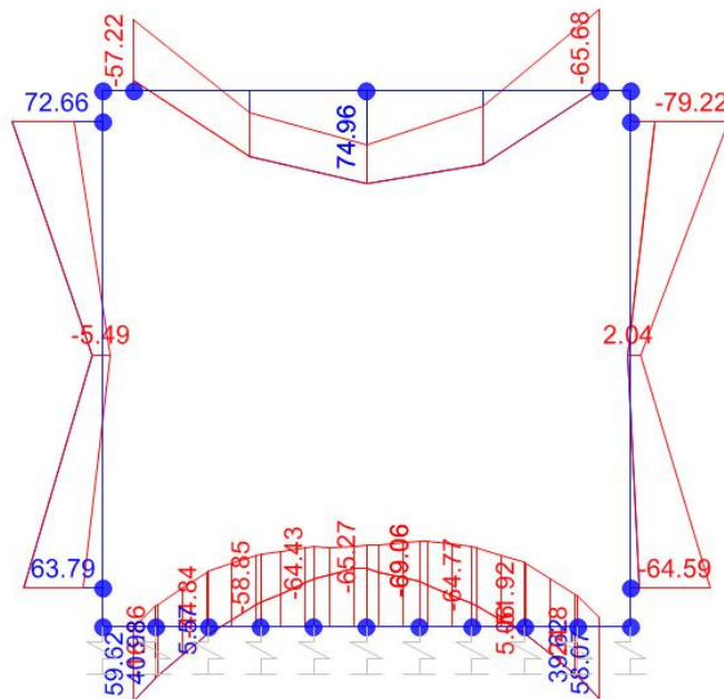
Momento Flettente
