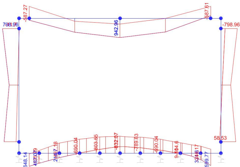
Momento Flettente
