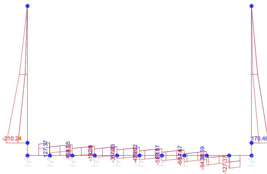
Taglio
