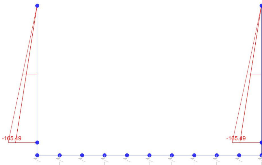
Sforzo normale
