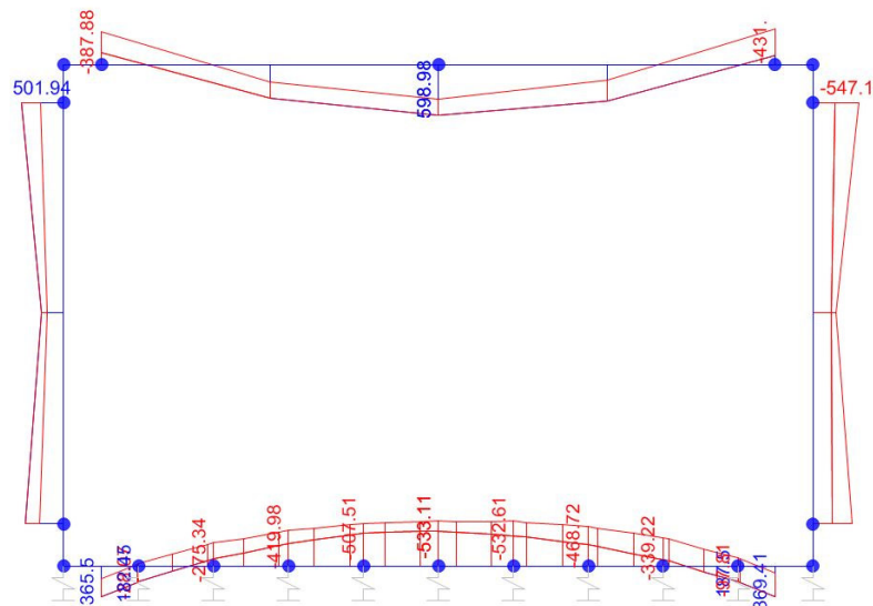
Momento Flettente
