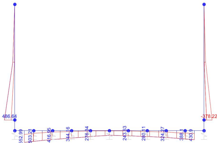
Momento Flettente
