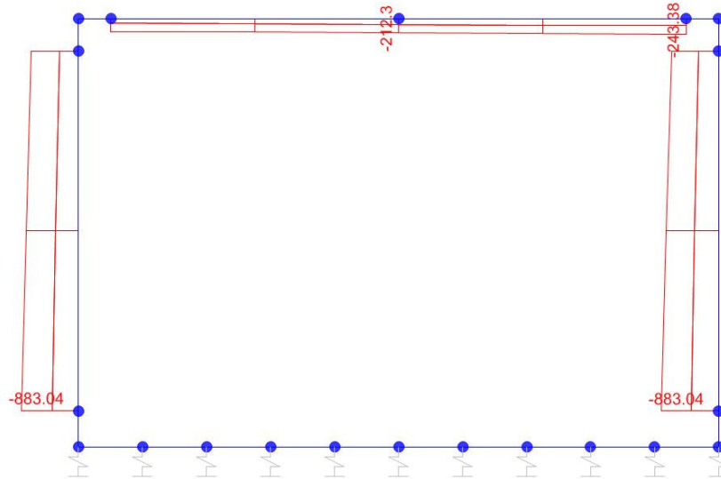
Sforzo normale
