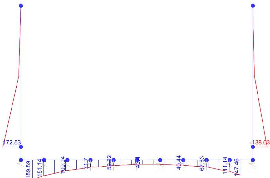
Momento
