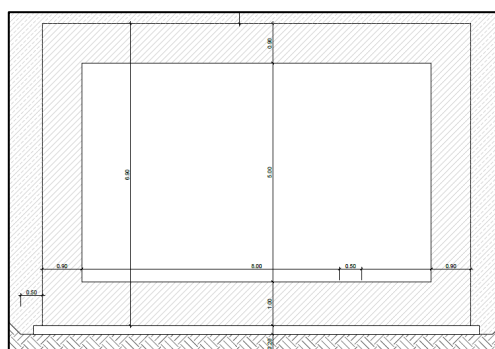
Figura 1c. Sezione trasversale dello scatolare
