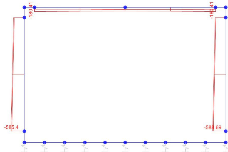
Sforzo normale
