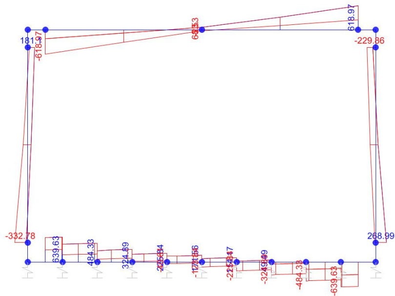
Taglio
