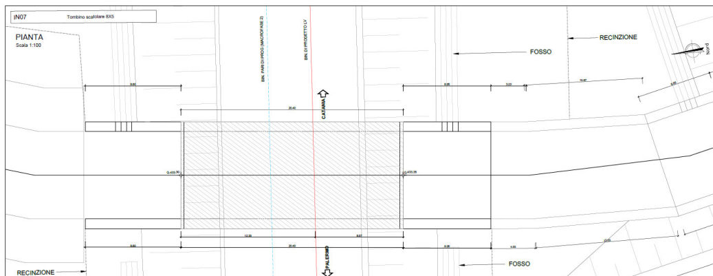
Figura 1a. Stralcio planimetrico dello scatolare
