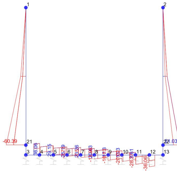
Taglio
