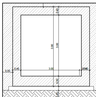
Figura 1c. Sezione trasversale dello scatolare
