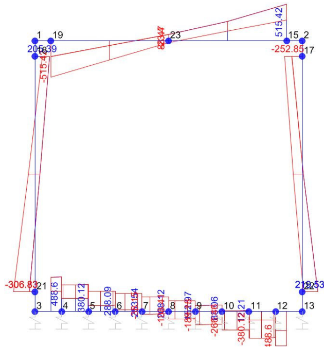
Taglio
