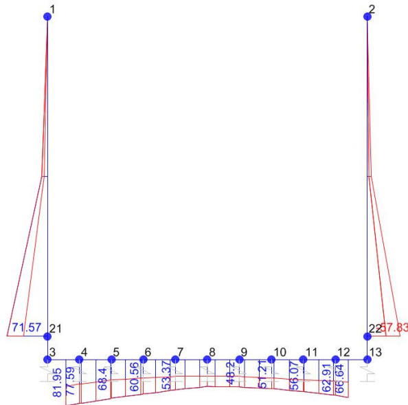
Momento Flettente
