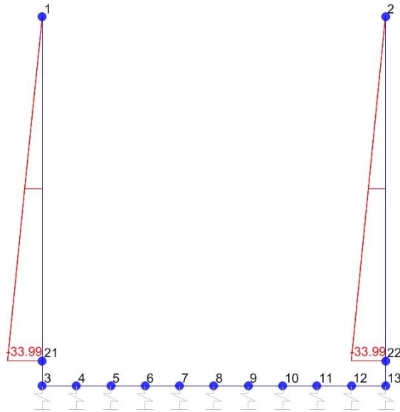
Sforzo normale
