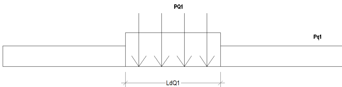
Figura 8. Carichi Treno LM71 su L_{dQ1}
