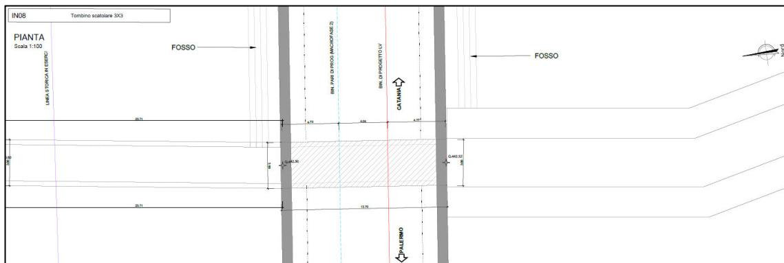
Figura 1a. Stralcio planimetrico dello scatolare
