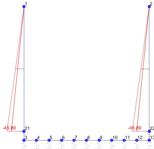
Sforzo normale
