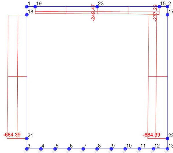
Sforzo normale
