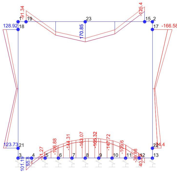
Momento Flettente
