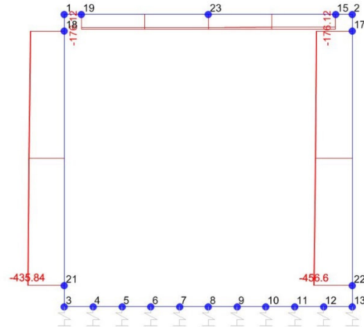
Sforzo normale
