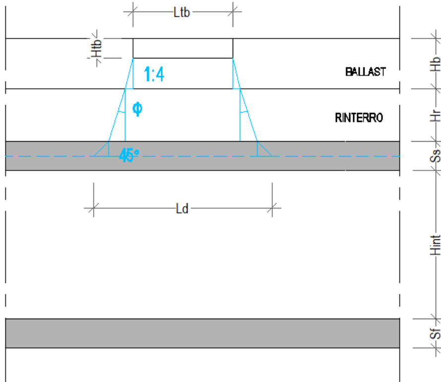
Figura 7. Schema modalità di diffusione dei carichi ferroviari
