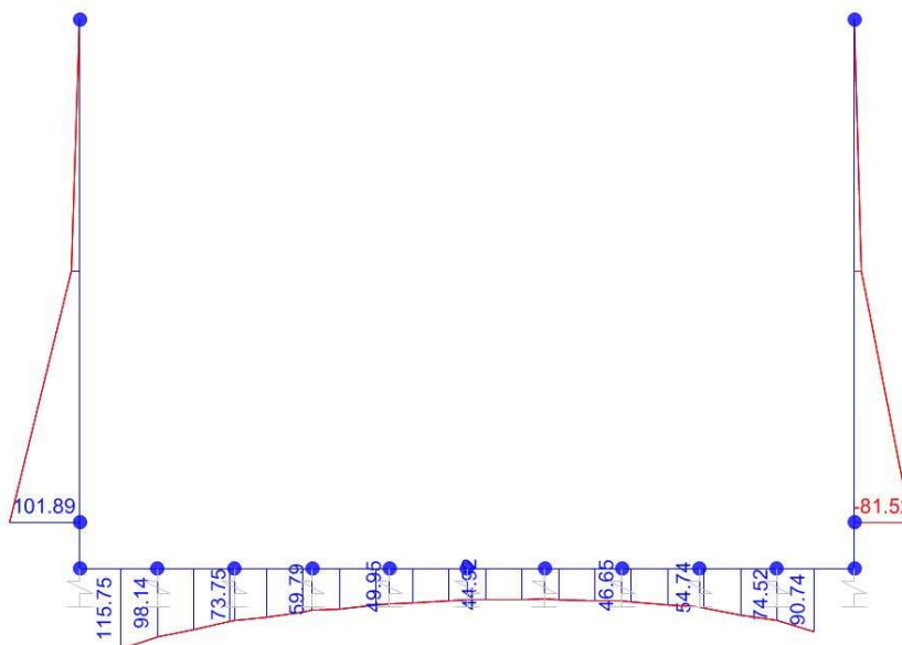
Momento flettente
