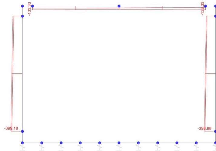
Sforzo normale
