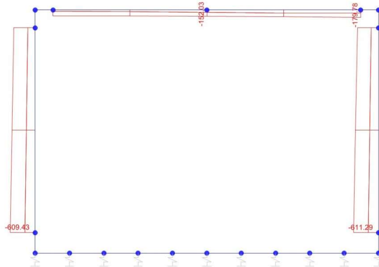
Sforzo normale
