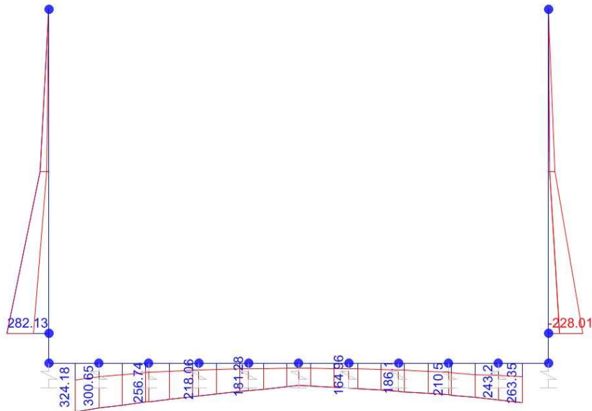
Momento Flettente
