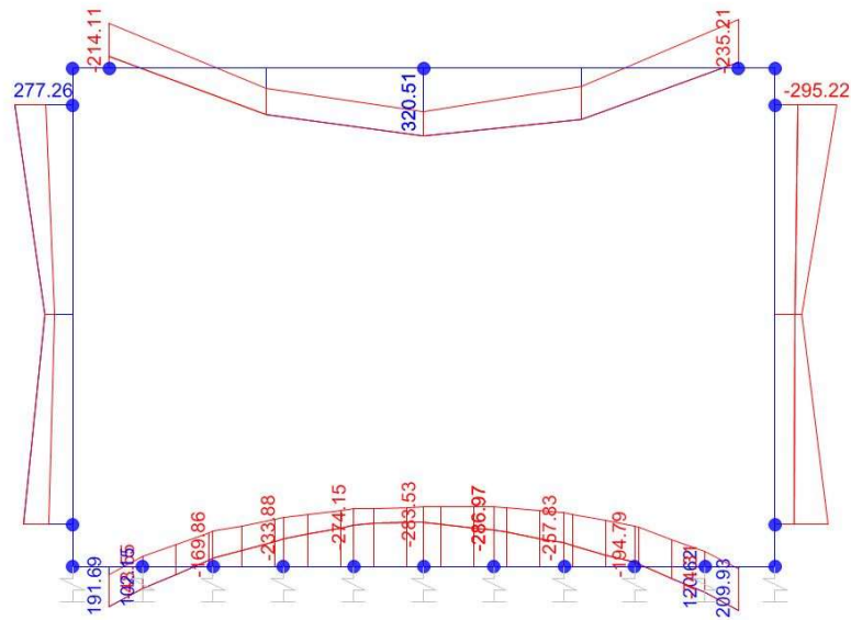
Momento Flettente
