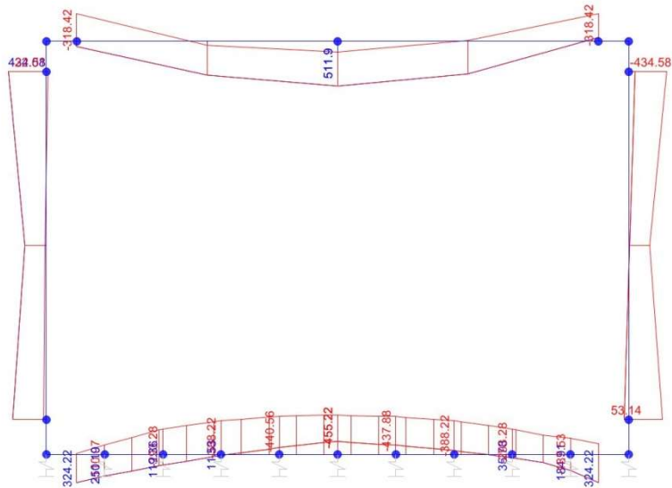
Momento Flettente
