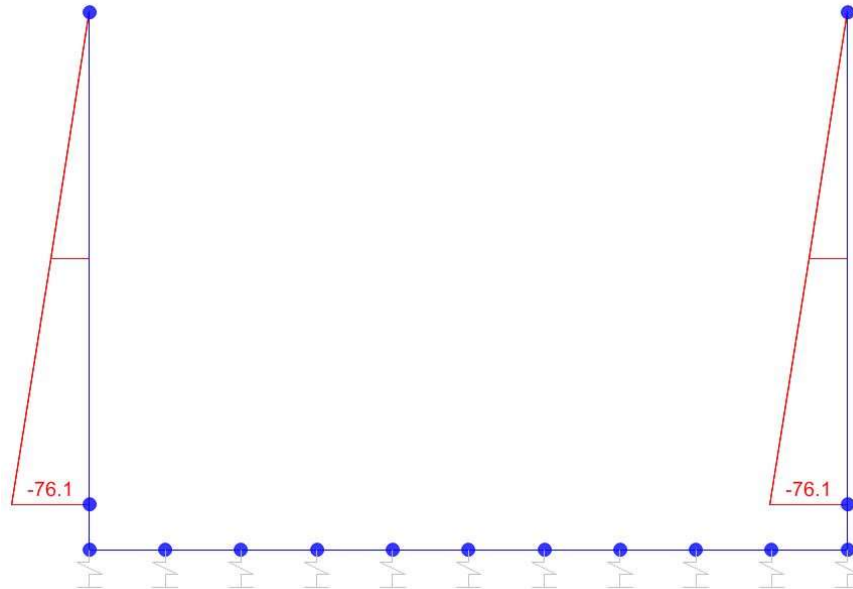
Sforzo normale
