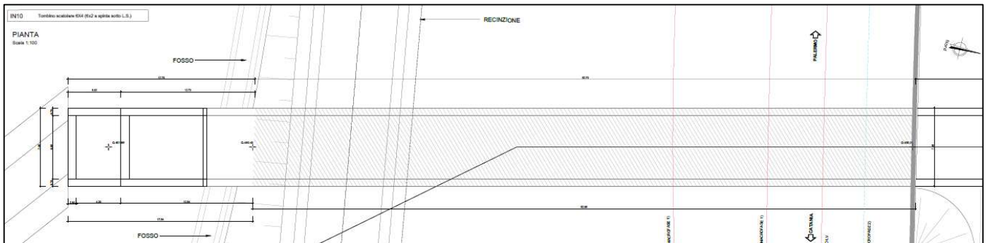
Figura 1a. Stralcio planimetrico dello scatolare
