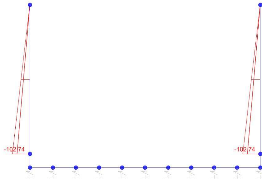
Sforzo normale
