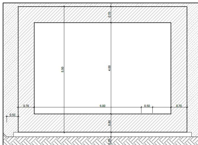
Figura 1c. Sezione trasversale dello scatolare
