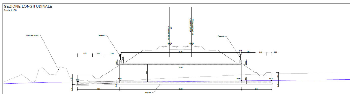
Figura 1b. Sezione longitudinale dello scotolare
