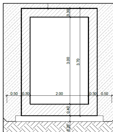
Figura 1c. Sezione trasversale dello scotolare
