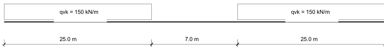
Figura 6. Treno SW/2
