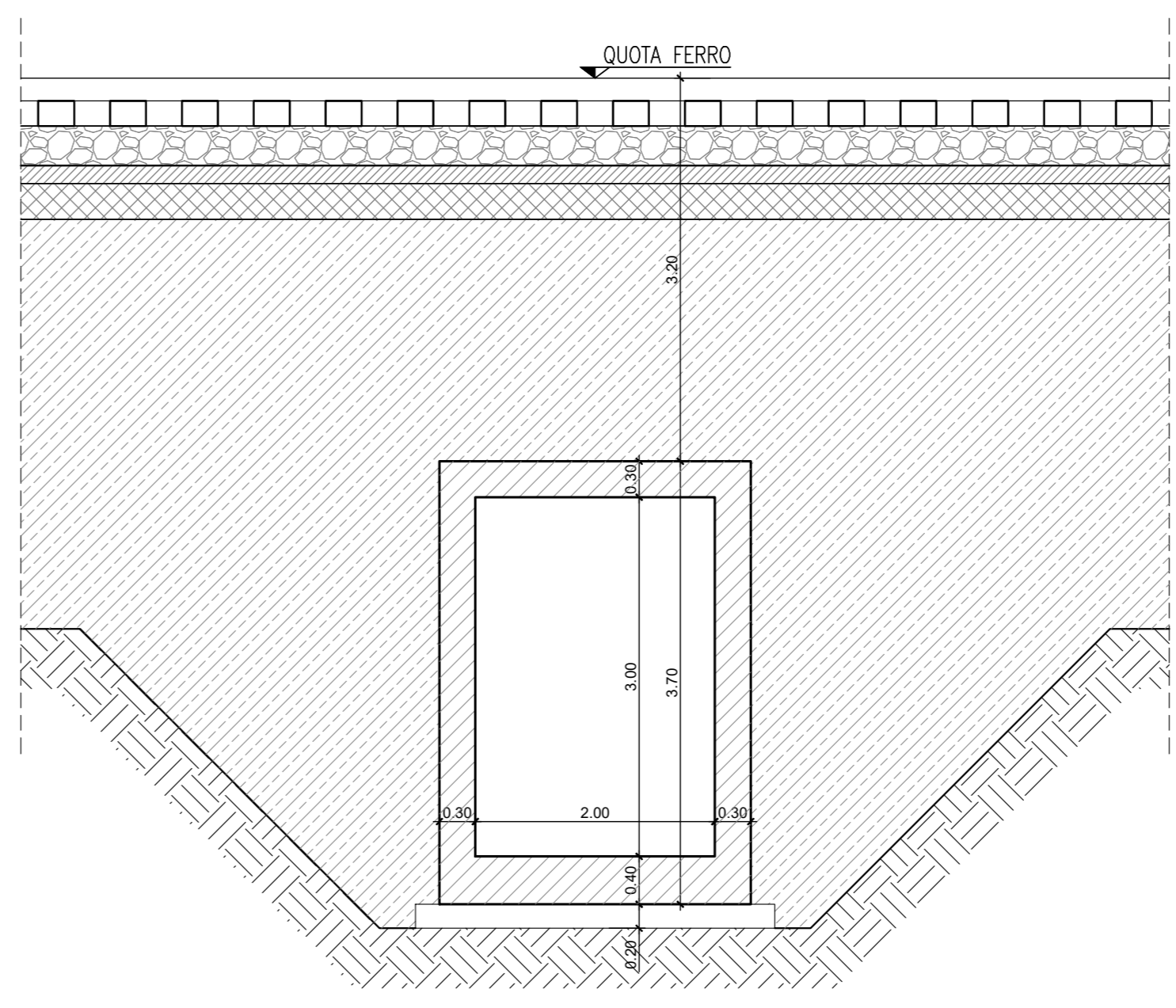
Tombino scatolare 2x3 sezione su BP MACROFASE 2 Scala 1:50
