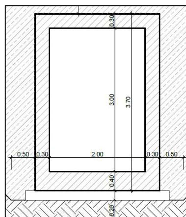
Figura 1c. Sezione trasversale dello scatolare
