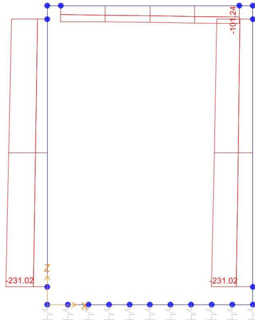
Sforzo normale
