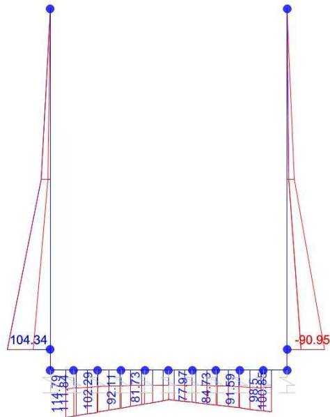
Momento Flettente
