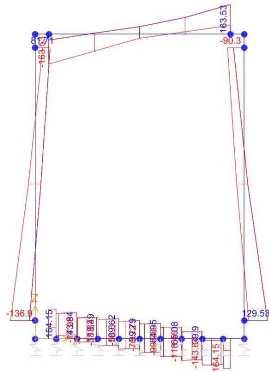
Taglio
