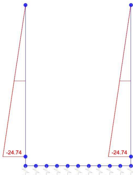
Sforzo normale
