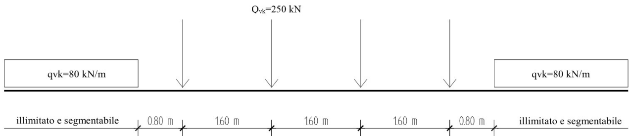
Figura 5. Treno LM71
