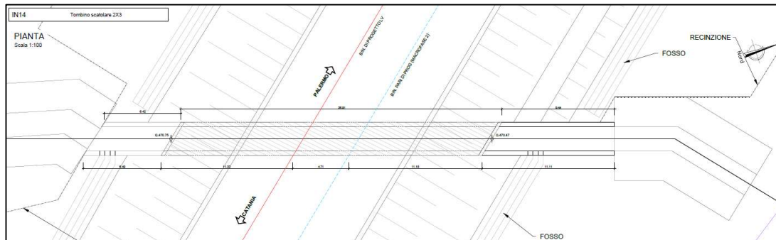
Figura 1a. Stralcio planimetrico dello scatolare
