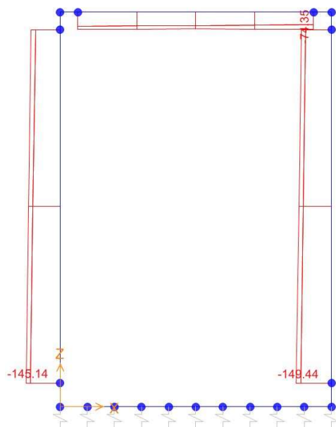
Sforzo normale
