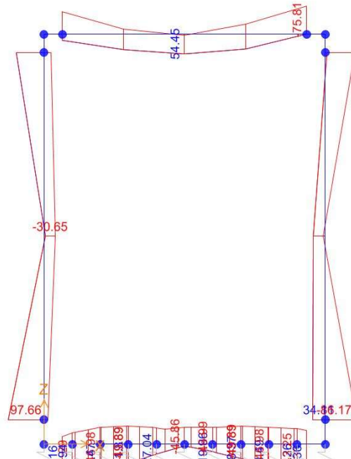
Momento Flettente
