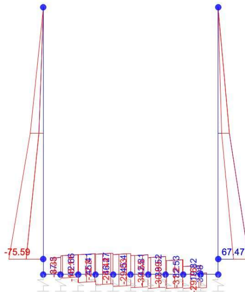
Taglio
