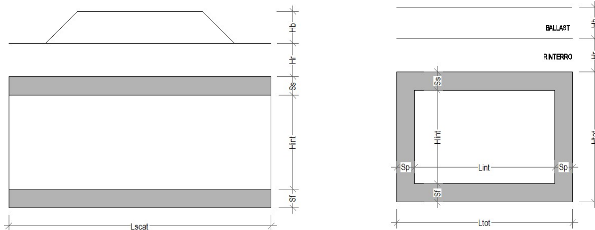
Figura 2. Simbologia adottata
