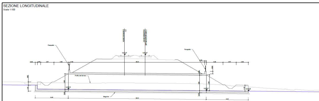
Figura 1b. Sezione longitudinale dello scatolare
