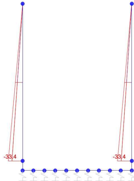
Sforzo normale
