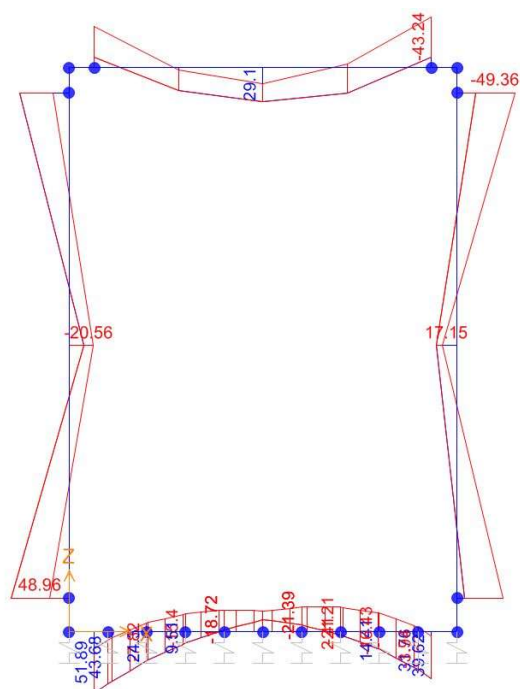
Momento Flettente
