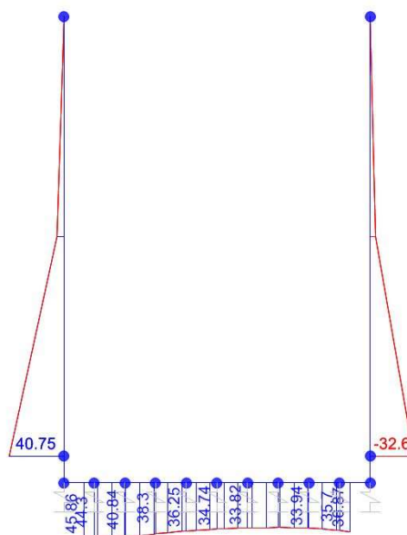
Momento flettente
